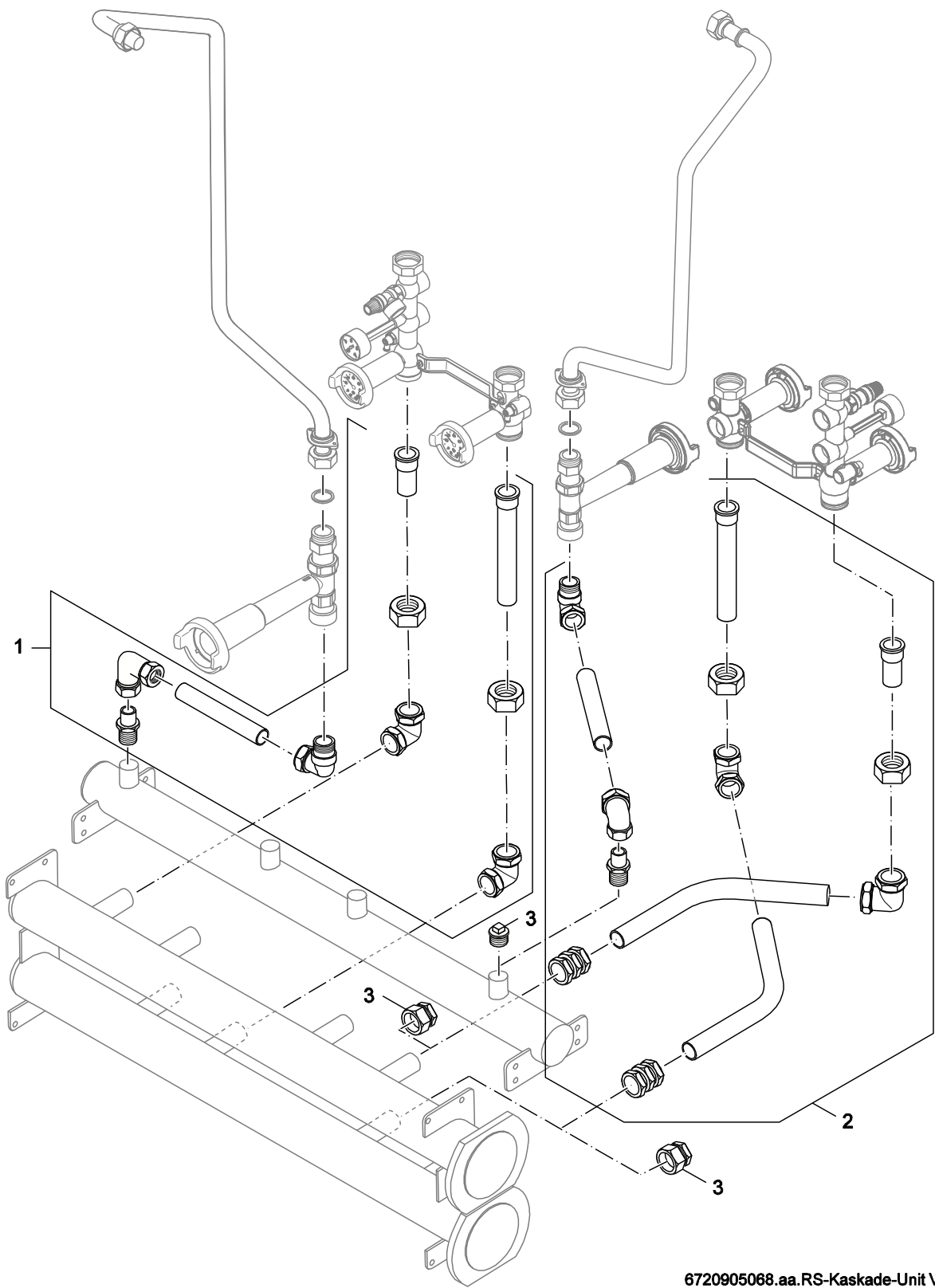
6720905068.aa.RS-Kaskade-Unit Verrohrung
