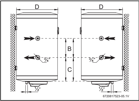
Фиг. 4 Размери в mm (Tronic 1500T)
