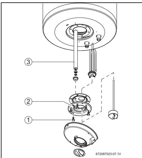
Фиг. 16 Достъп до вътрешността и компоненти
