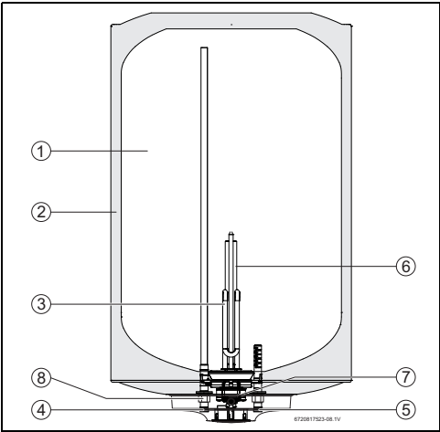
Фиг. 5 Конструкция на бойлера (пример Tronic 2000 T)
