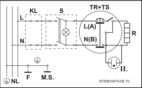
Фиг. 6 Схема на свързване
