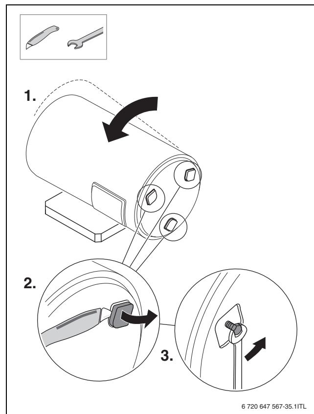
Fig. 9 Poser le ballon d'eau chaude sanitaire et dégager le pied réglable
