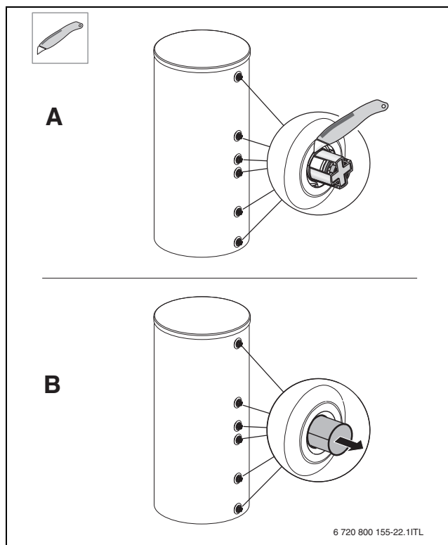
Fig. 11 Retirer les capuchons
