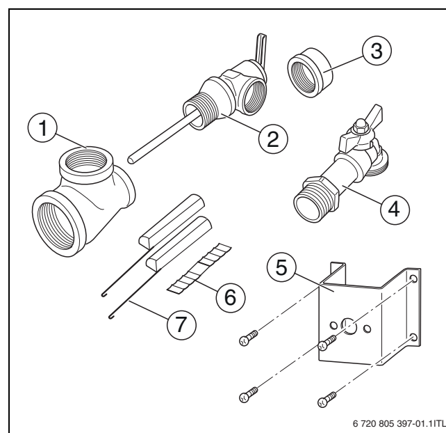
Fig. 1 Composants du kit du ballon
