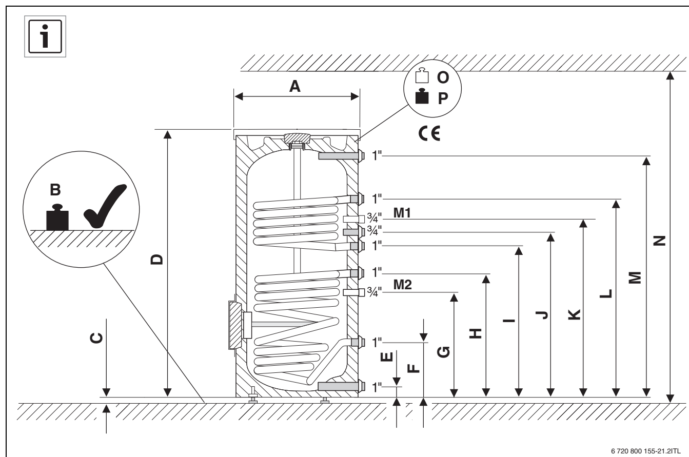
Fig. 5 Dimensions de construction et de raccordement
