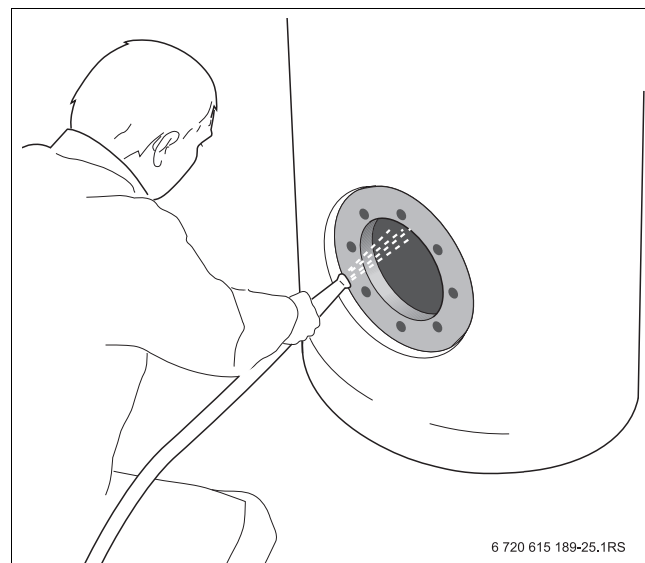
Fig. 20 Rincer le ballon d'ECS
