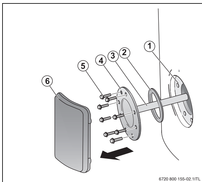
Fig. 23 Montage de la trappe de visite
