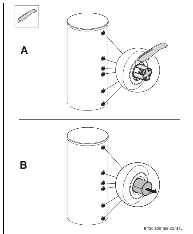
Fig. 11 Remove caps
