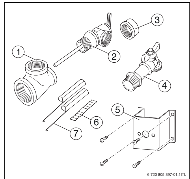
Fig. 1 Componentes del set del acumulador
