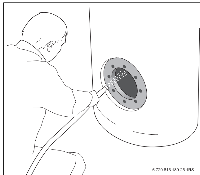
Fig. 20 Limpiar el acumulador de agua caliente
