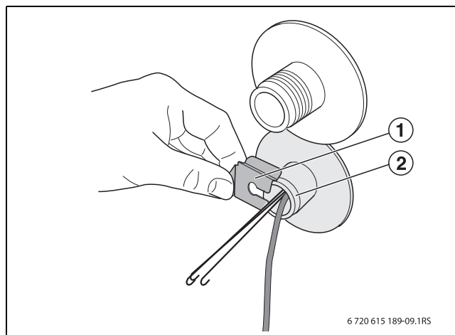
Fig. 15 Montage de l'arrêt de sécurité de la sonde
