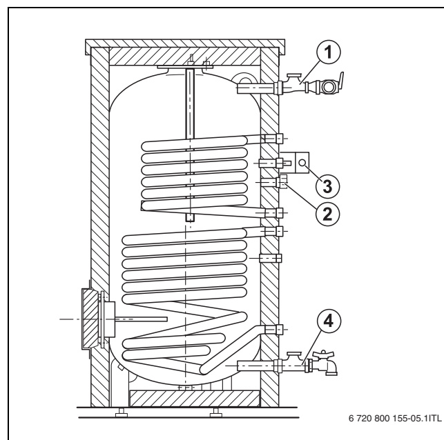
Fig. 13 Raccorder le kit au ballon d'eau chaude sanitaire
