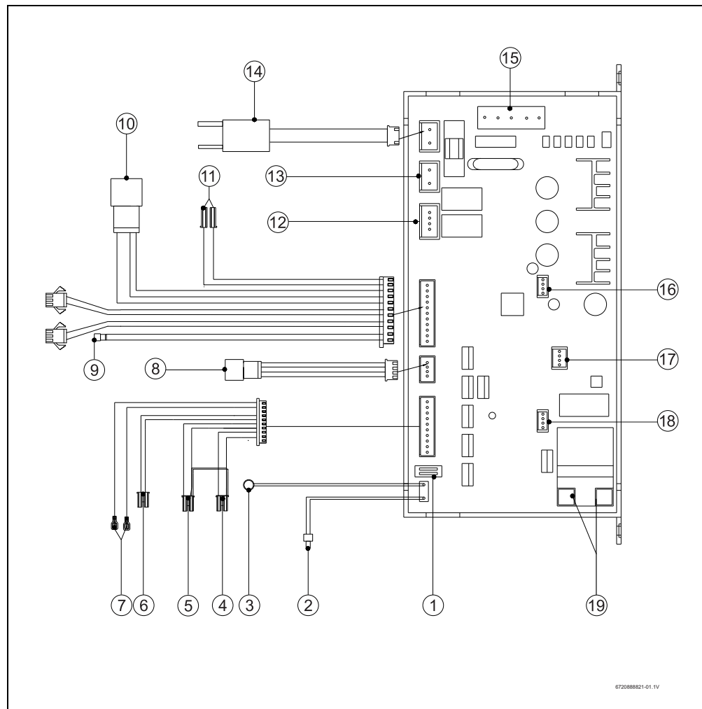
Fig. 20 Esquema de conexión
