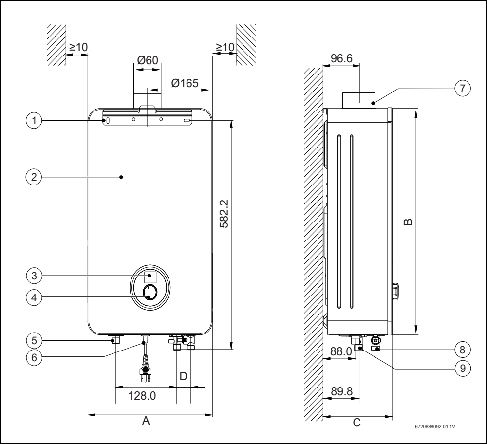
Fig. 1 Dimensiones 8/11... (en mm)
