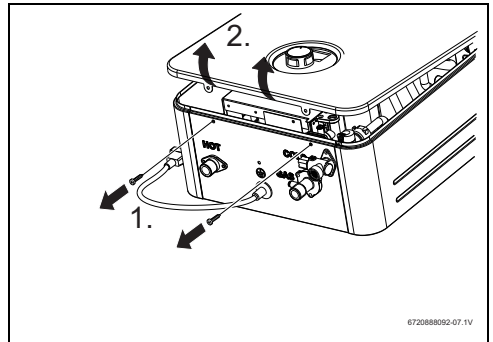
Fig. 18 Retirar la parte frontal
