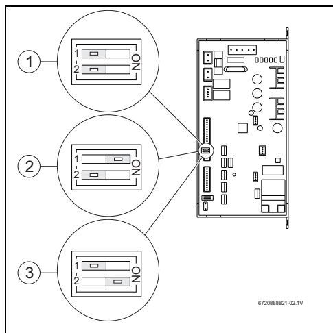
Fig. 14 Configuración de los interruptores
