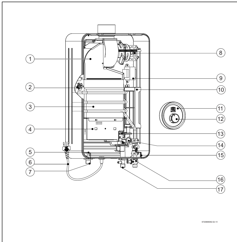
Fig. 3 Construcción del aparato
