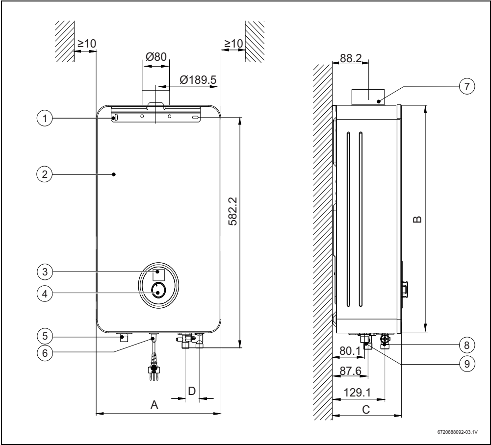
Fig. 2 Dimensiones 14...(en mm)
