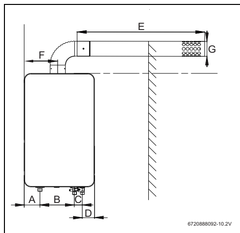
Fig. 10 Dimensiones... (en mm)
