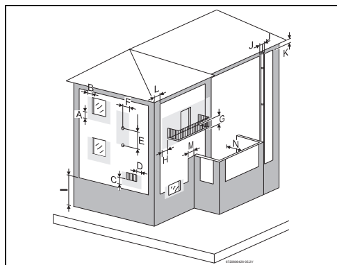
Fig. 12 Distancias mínimas a puntos de salida
