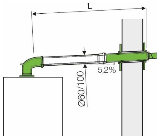
7 738 112 499 Sada odkouření 60/100 přes zeď s příp. kolénem
