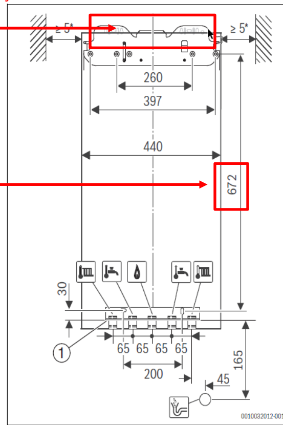
Obr. 3 Čelní pohled (mm)
