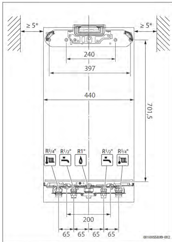
Obr. 17 Čelní pohled a připojky s použitím montážní lišty č. 869
