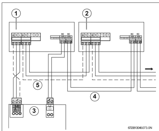
Obr. 28 Připojení několika modulů
