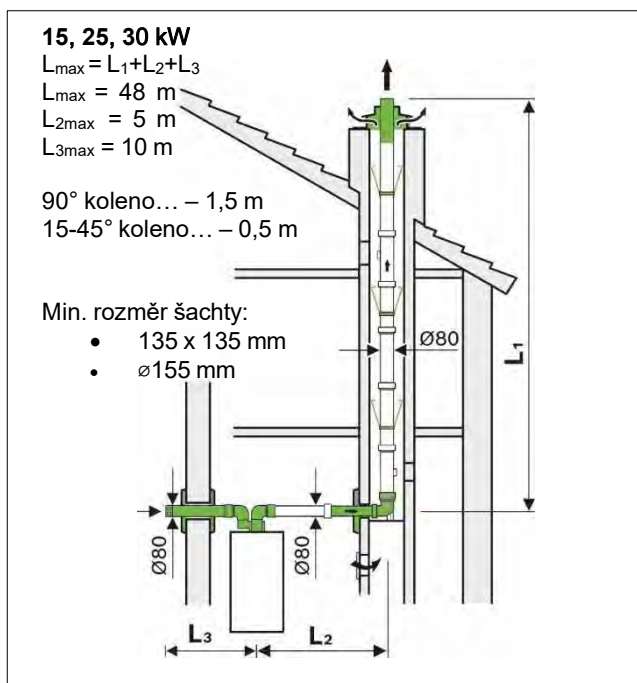
Obr. 36 Dělené odkouření C 53 2x80 mm
