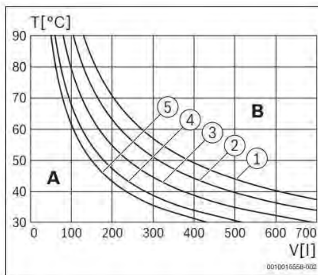
Obr. 20 Charakteristiky expanzní nádoby, expanzní nádoba vytápění o obsahu 12 l
