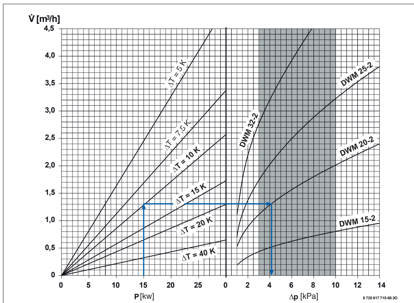
Obr. 30 Graf pro dimenzování třícestného směšovacího ventilu
