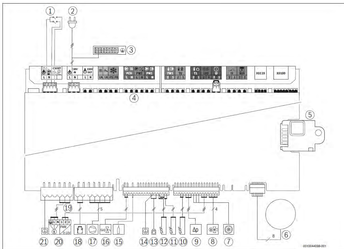
Obr. 23 Řídící deska – elektrické zapojení
