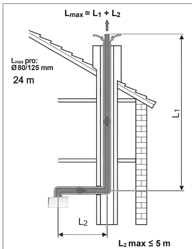
Obr. 37 Odvod spalin a přívod spalovacího vzduchu koncentrickým potrubím v šachtě podle C 93x
