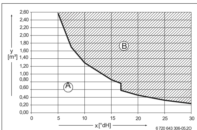
Obr. 23 Požadavky na plnicí a doplňovací otopnou vodu u přístrojů < 50 kW
