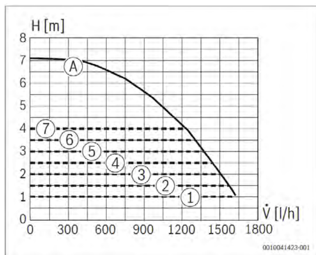
Obr. 21 Pole charakteristik čerpadla a charakteristiky čerpadla
