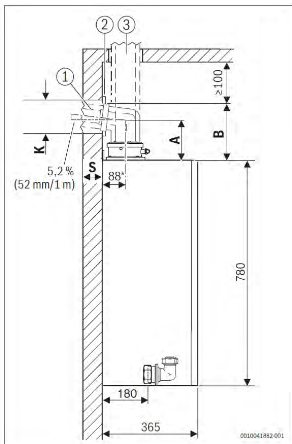
Obr. 19 Pohled z boku, při čelním pohledu je osa odkouření ve středu kotle
