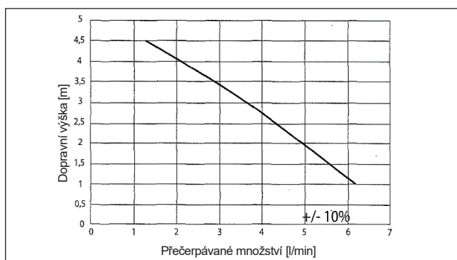
Obr. 25 Graf čerpadla kondenzátu
