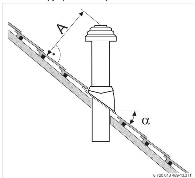
Obr. 34 Odstupy a sklony šikmých střech
