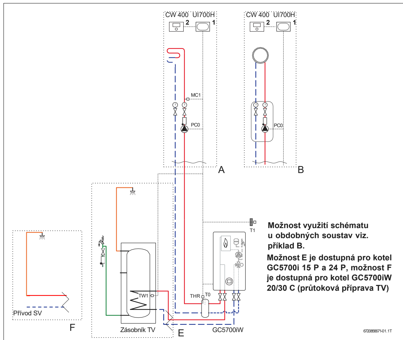
Obr. 4 Schéma soustavy s regulací (orientační zapojení)
