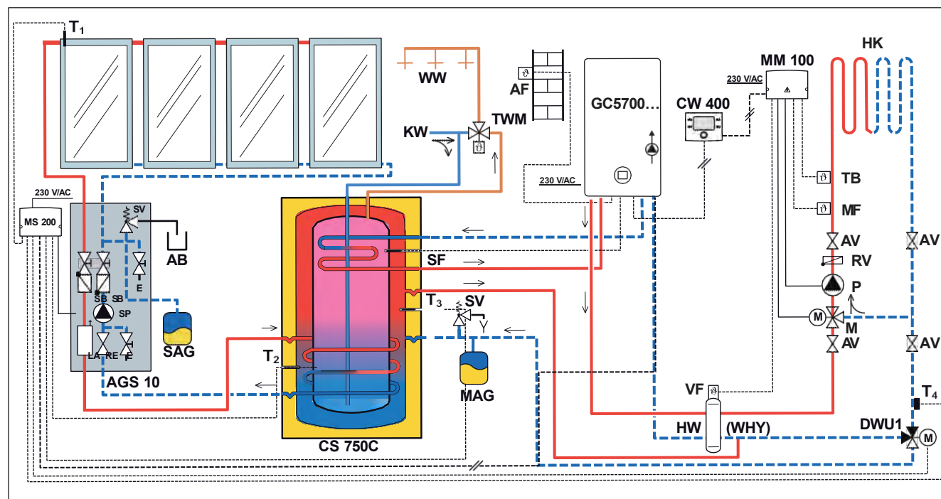
Obr. 9 Příklad solární podpory vytápění se směřovaným otopným okruhem
