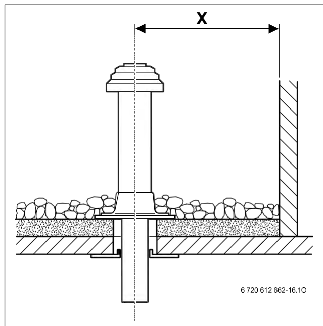
Obr. 33 Odstupy u ploché střechy
