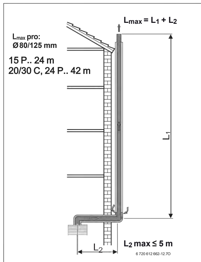
Obr. 40 Odvod spalin koncentrickým potrubím na fasádě podle C 53x
