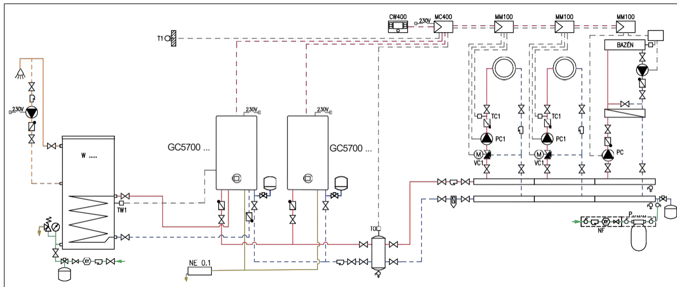
Obr. 15 Příklad kaskády se dvěma kondenzačními kotli, přípravou teplé vody a dvěma otopnými okruhy
