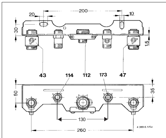
Obr. 18 Montážní připojovací lišta č. 869 pro montáž na omítku (standardně dodávána jako volitelné příslušenství ke kotlům Bosch Condens GC5700iW...)
