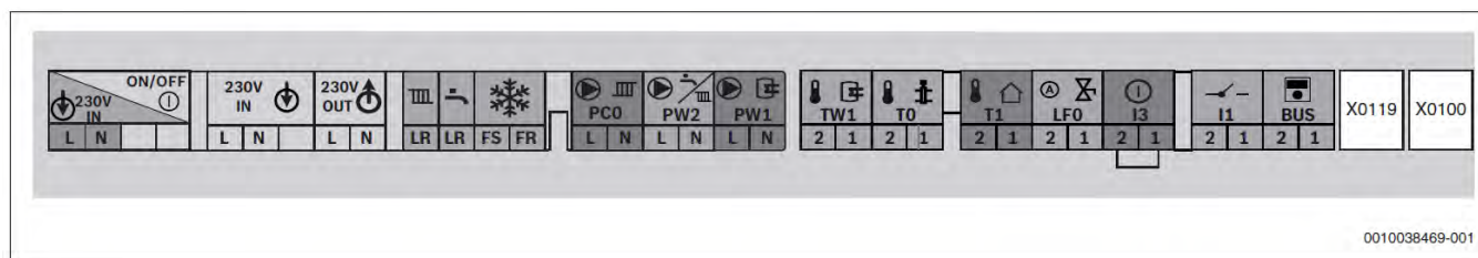
Obr. 22 Svorkovnice pro externí příslušenství
