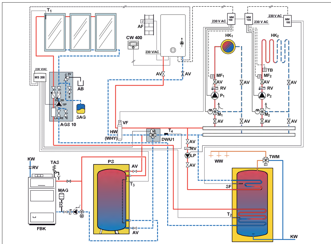
Obr. 10 Kotel na tuhá paliva se solární přípravou teplé vody a dvěma otopnými okruhy
