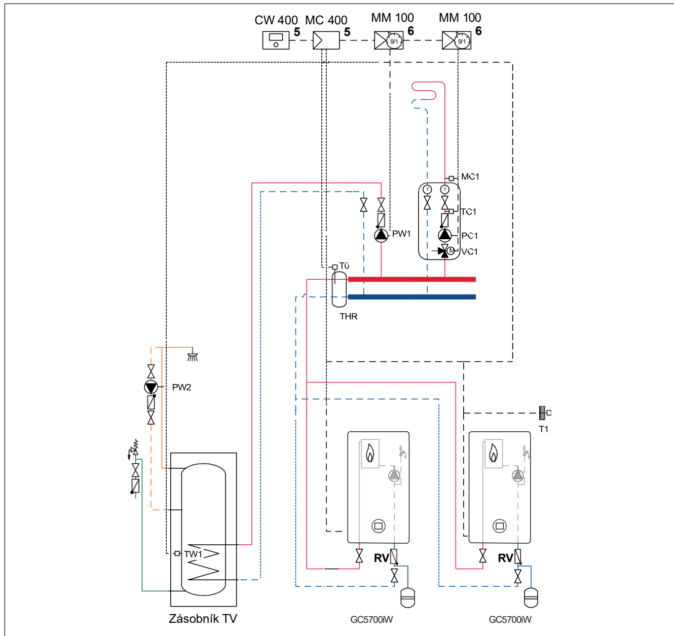
Obr. 13 Příklad kaskády se dvěma kondenzačními kotli, přípravou TV a jedním směšovaným otopným okruhem
