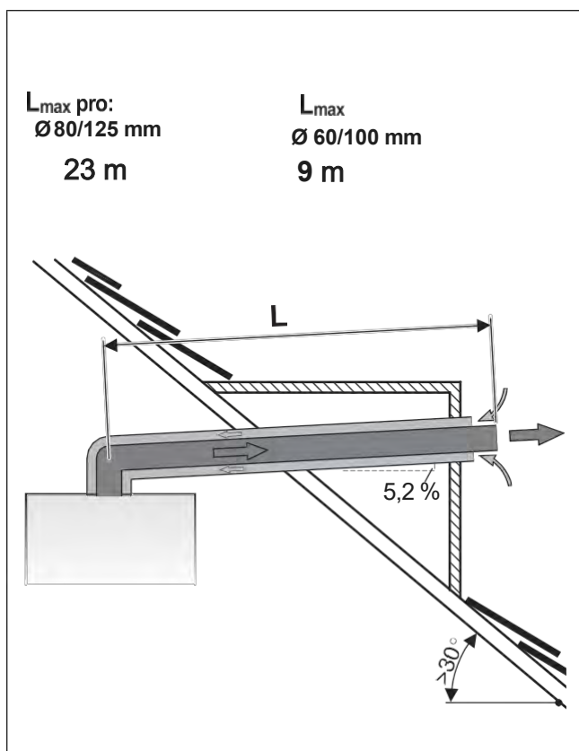
Obr. 38 Vodorovný odvod spalin a přívod spalovacího vzduchu koncentrickým potrubím podle C 13x
