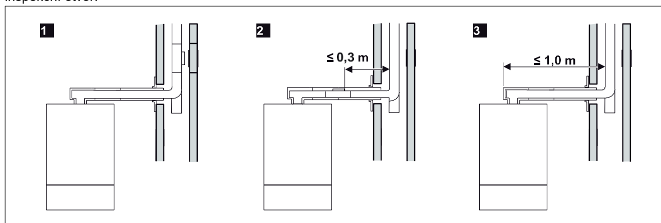
Obr. 31 Umístění revizních otvorů
