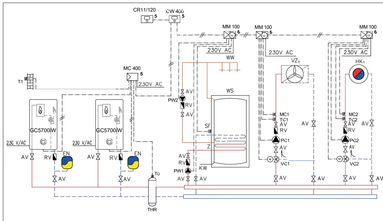
Obr. 14 Příklad kaskády se dvěma kondenzačními kotli, přípravou teplé vody a dvěma otopnými okruhy
