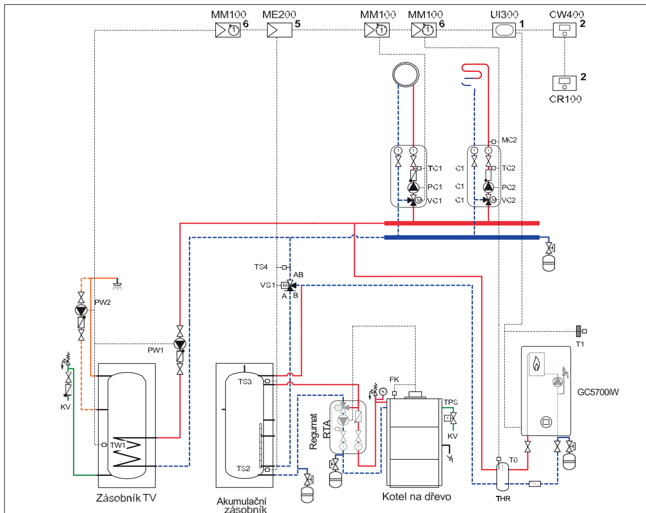
Obr. 11 Schéma soustavy s regulací (orientační zapojení)
