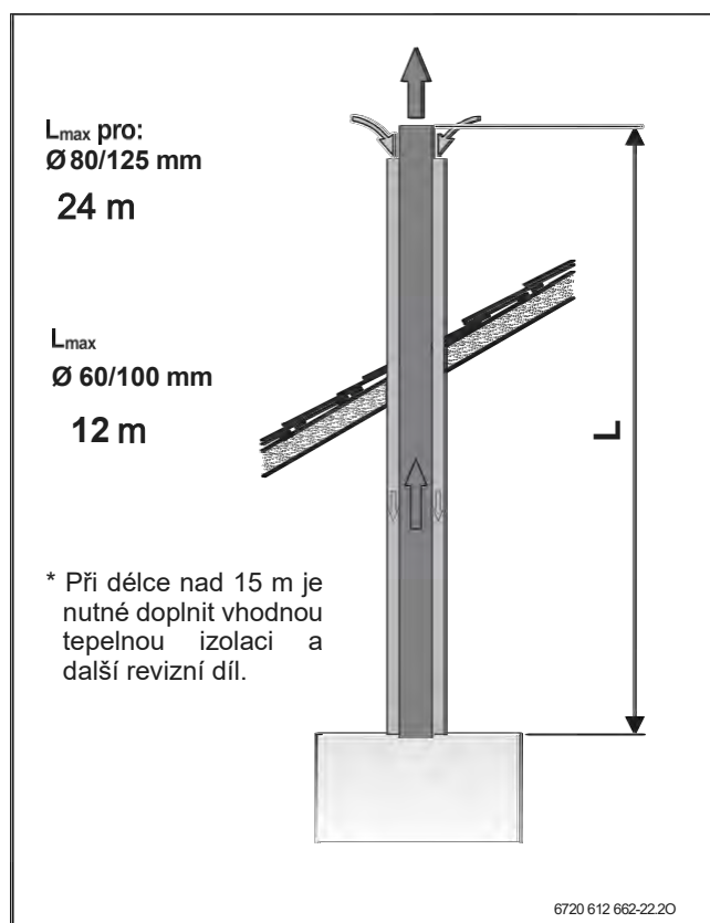
Obr. 39 Svislý odvod spalin a přívod spalovacího vzduchu koncentrickým potrubím podle C 33x
