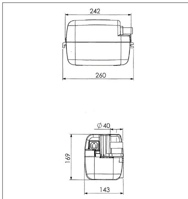
Obr. 24 Čerpadlo kondenzátu
