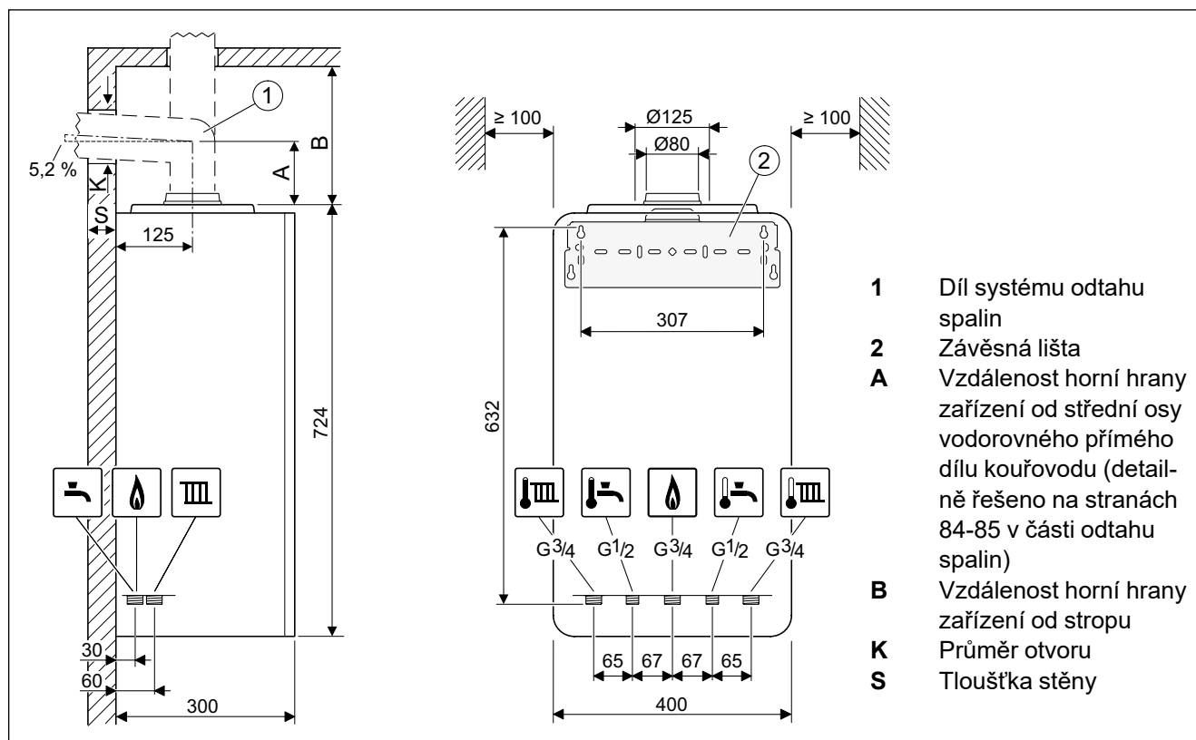
Obr. 25 Rozměry kotle Condens GC2300iW...
