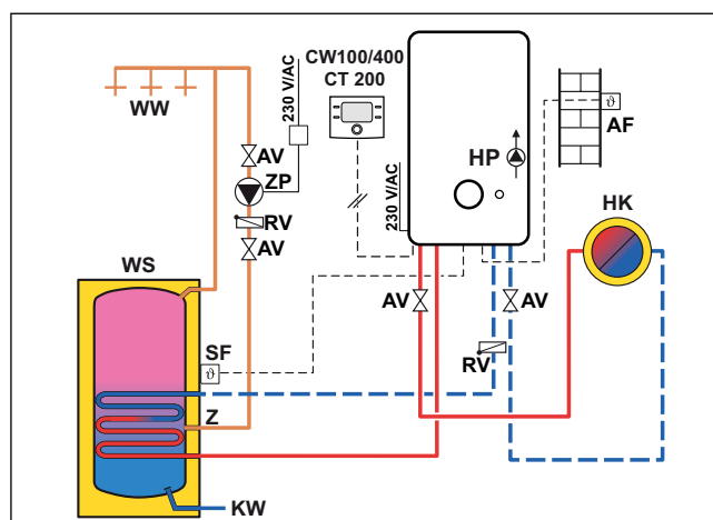
Obr. 11 Příklad s ekvitermním regulátorem CW100/CW400 a CT 200 a externě řízenou cirkulací teplé vody
