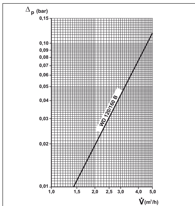
Obr. 49 WD 120/160 B
