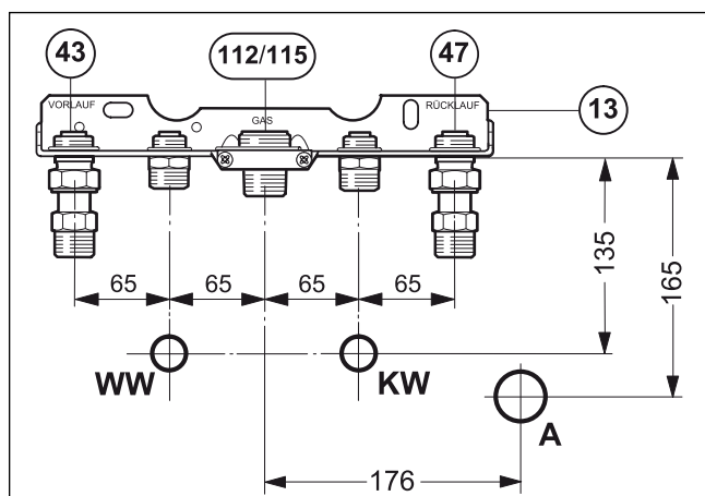
Obr. 44 Přípojky na omítku s odstupem od stěny 60 mm
