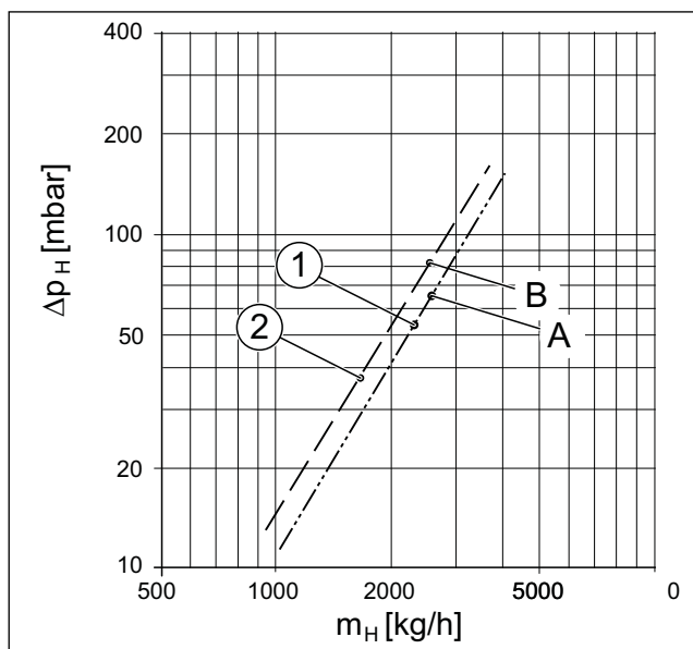
Obr. 56 Tlaková ztráta teplovodní otopné spirály zásobníku
