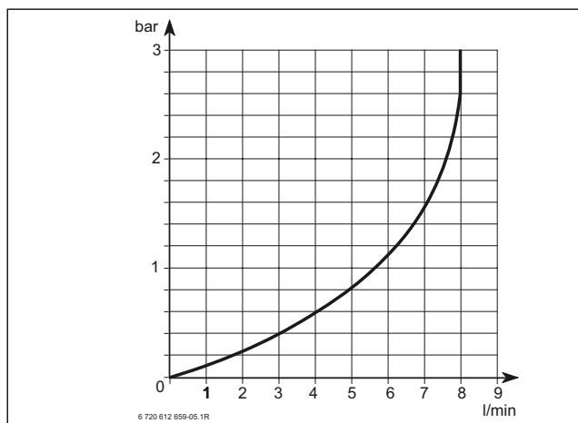
Obr. 60 Informativní graf tlakové ztráty u kombi-kotlů s montážními připojovacími lištami
