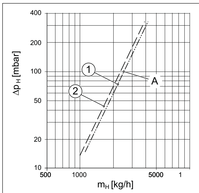
Obr. 57 Tlaková ztráta teplovodní otopné spirály zásobníku
