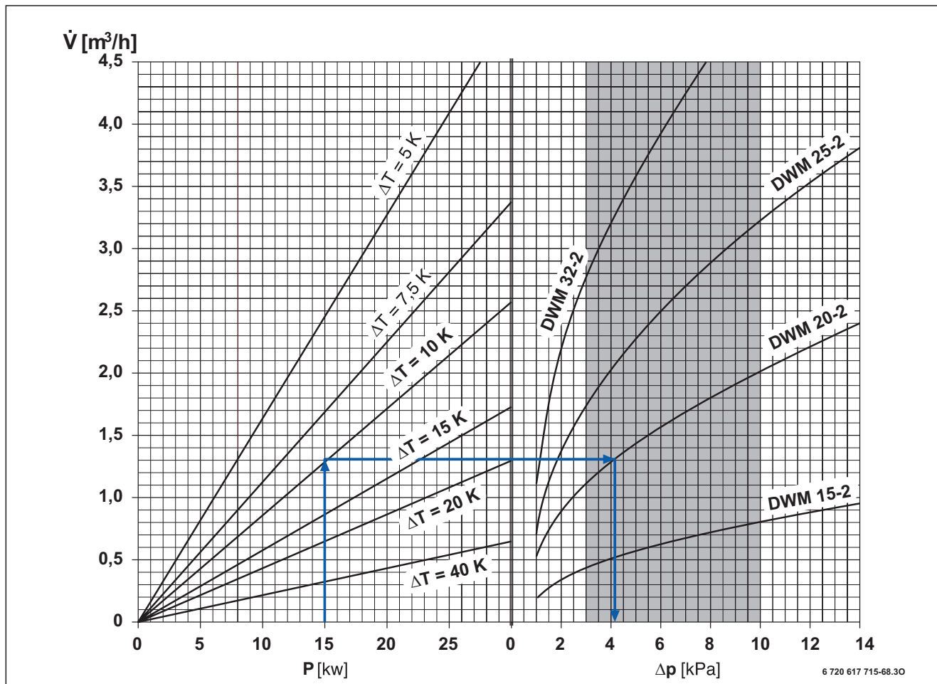
Obr. 72 Graf pro dimenzování 3cestného směšovacího ventilu
