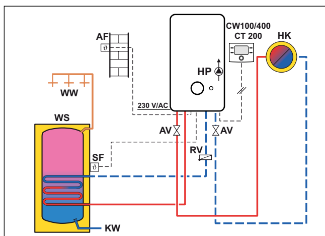
Obr. 10 Příklad s ekvitermním regulátorem CW100/CW400 a CT 200
