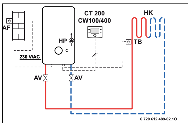
Obr. 3 Příklad s ekvitermním regulátorem CW100/CW400 a CT 200 a podlahovým vytápěním s průtokem do 1000 l/h
