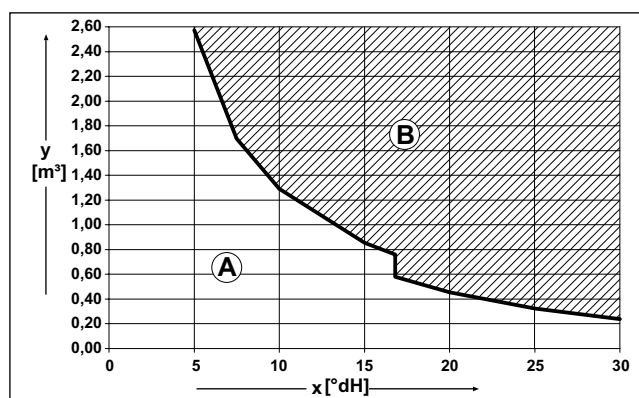
Obr. 30 Požadavky na plnicí a doplňovací vodu u přístrojů < 50 kW
