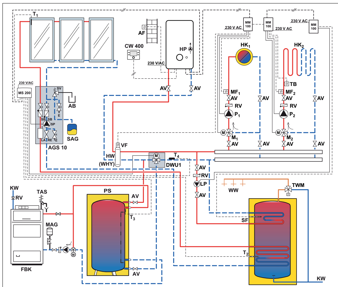
Obr. 22 Kondenzační kotel s kotlem na tuhá paliva a se solární přípravou teplé vody a dvěma otopnými okruhy
