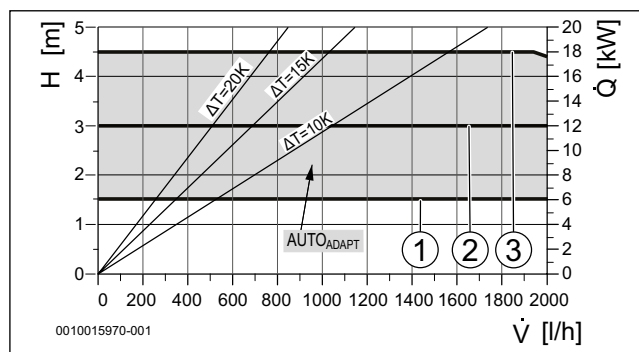
Obr. 100 Charakteristiky čerpadla při konstantním tlaku
