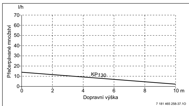
Obr. 38 Graf čerpadla kondenzátu
