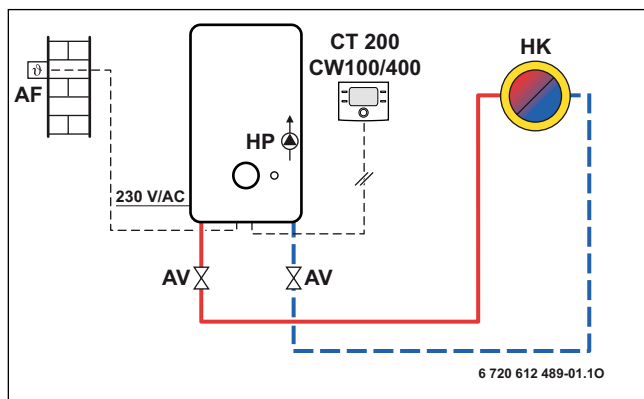
Obr. 1 Příklad s ekvitermním regulátorem CW100/CW400 a CT 200
