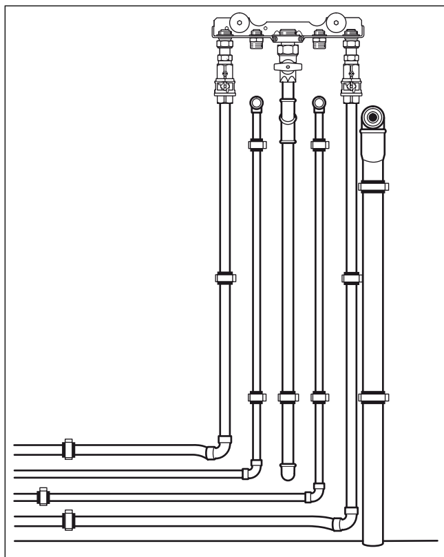
Obr. 46 Nástěnné potrubní propojení na straně stavby s odstupem od stěny 60 mm
