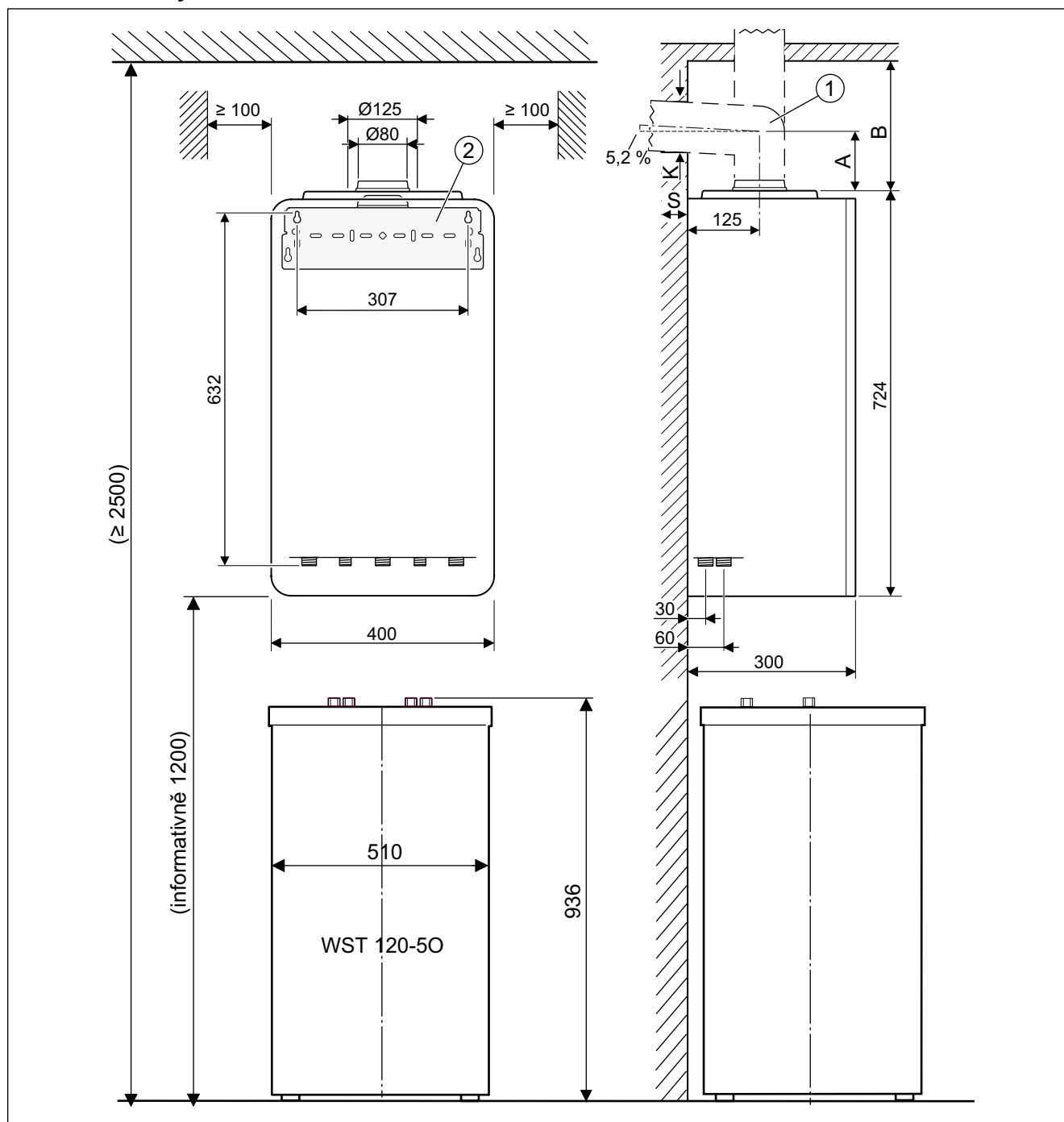
Obr. 52 Informativní výkres kotle Condens GC2300iW 15/25 P se zásobníkem WST 120-50
