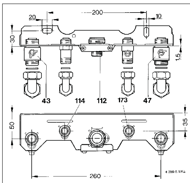
Obr. 27 Vertikální montážní připoj. lišta č. 869, pro připojení nutno doplnit Propojení (obj. č. 7 736 901 403)
