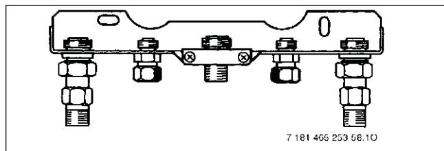
Obr. 32 Montážní připojovací lišta s uzavíracími krytkami (příslušenství č.304)
