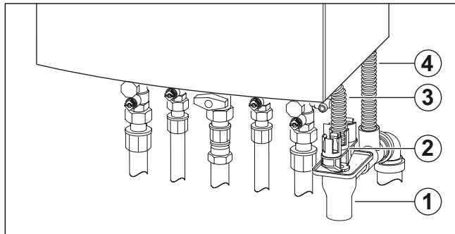
Obr. 29 Trychtýřový sifon s odkapovým adaptérem (příslušenství č. 432)
