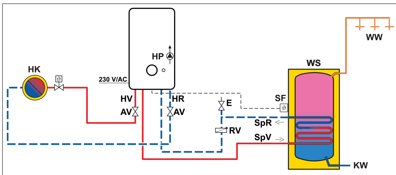
Obr. 53 Příklad zapojení kotle Condens GC2300iW 24 P s vedle stojícím zásobníkem teplé vody
