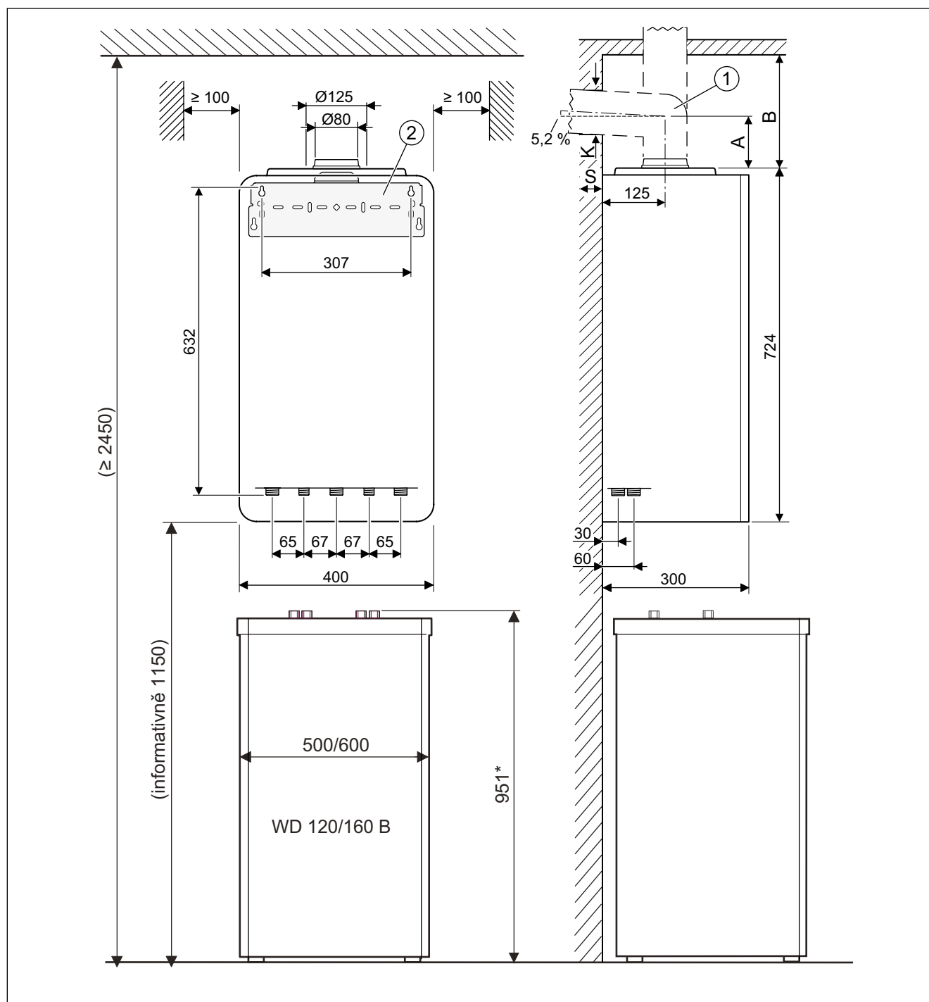
Obr. 51 Informativní výkres Condens GC 2300iW... se zásobníkem WD 120/160 B
