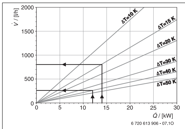
Obr. 97 Diagram k určení průt. množství v otopném okruhu
