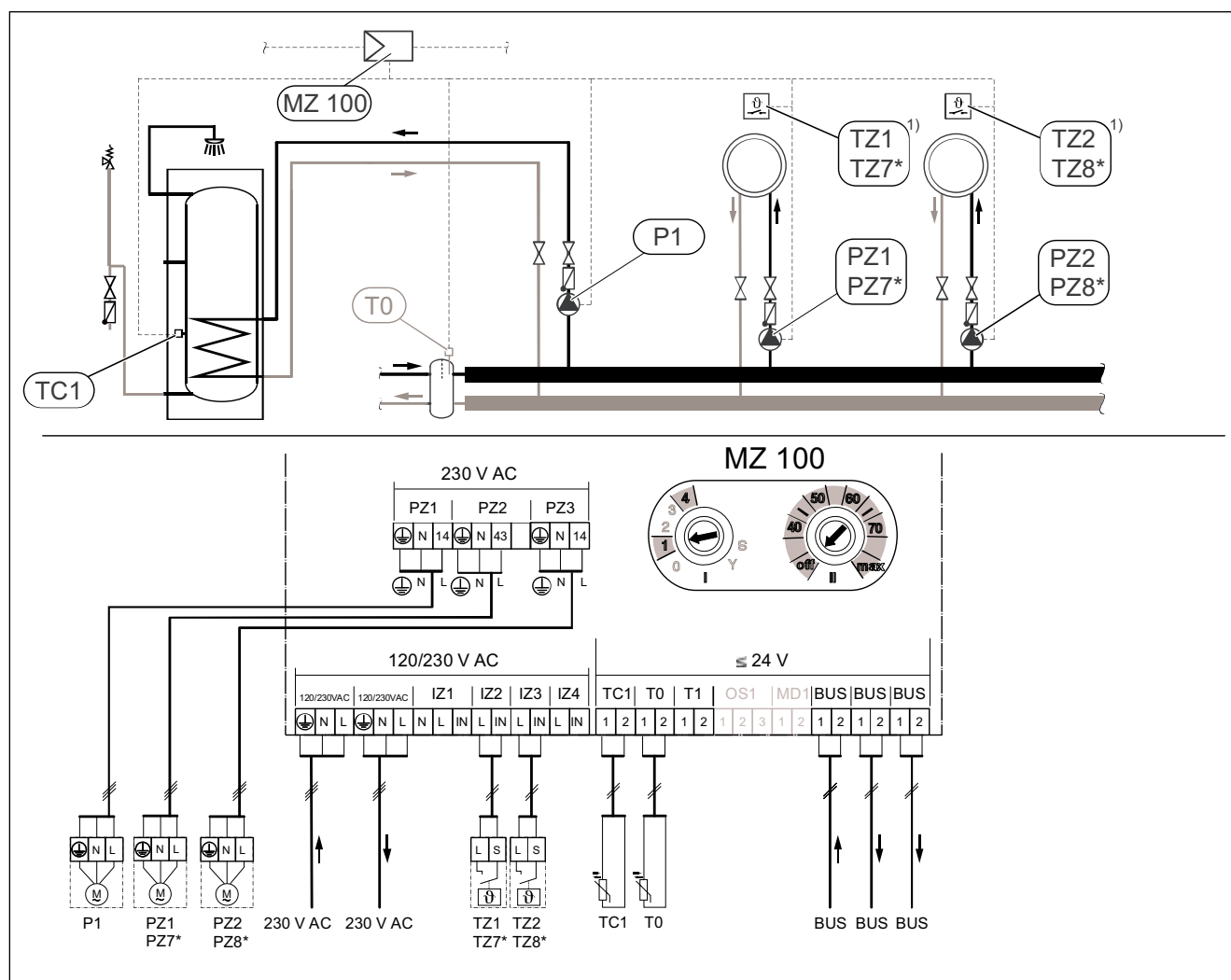
Obr. 23 Příklad užití modulu MZ 100 v otopné soustavě
