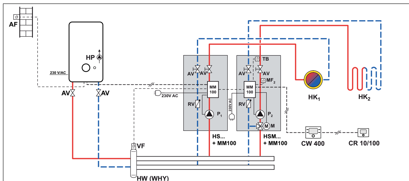
Obr. 5 Příklad dvou otopných okruhů s rychlomontážními sadami HS / HSM, instalaci lze realizovat i s využitím kompaktní rychlomontážní sady pro oba okruhy MCM101 MM200 V2 (viz schéma na str. 8 obr. 8)
