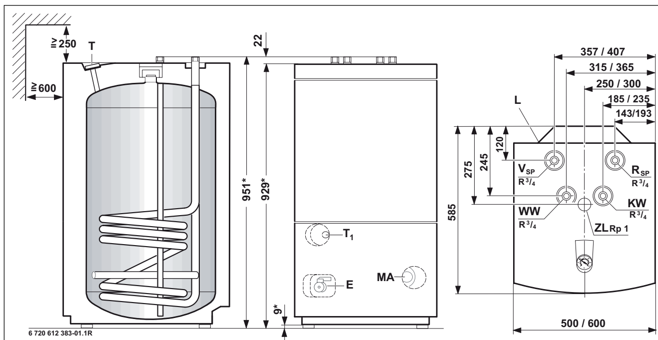
Obr. 42 Montážní a připojovací rozměry WD 120/160 B (údaje o rozměrech za lomítkem se vztahují k nejbližšímu většímu provedení zásobníku)
