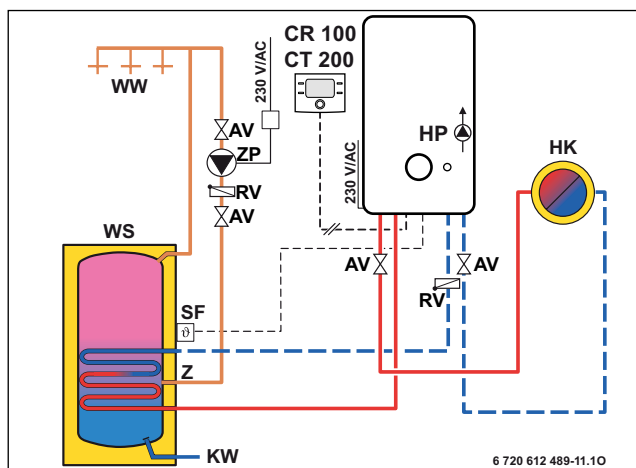
Obr. 13 Příklad s regulátorem CR 100 nebo CT 200 řízeným podle teploty prostoru a externě řízenou cirkulací teplé vody
