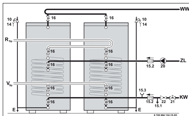
Obr. 41 Paralelní řazení
