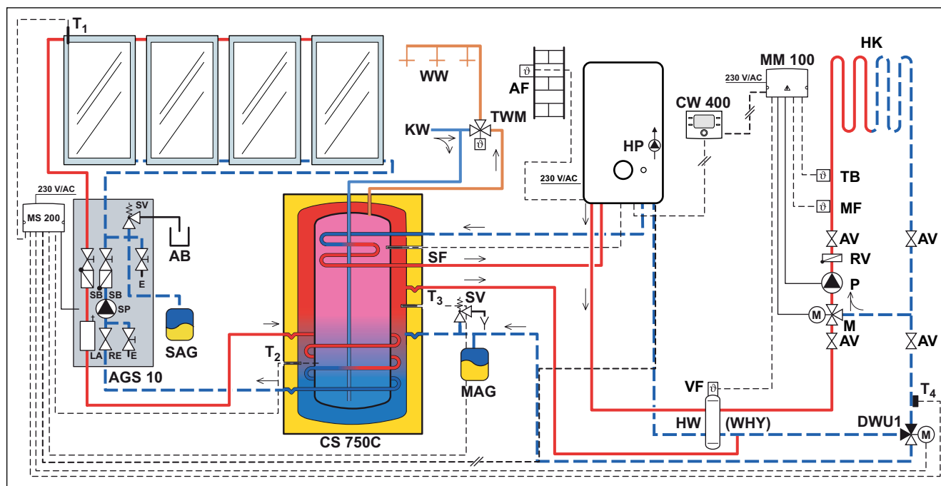
Obr. 21 Příklad solární podpory vytápění se směřovaným otopným okruhem
