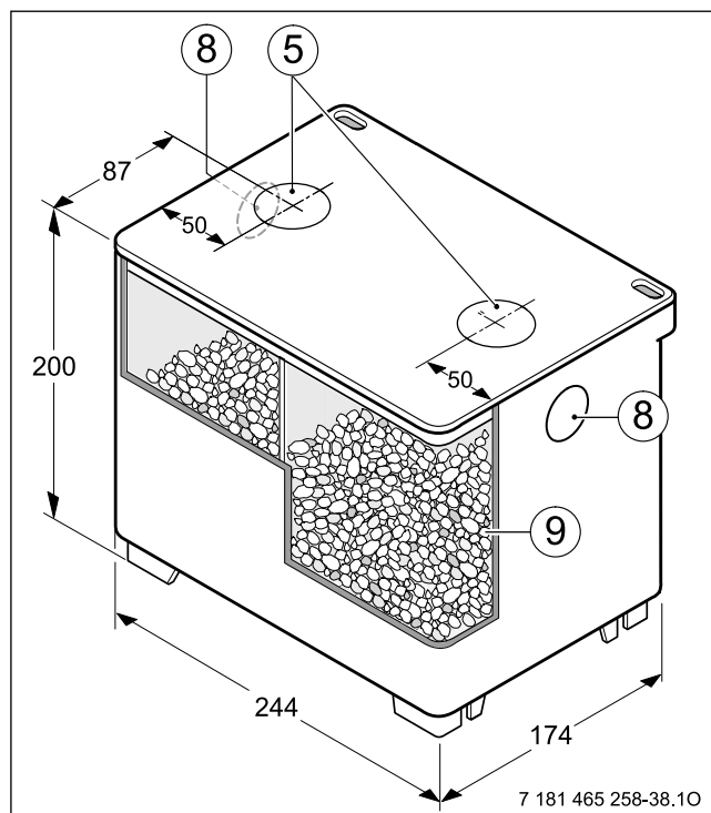
Obr. 39 Neutralizační box
