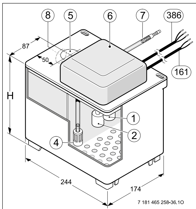
Obr. 37 Čerpadlo kondenzátu
