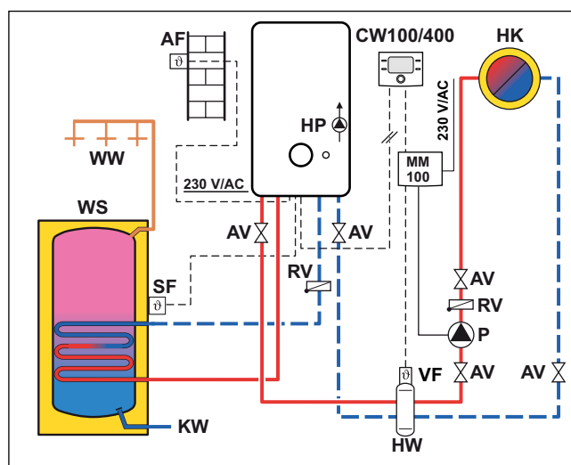
Obr. 15 Příklad nesměšovaného otopného okruhu s požadovaným průtokem otopné vody nad 1000l/hod
