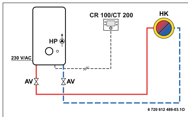
Obr. 2 Příklad s prostorovým regulátorem CR 100 a CT 200
