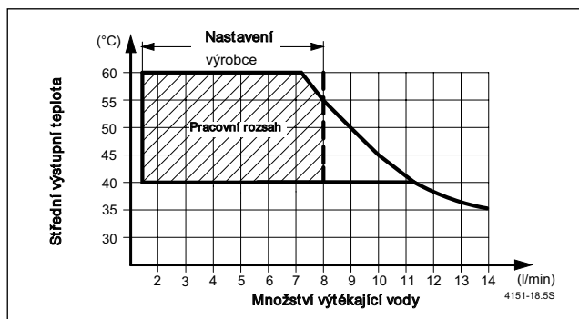
Obr. 59 Výtok teplé vody
