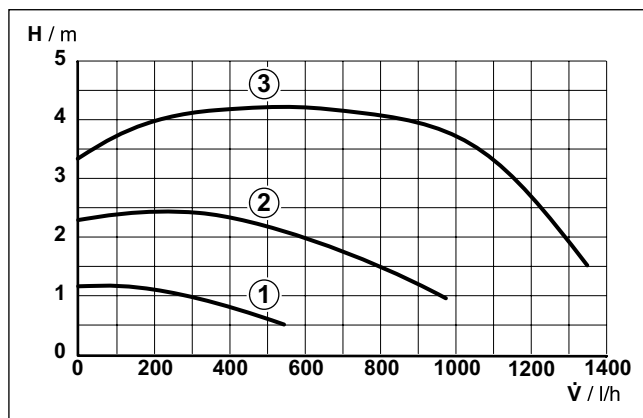
Obr. 36 Provoz při proporcionálním tlaku s vestavěným energeticky úsporným a elektronicky řízeným oběhovým čerpadlem
