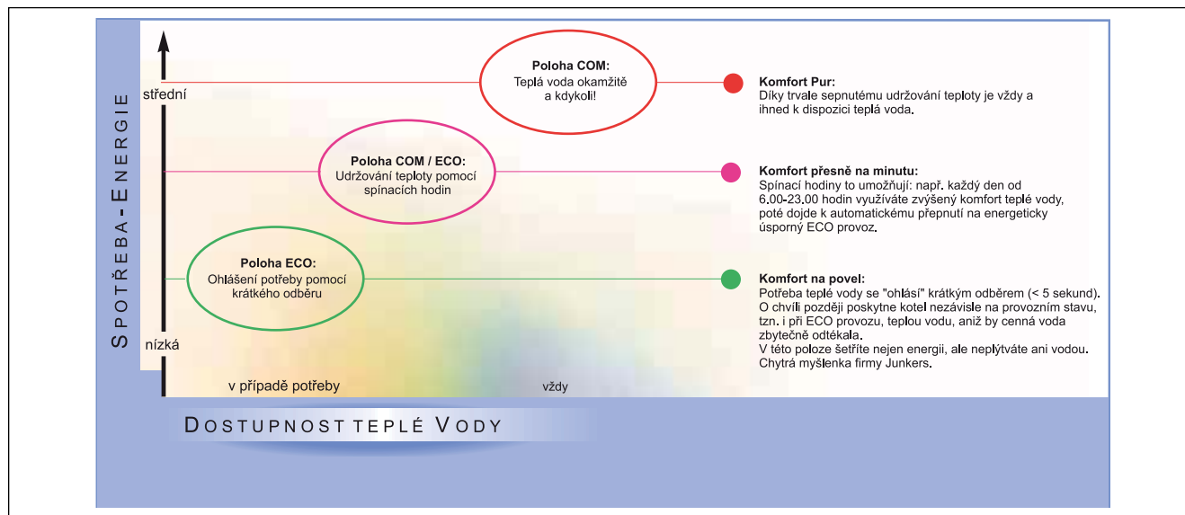
Obr. 58 Možnosti nastavení komfortu teplé vody
