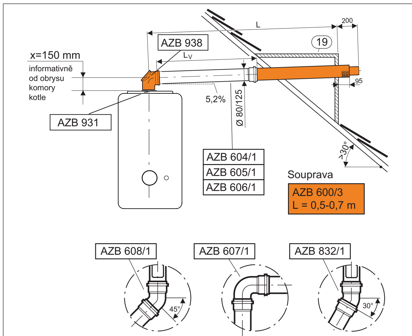
Obr. 83 Možno použít i novou sadu AZB 918 s kolenem s měřicími body a připojovací přírubou (bez revizního T-kusu a bez potřeby AZB 931)
