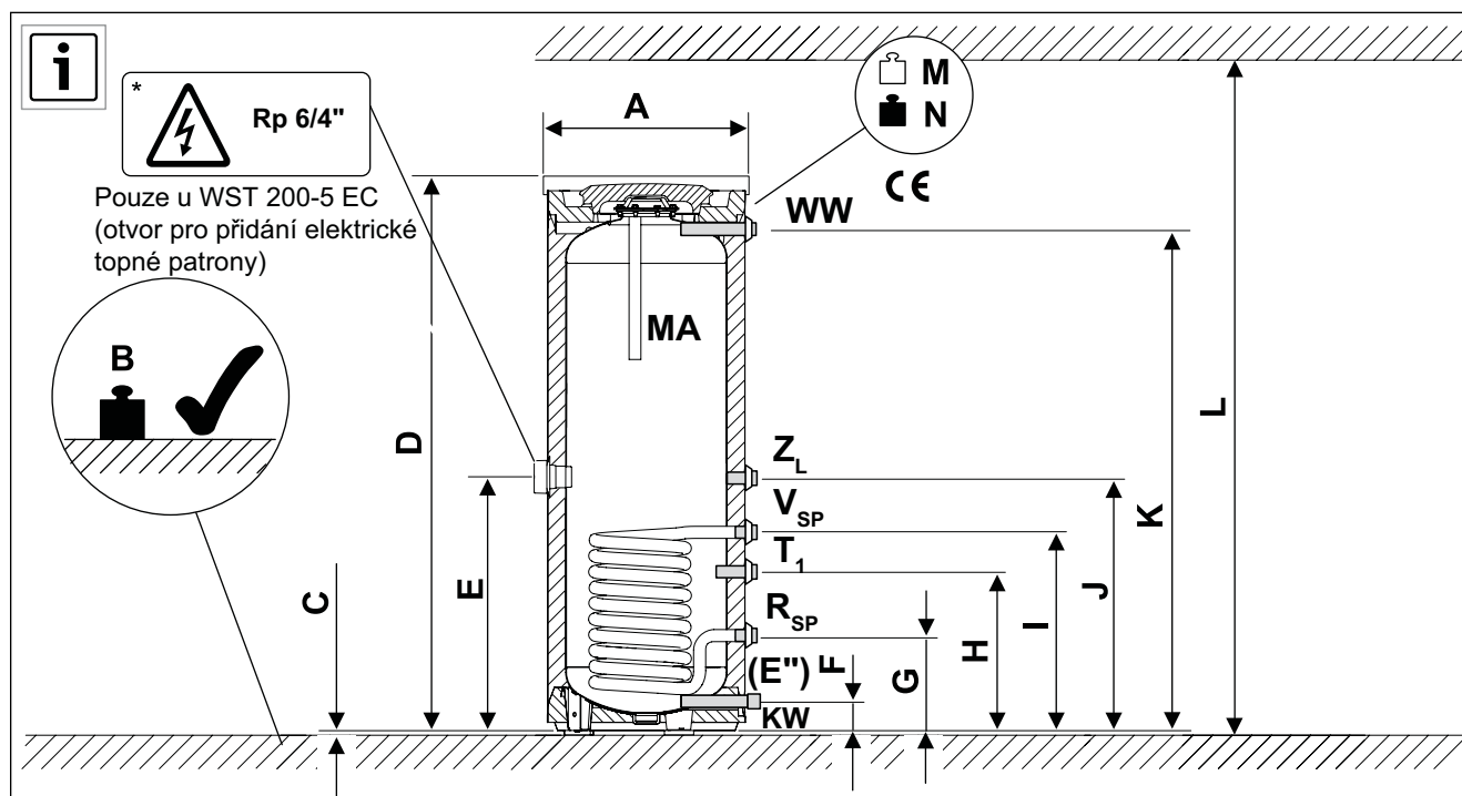
Obr. 54 Montážní a připojovací rozměry WST 120/160/200 - 5 (E) C
