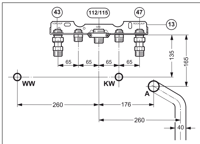
Obr. 47 Připojky na omítku bez odstupu od stěny
