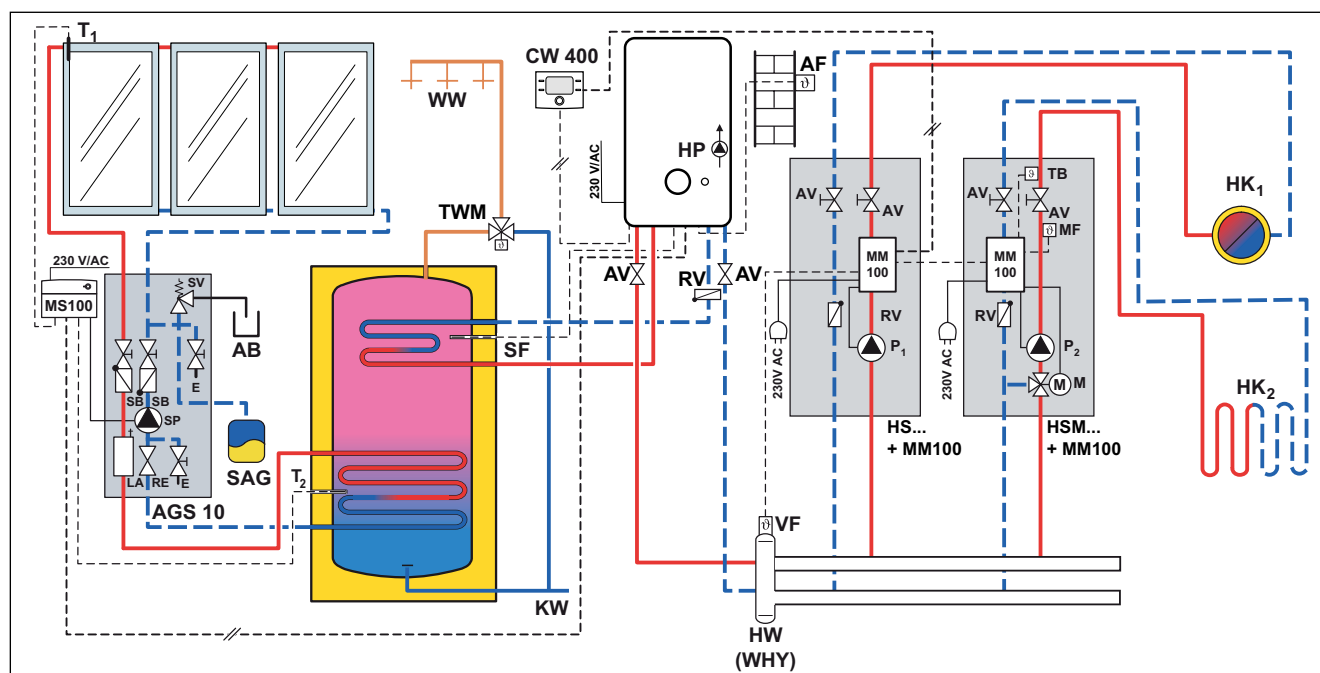
Obr. 20 Příklad solární přípravy teplé vody s jedním nesměšovaným a jedním směšovaným otopným okruhem
