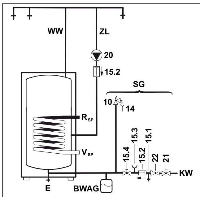
Obr. 40 Schéma připojení teplé vody
