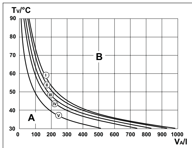
Obr. 31 Charakteristiky expanzní nádoby
