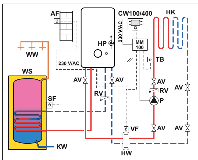
Obr. 14 Příklad podlahového vytápění s požadovaným průtokem otopné vody nad 1000l/h
