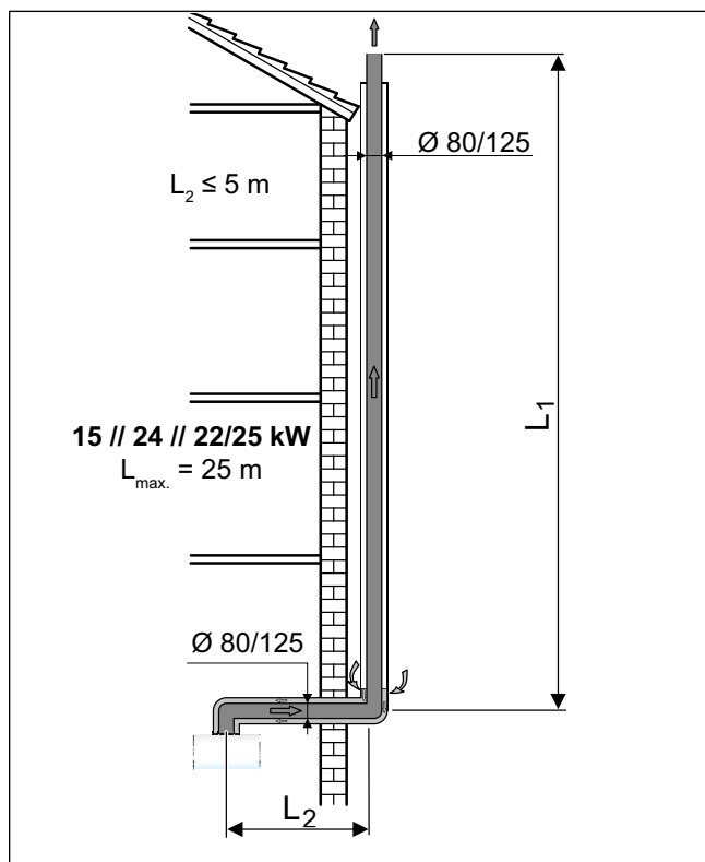
Obr. 90 Vedení odtahu spalin po fasádě podle C53(x)
