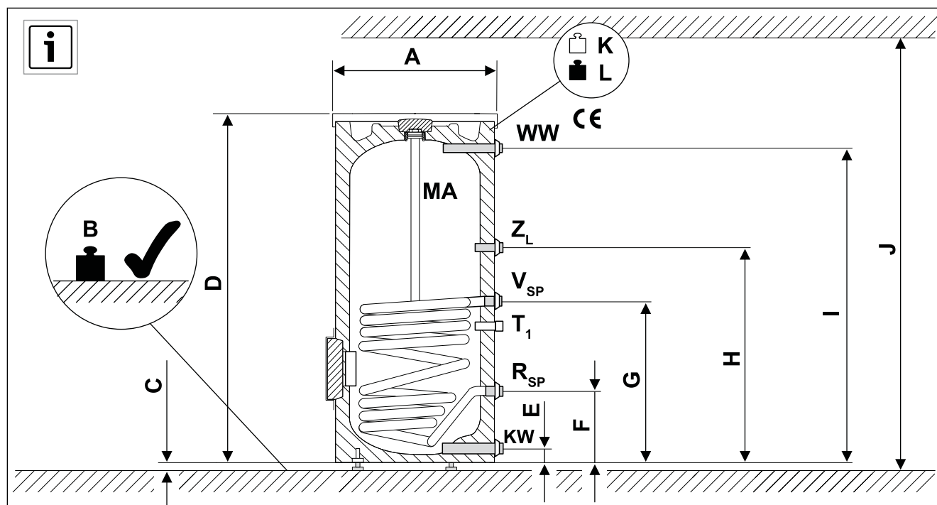
Obr. 55 Montážní a připojovací rozměry WST 300/400 - 5 C
