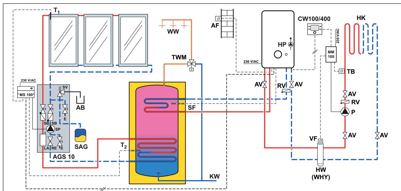
Obr. 19 Příklad solární přípravy teplé vody a termohydraulického rozdělovače
