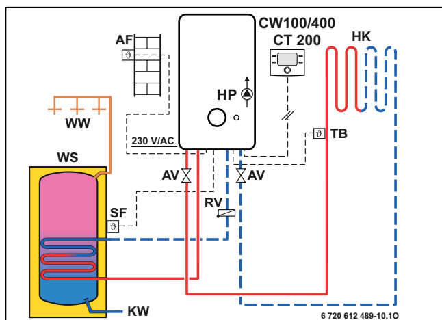
Obr. 12 Příklad s ekvitermním regulátorem CW100/CW400 a CT 200 a podlahovým vytápěním s průtokem otopné vody do 1000l/h
