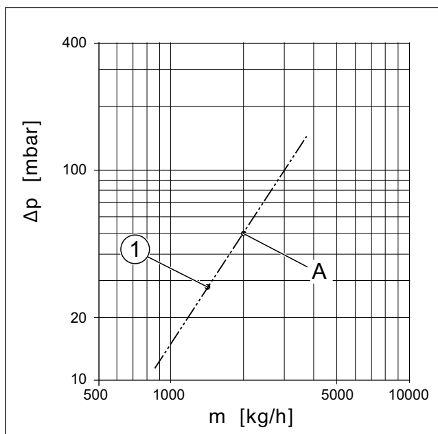
Obr. 50 WST 120-50
