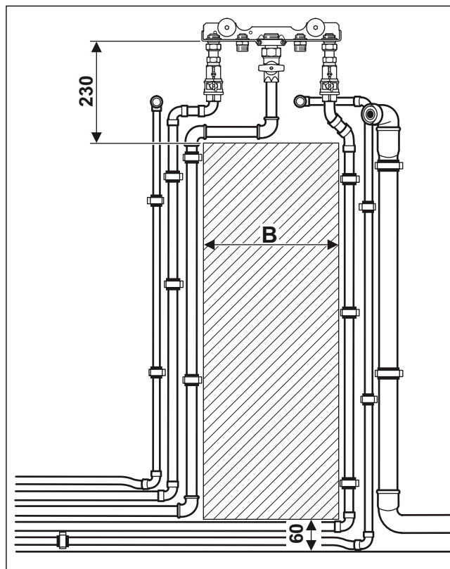
Obr. 48 Nástěnné potrubní propojení na straně stavby bez odstupu od stěny
