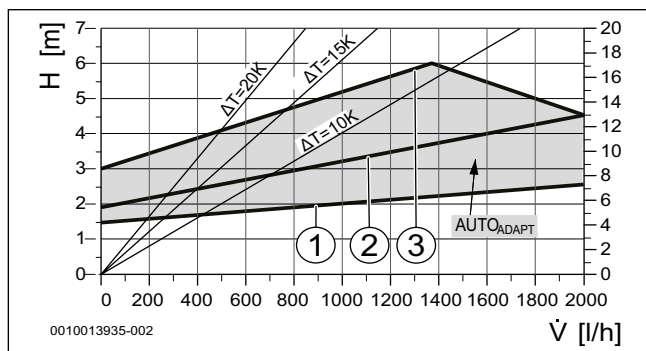
Obr. 99 Charakteristiky čerpadla při proporcionálně rostoucím tlaku
