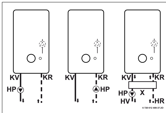
Obr. 34 Sériové řazení čerpadel vytápění
