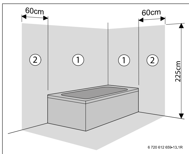
Obr. 61 Ochranné úseky
