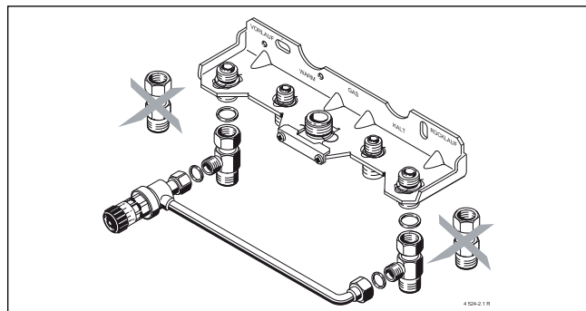
Obr. 33 Přepouštěcí ventil příslušenství č. 687 pro montážní připojovací lištu příslušenství č. 258 nebo č. 869
