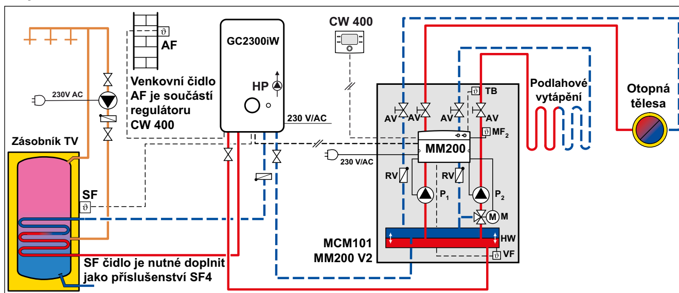
Obr. 8 Příklad dvou otopných okruhů řešených s rychlomontážní sadou MCM101 MM200 V2
