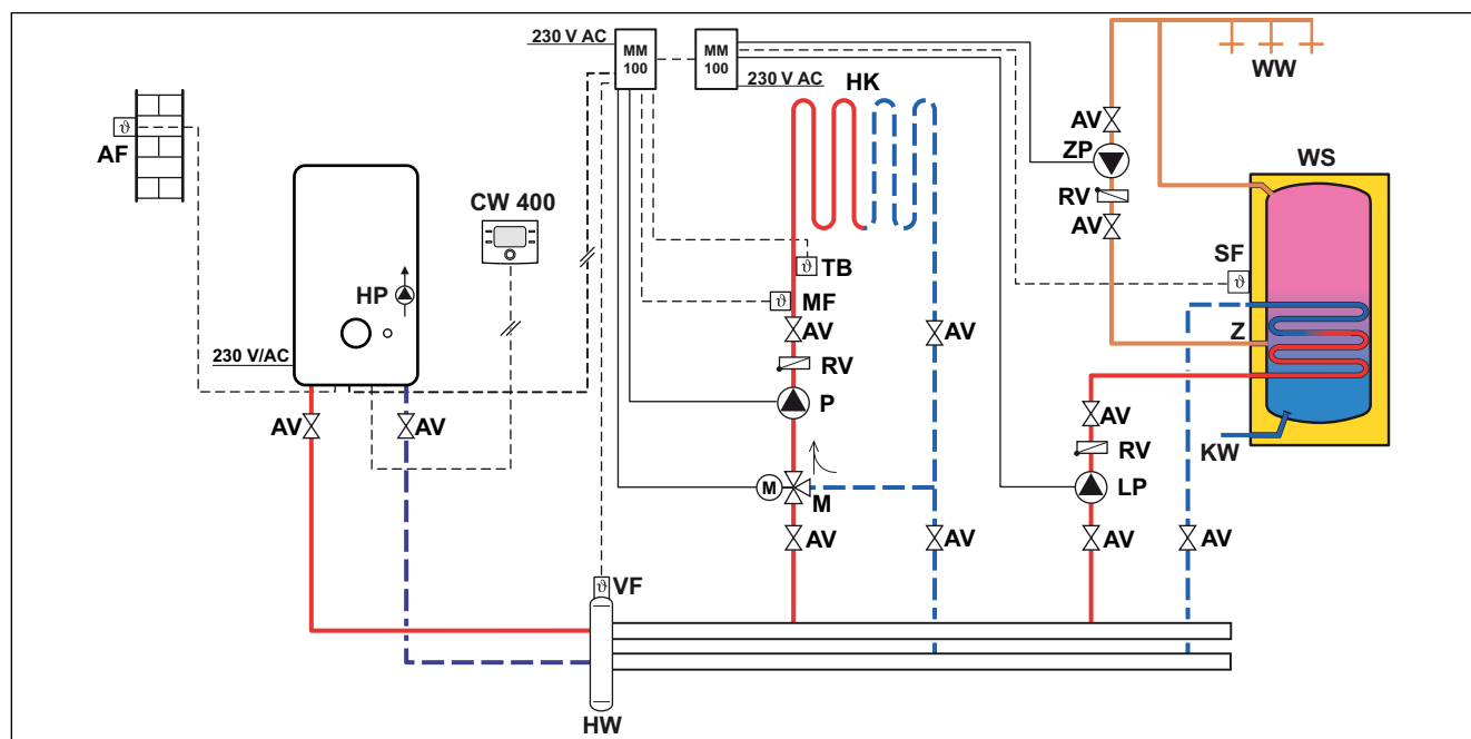
Obr. 16 Příklad termohydraulického rozdělovače se zásobníkem teplé vody a jedním směšovaným otopným okruhem
