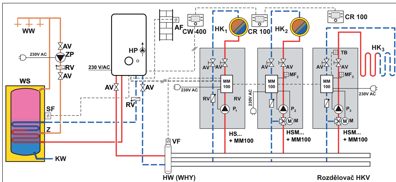
Obr. 17 Příklad otopné soustavy se zásobníkem teplé vody a třemi otopnými okruhy řešenými pomocí rychlomontážních sad HS.../HSM...
