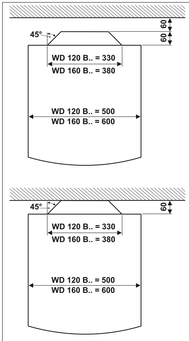
Obr. 45 Odstupy od stěn místnosti
