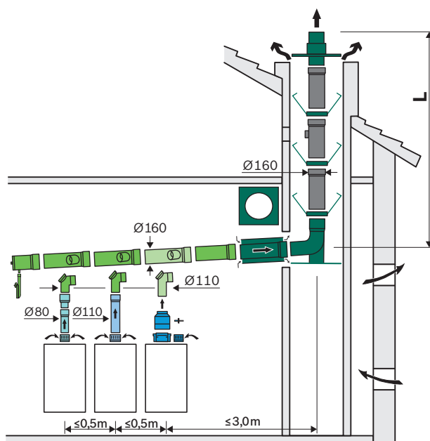
Lunghezze massime ammesse [m] per sistemi fumari in cascata B23(p) per caldaie da 14 a 35 kW, con PP rigido da DN160 mm
