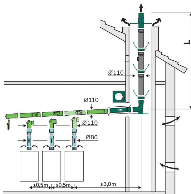
Lunghezze massime ammesse [m] per sistemi fumari in cascata B23(p) per caldaie da 14 a 35 kW; con PP rigido da DN110 mm
