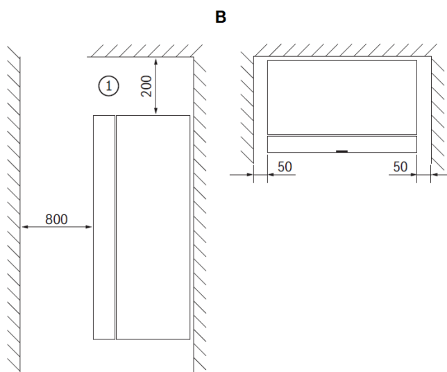
[B] Unità interna murale AWEi
