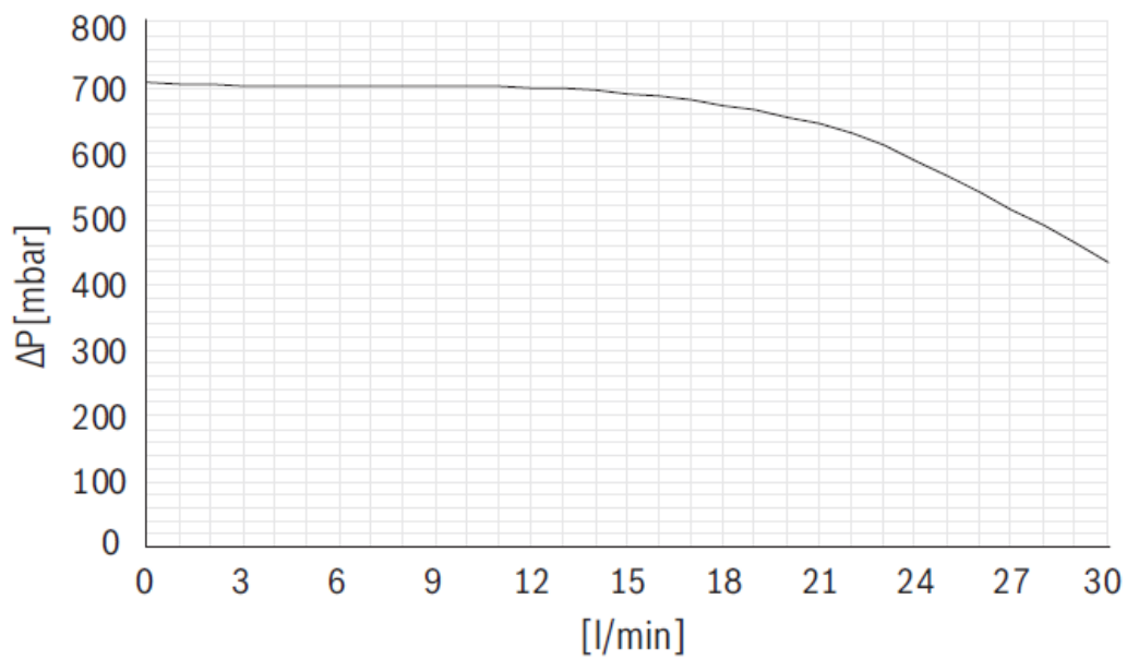
Curva caratteristica circolatore PC0 unità interna AWMi
