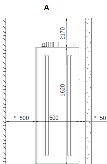
[A] Unità interna tower AWMi e AWMHi
