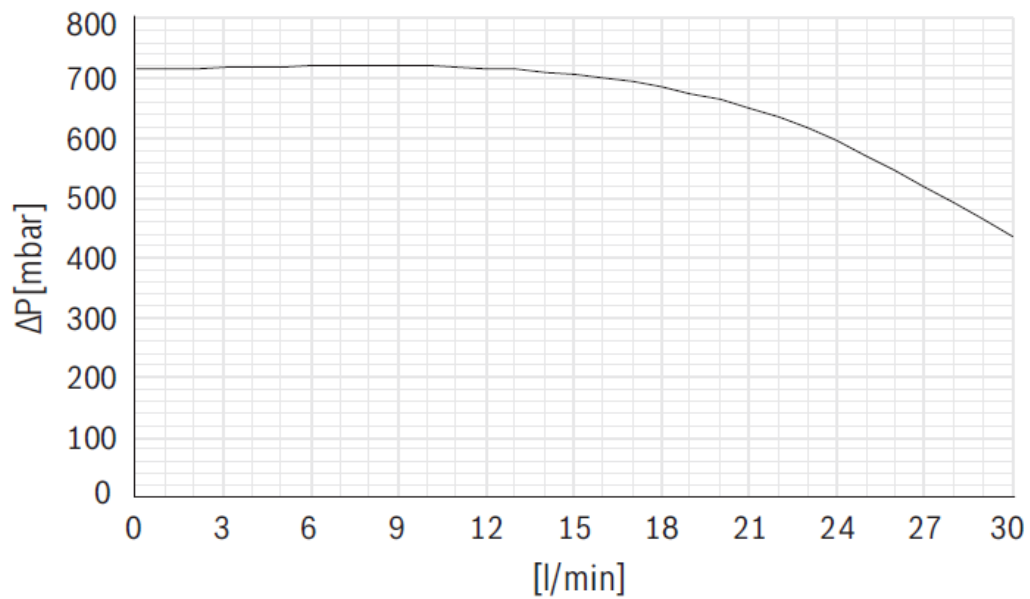
Curva caratteristica circolatore PC0 unità interna AWEi
