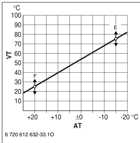
Fig. 9 Curva di riscaldamento
