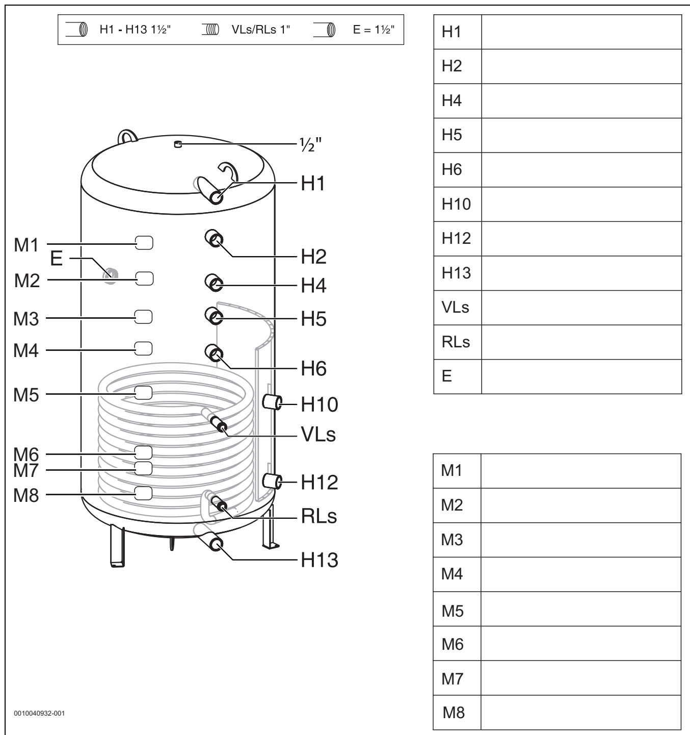
Fig. 28 BS 500, 750, 1000, 1300-6 ER
