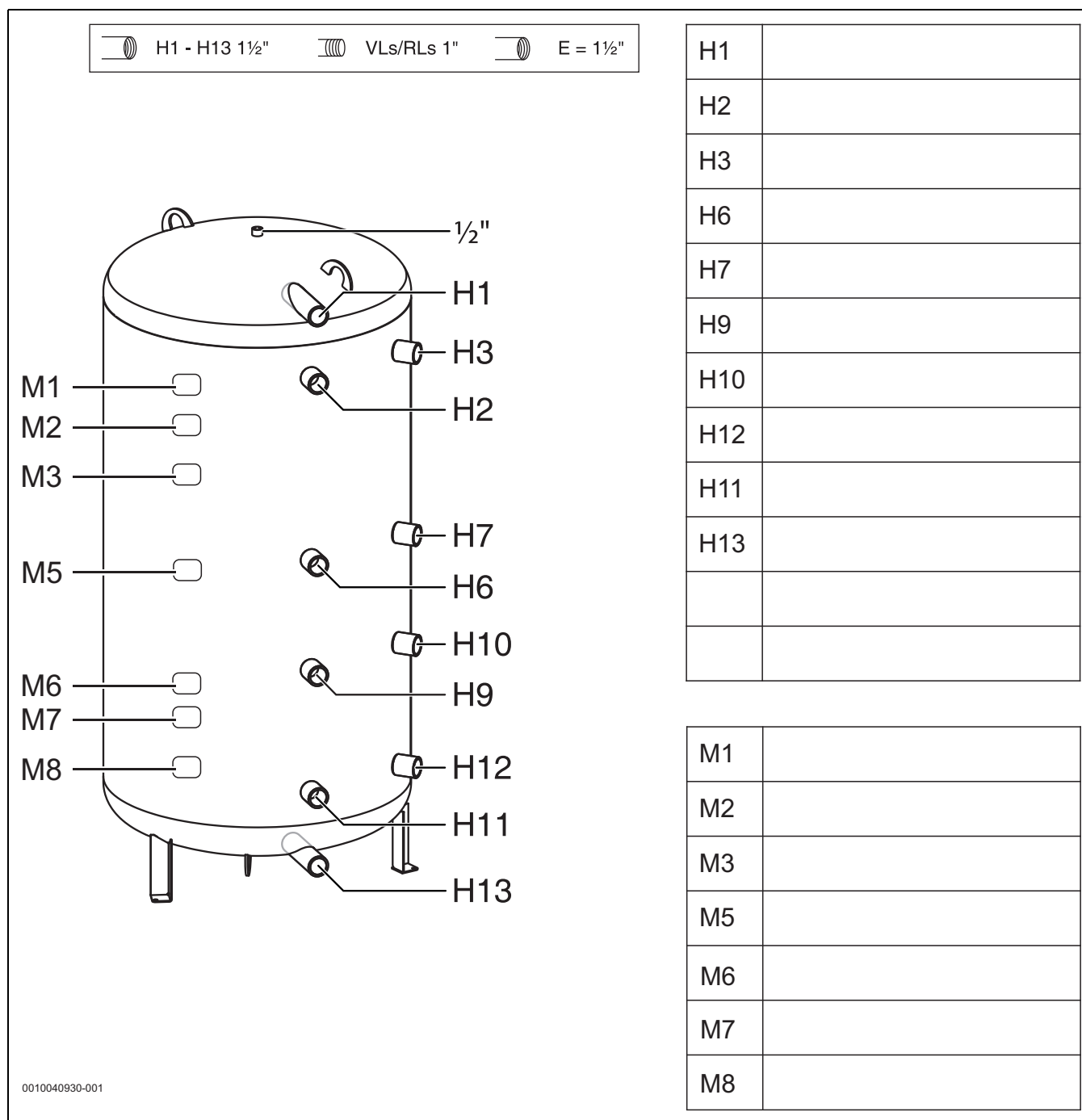
Fig. 26 B 500, 750, 1000, 1300-6 M
