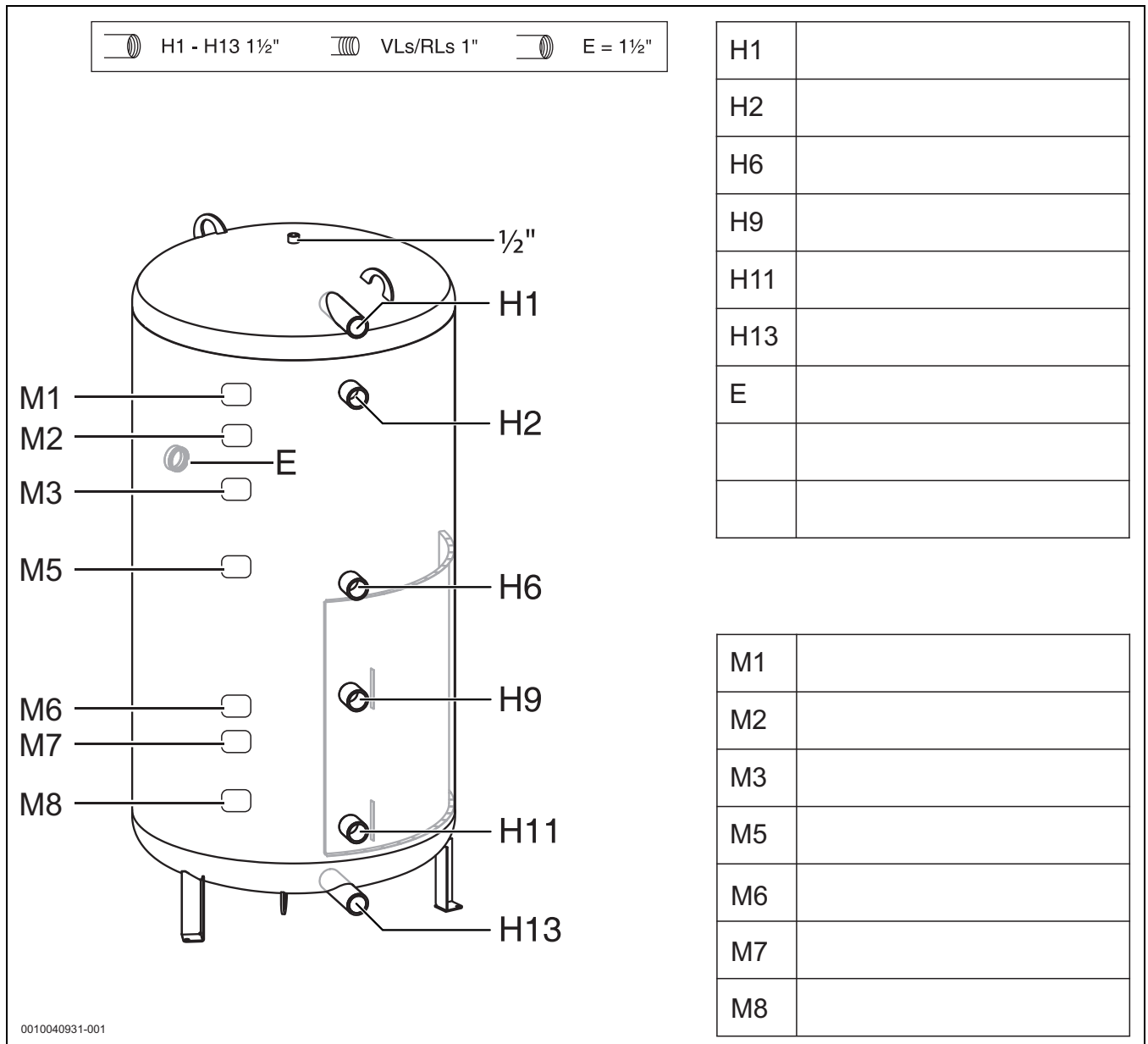
Fig. 27 B 500, 750, 1000, 1300-6 ER
