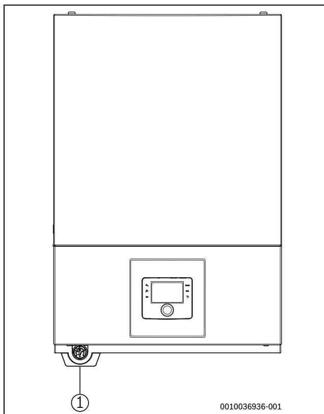
Fig. 5 AWS E unité intérieure (vue avec bac de récupération)
