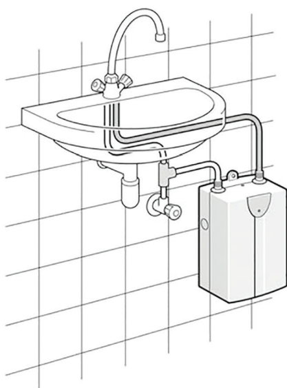
Installation Tronic 1000 T sous évier
