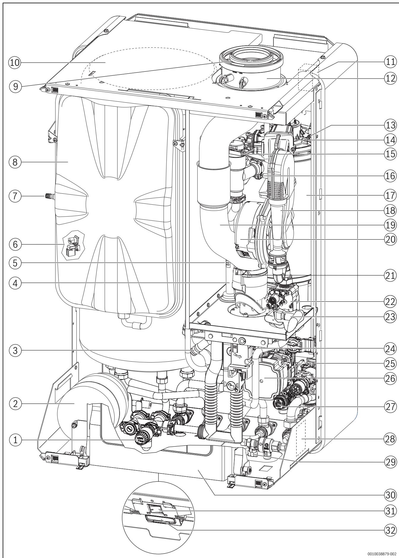
Fig. 5 Structura echipamentului
