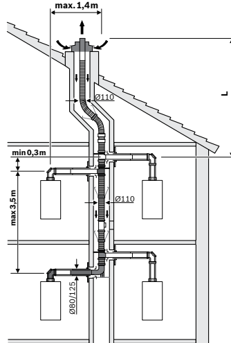
Zestaw podstawowy C14 (3x) do szachtu Zestaw podstawowy C14 (3x) w szachcie
