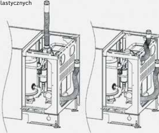
Podłączenie boczne lub boczne/górne za pomocą węży elastycznych
