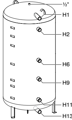
BS 500, 750, 1000 1300-6 ER
