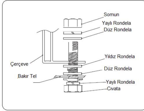
Şekil 7: Topraklama yöntemi şematik gösterimi
