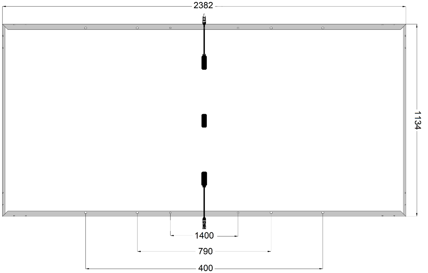
Şekil 1: SPE 620-132GGT/ SPE 625-132GGT/ SPE 630-132GGT panel boyutlandırması
