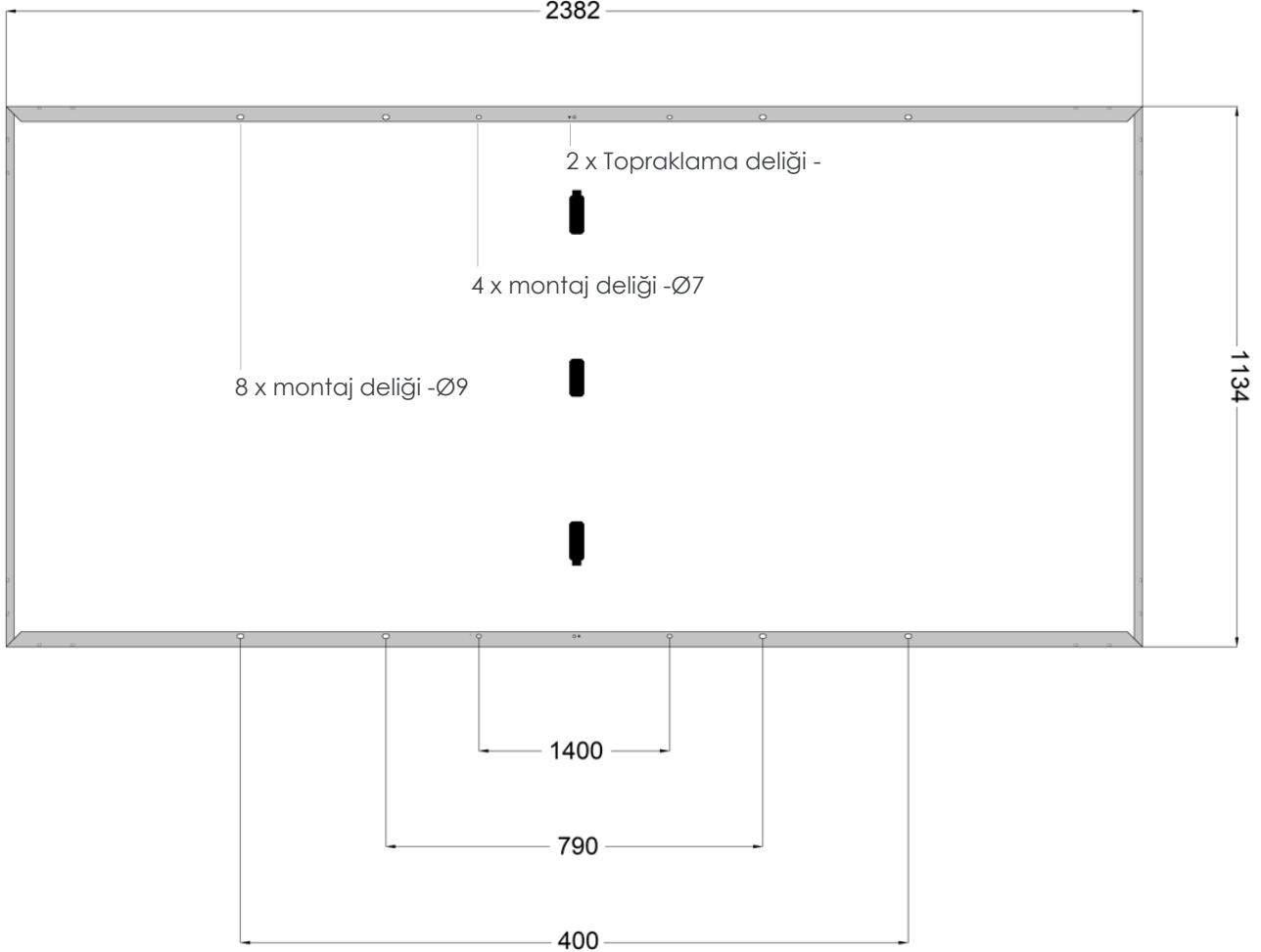
Şekil 2: Montaj deliklerine göre kurulum
