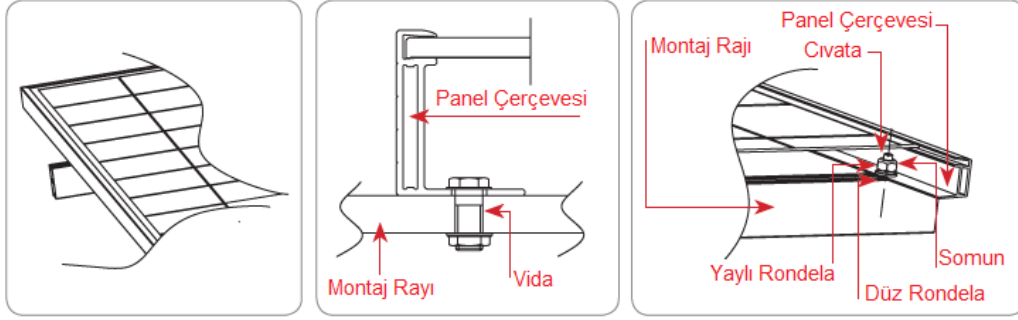
Şekil 2: Montaj deliklerine göre kurulum
