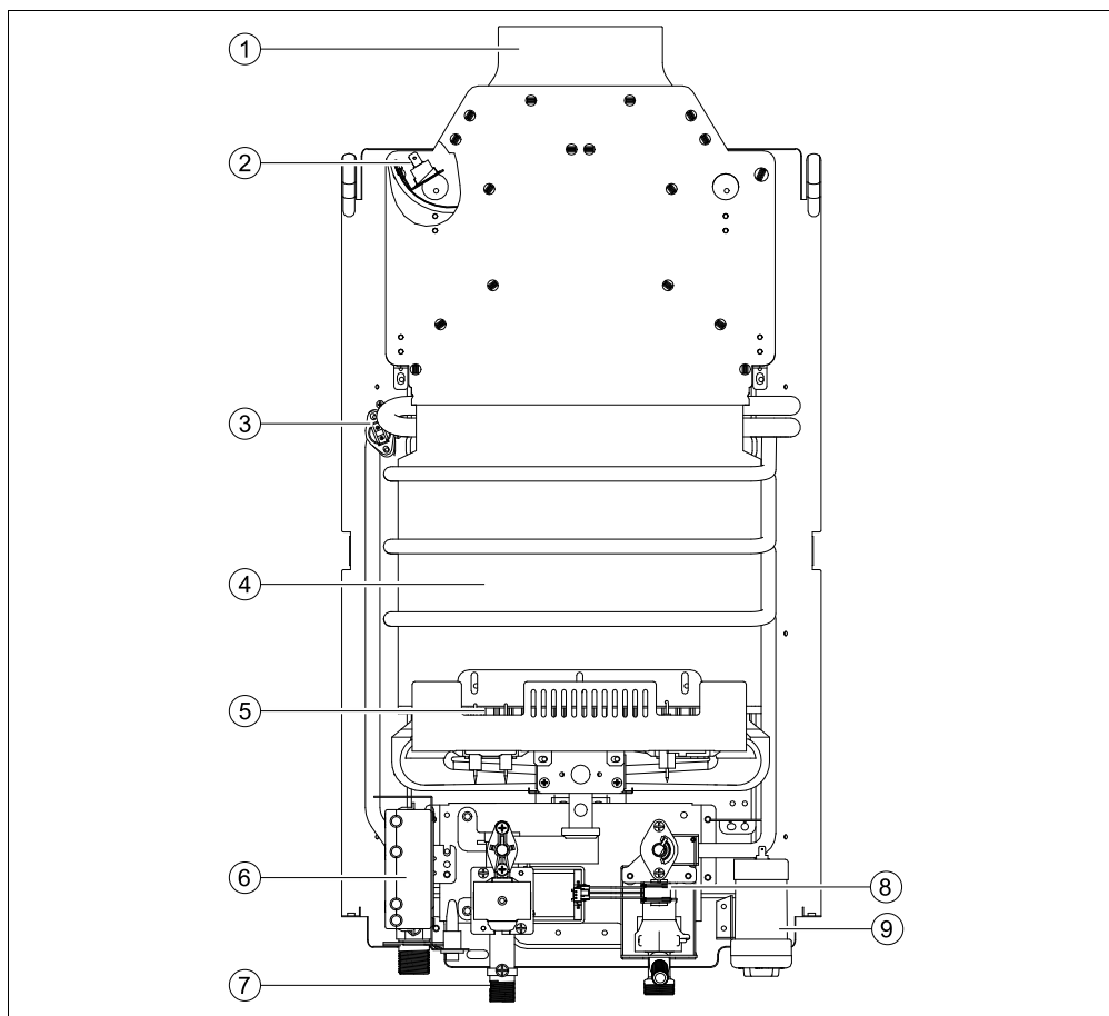
Fig. 2 Vista general del aparato
