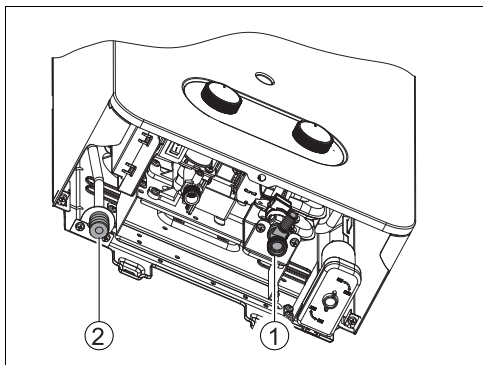
Fig. 16 Conexión de agua
