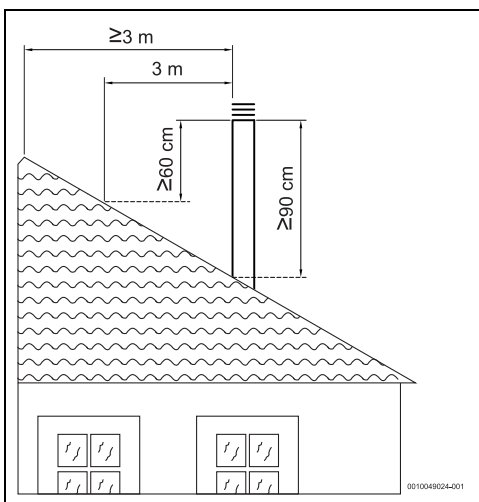
Fig. 14 Distancia del ducto a más de 3 metros de la cumbrera más alta
