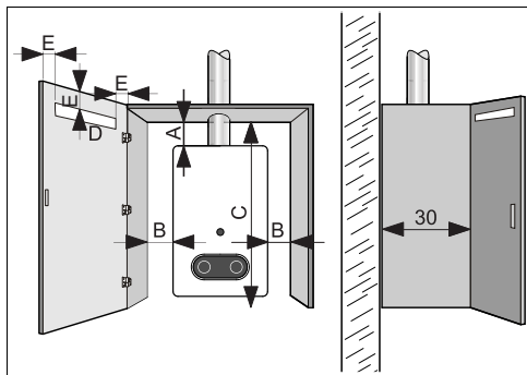
Fig. 11 Instalación en casetas
