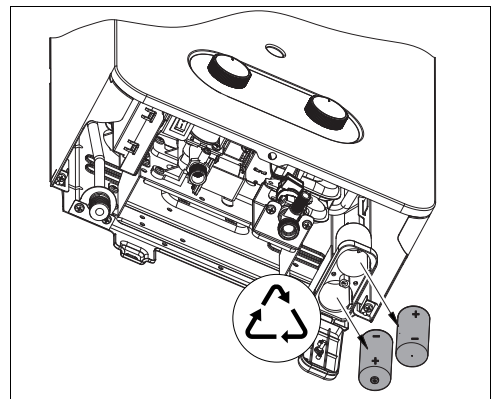
Fig. 4 Cambiar las baterías
