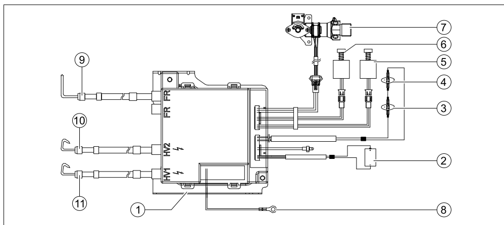
Fig. 18 Esquema eléctrico
