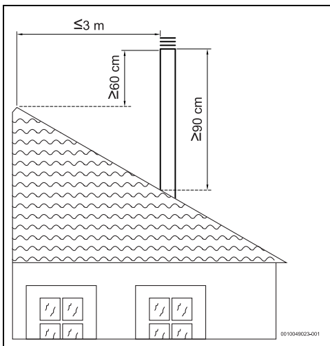
Fig. 13 Distancia del ducto a menos de 3 metros de la cumbrera más alta
