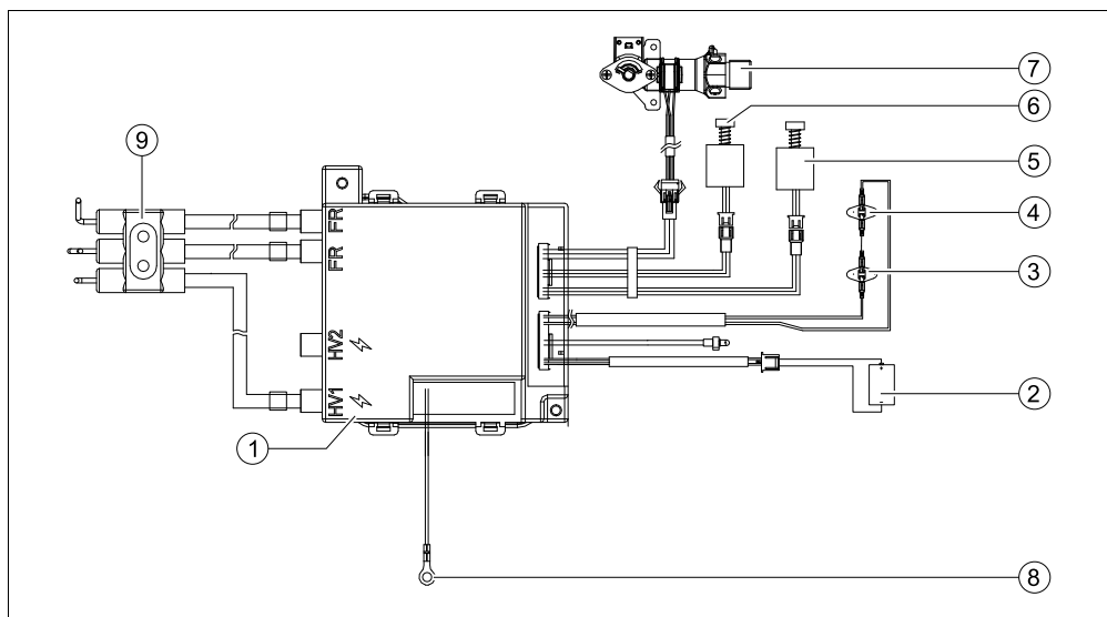
Fig. 16 Esquema eléctrico
