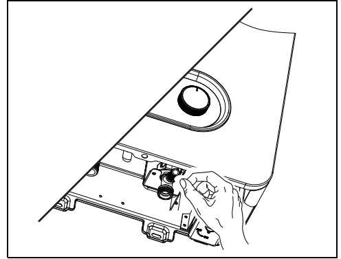
Fig. 10 Vaciado
