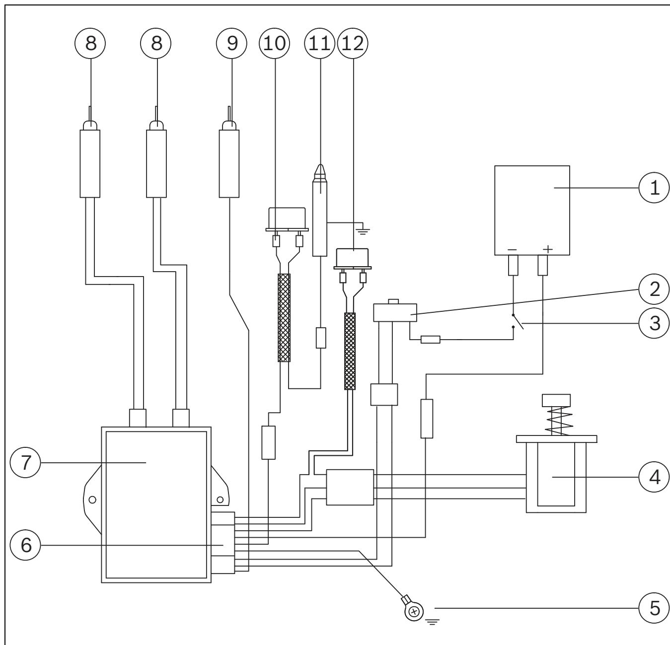
Fig. 3 Esquema eléctrico
