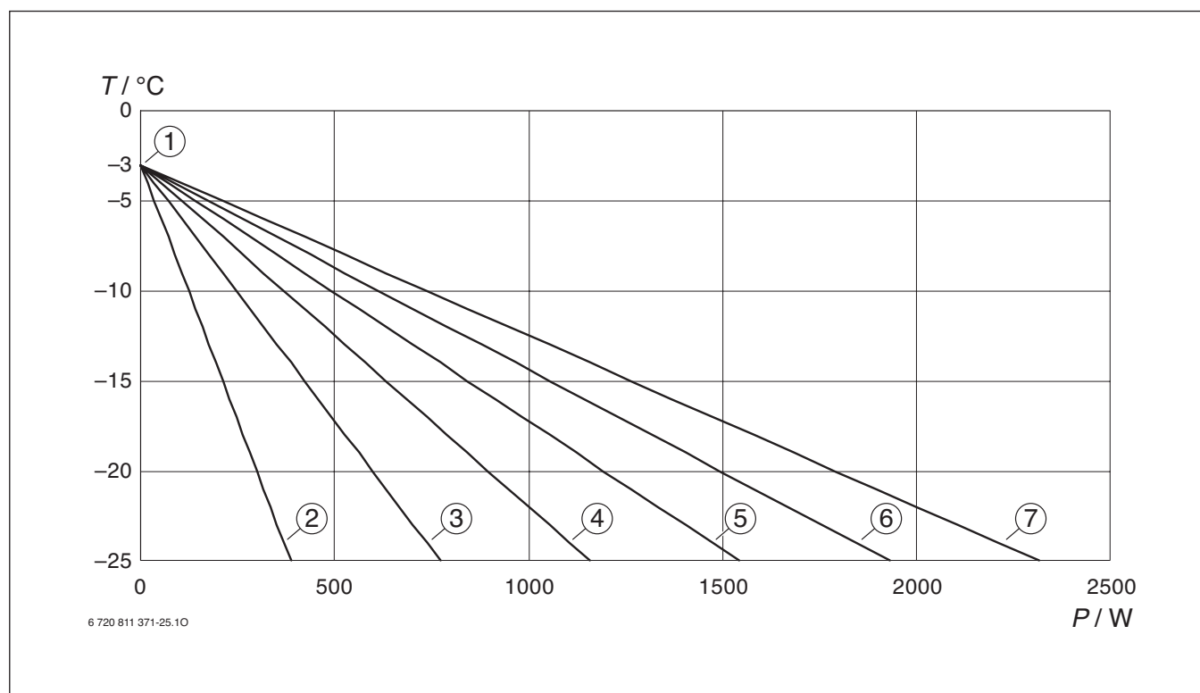
Rys. 12 Wymagana moc cieplna modułu podgrzewania wstępnego w zależności od temperatury zewnętrznej
