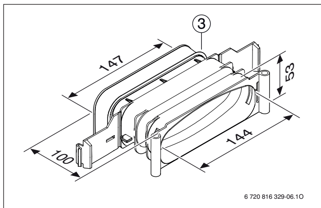
Rys. 129 FKV 140-3
