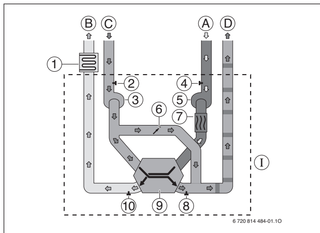
Rys. 9 Zasada działania
