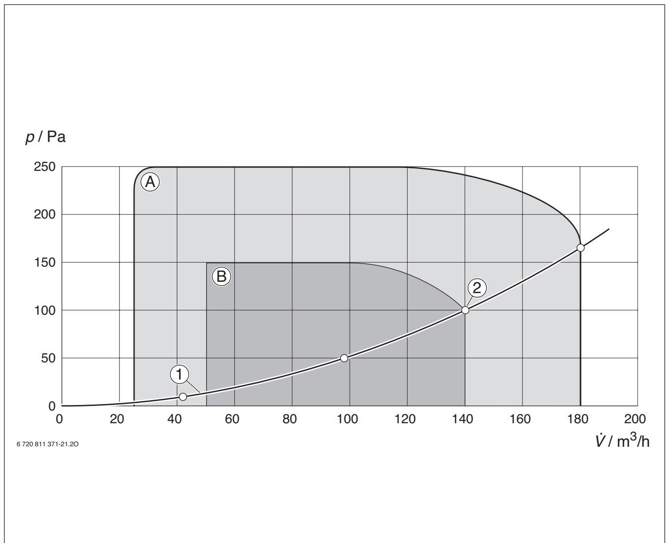
Rys. 33 Charakterystyki wzrostu ciśnienia/strumienia objętości LP 140-2
