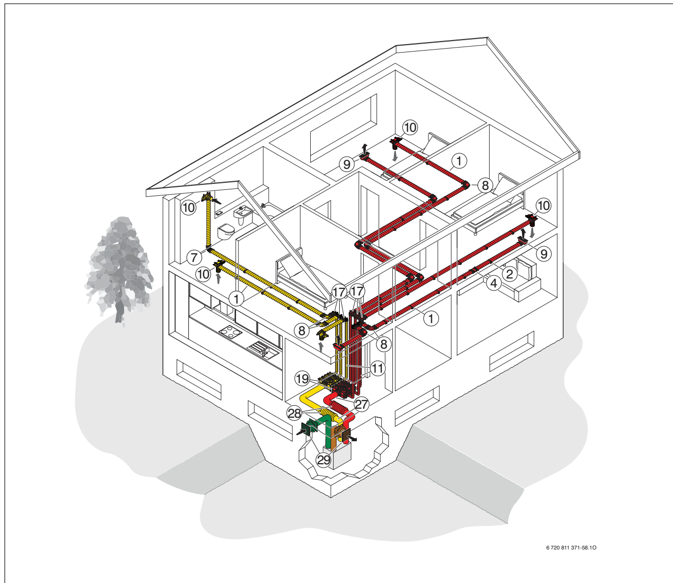
Rys. 7 Dom systemowy Junkers AerastarComfort LP...-2
