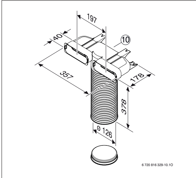
Rys. 124 FKU 140-1
