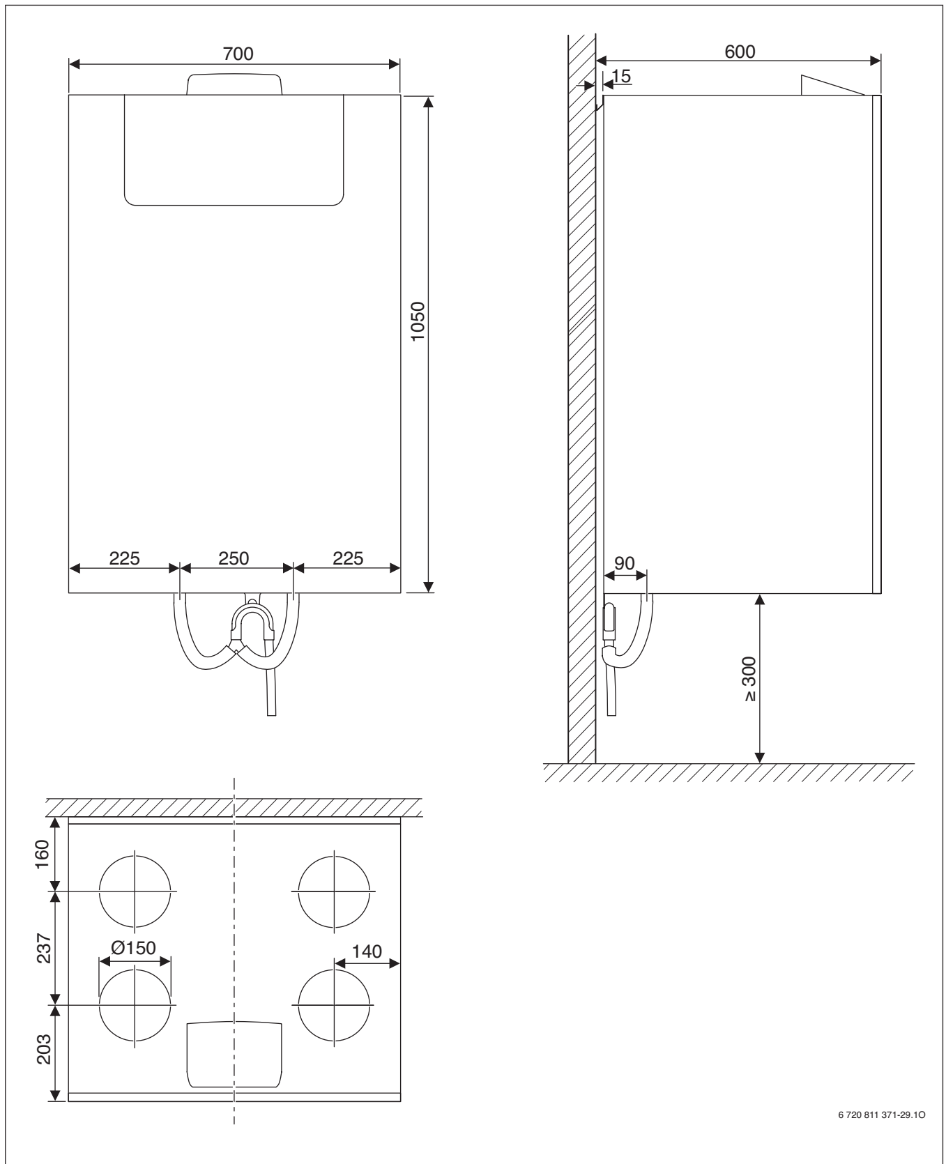
Rys. 29 AerastarComfort LP 230-2 (wymiar w mm)
