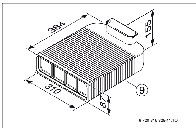
Rys. 135 FKU 140-2
