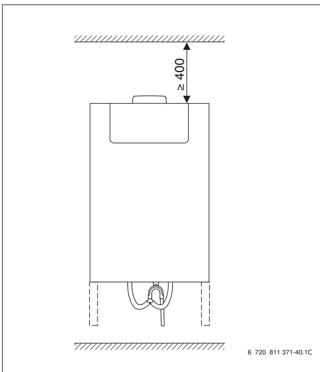
Rys. 32 Minimalne wymiary montażowe LP 230-2, LP 350-2
