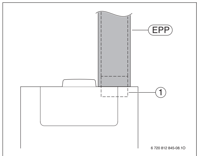
Rys. 67 Podłączenie rury z EPP
