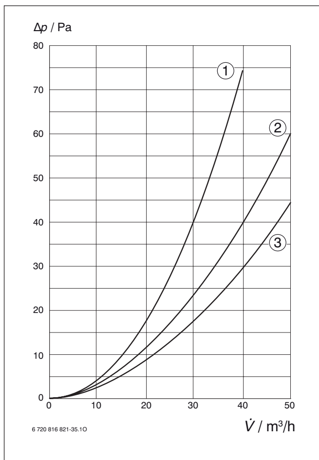
Rys. 168 Strata ciśnienia
