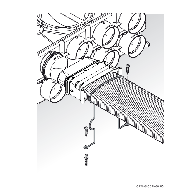
Rys. 104 FKV 140-1 + FK 140
