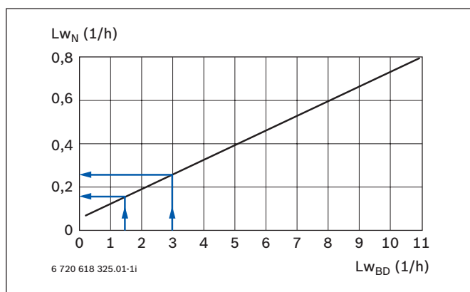
Rys. 1 Przeliczenie wymiany powietrza wg metody kontroli szczelności powietrznej Blower Door
