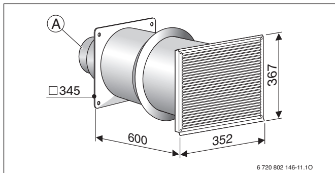
Rys. 85 Wymiary przepustu ściennego WG 160-2 (w mm)
