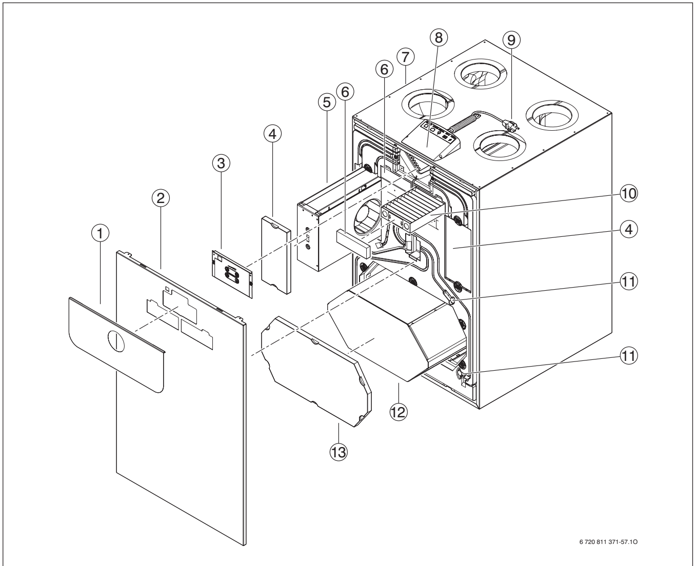
Rys. 27 Urządzenie wentylacji mieszkania LP 350-2
