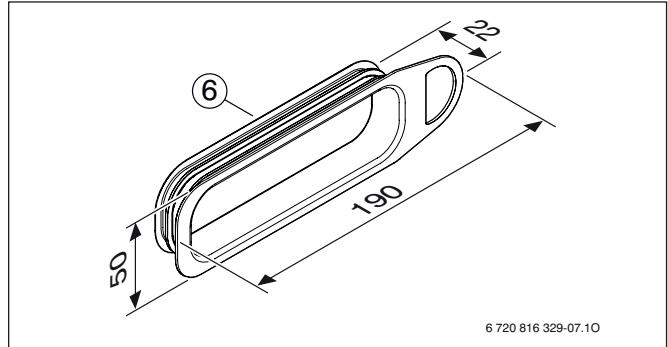
Rys. 133 FKS 140
