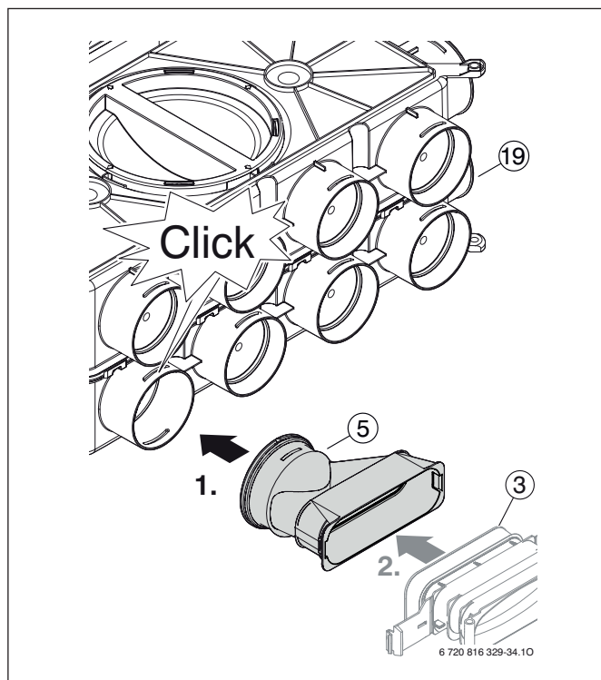
Rys. 103 FKV 140-1 + VK 160
