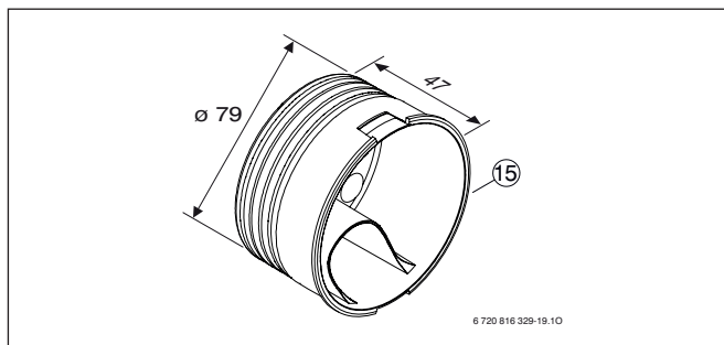
Rys. 115 RRS 75
