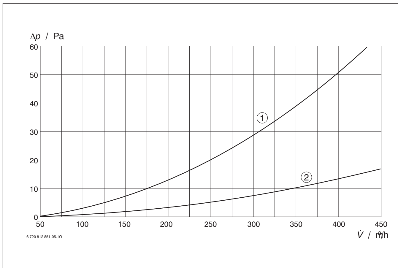
Rys. 55 Charakterystyka straty ciśnienia/strumienia objętości
