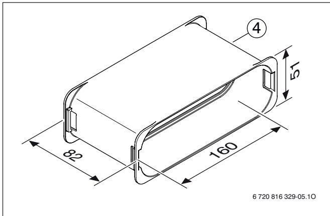
Rys. 132 FKV 140-2
