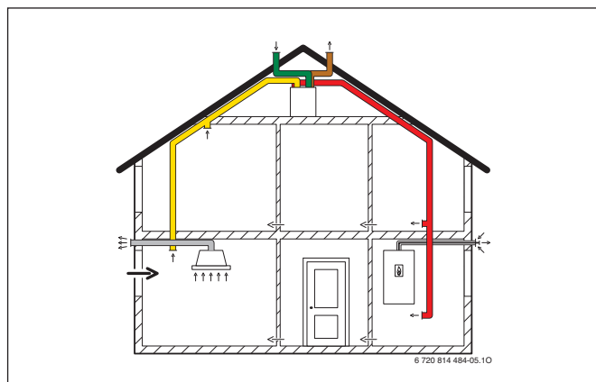
Rys. 175 AerastarComfort LP ...-2 i wyciąg kuchenny w trybie powietrza odprowadzanego
