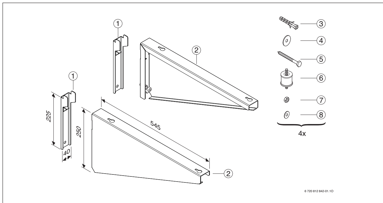
Rys. 23 Zakres dostawy
