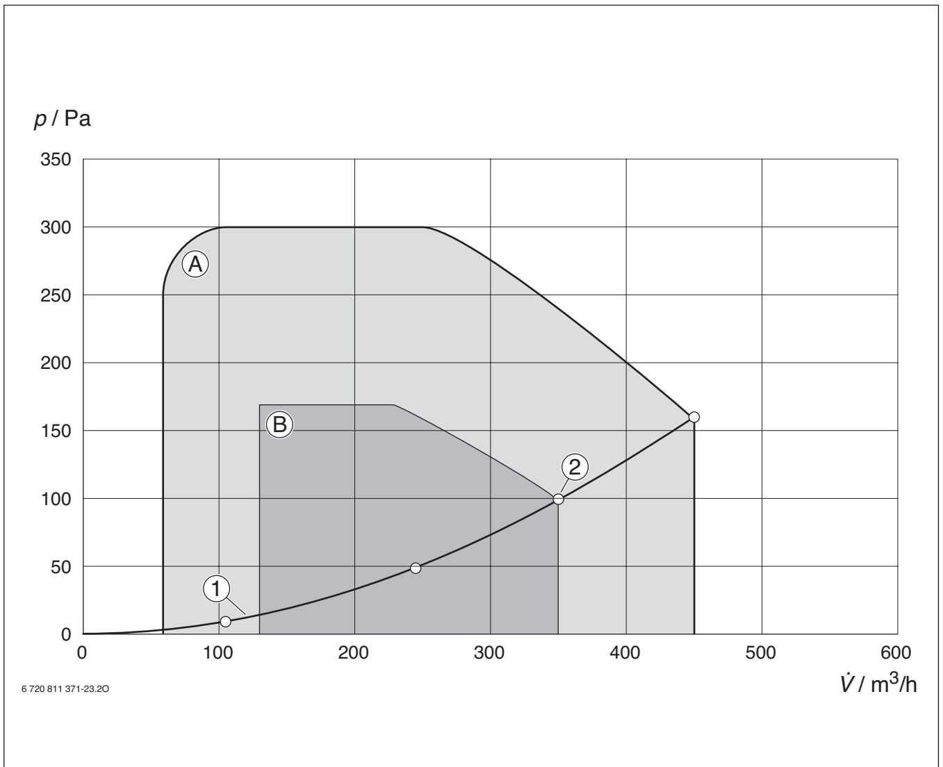
Rys. 35 Charakterystyki wzrostu ciśnienia/strumienia objętości LP 350-2
