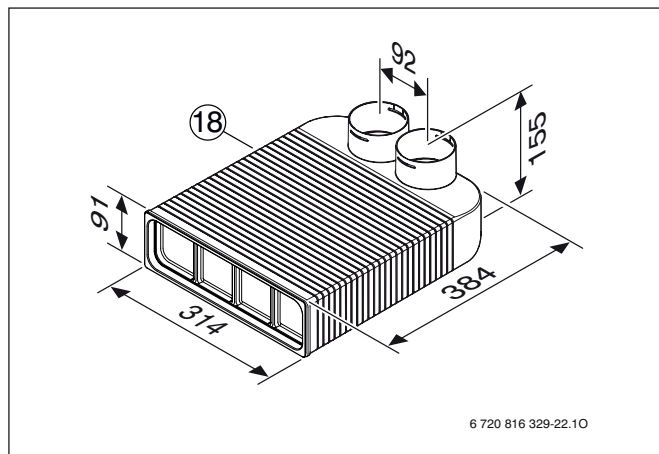
Rys. 136 RRU 75-2
