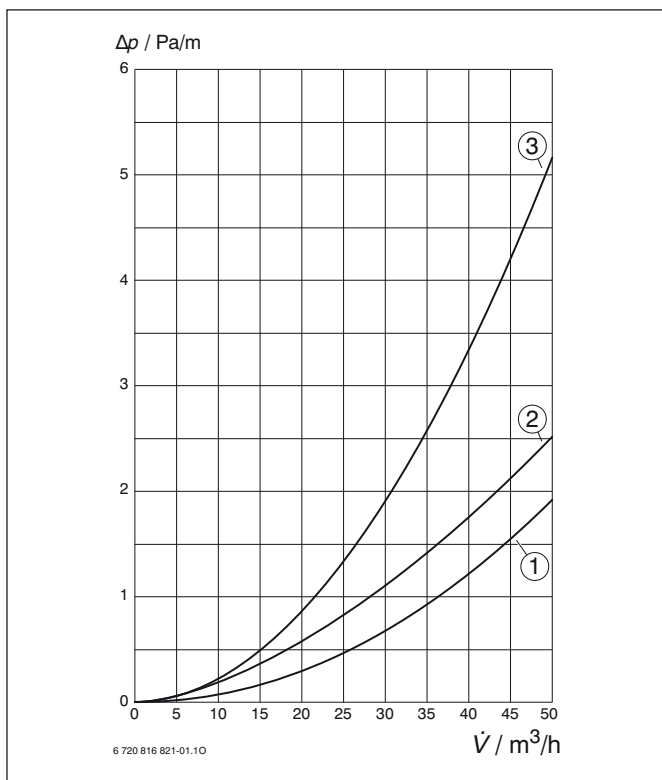
Rys. 119 Strata ciśnienia w kanale płaskim FK 140
