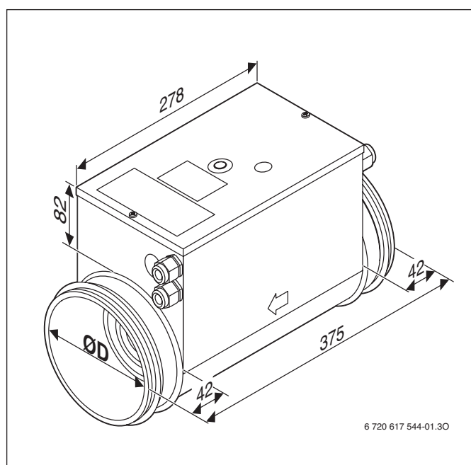
Rys. 53 Wymiary montażowe nagrzewnic HRE 125/160 (w mm)
