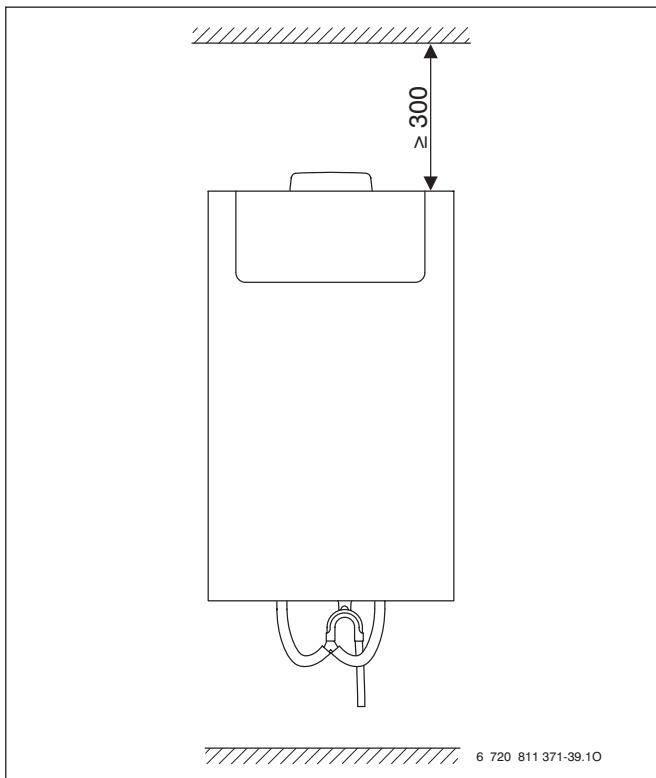
Rys. 31 Minimalne wymiary montażowe LP 140-2
