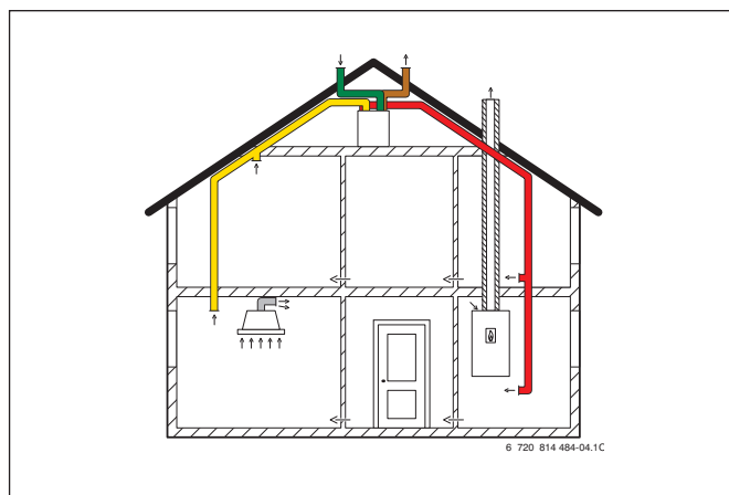
Rys. 174 AerastarComfort LP ...-2 i palenisko zależne od powietrza w pomieszczeniu
