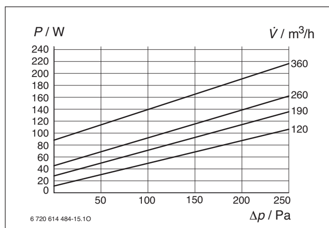
Rys. 38 Charakterystyki AerastarComfort LP 350-2
