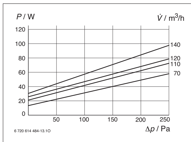
Rys. 36 Charakterystyki AerastarComfort LP 140-2
