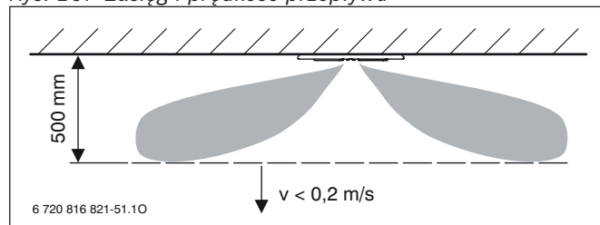
Rys. 167 Zasięg i prędkość przepływu
