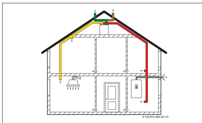
Rys. 173 AerastarComfort LP ...-2 i palenisko niezależne od powietrza w pomieszczeniu
