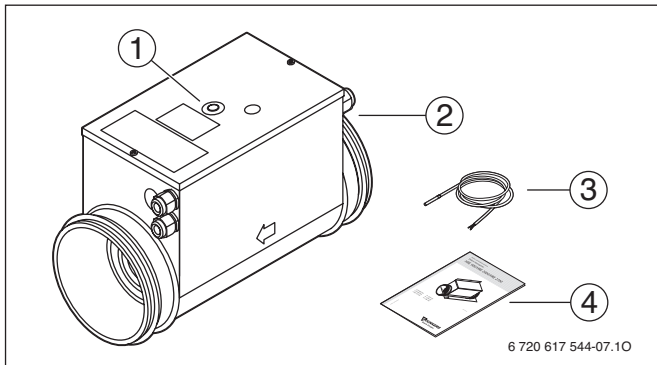
Rys. 50 Zakres dostawy
