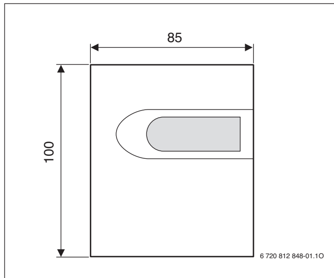
Rys. 49 Wymiary (w mm)
