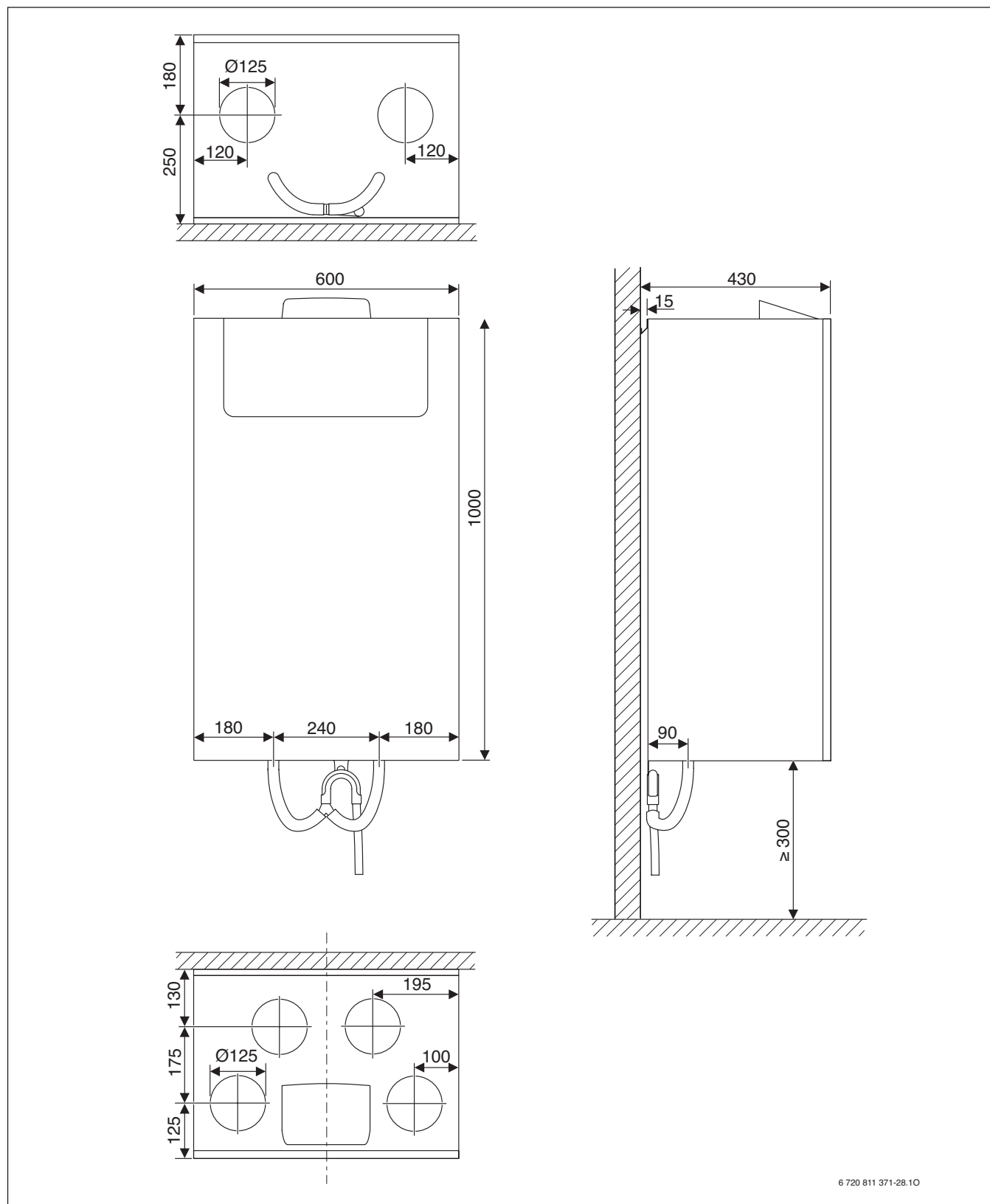
Rys. 28 AerastarComfort LP 140-2 (wymiary w mm)
