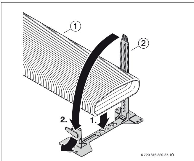
Rys. 118 Montaż kanału płaskiego
