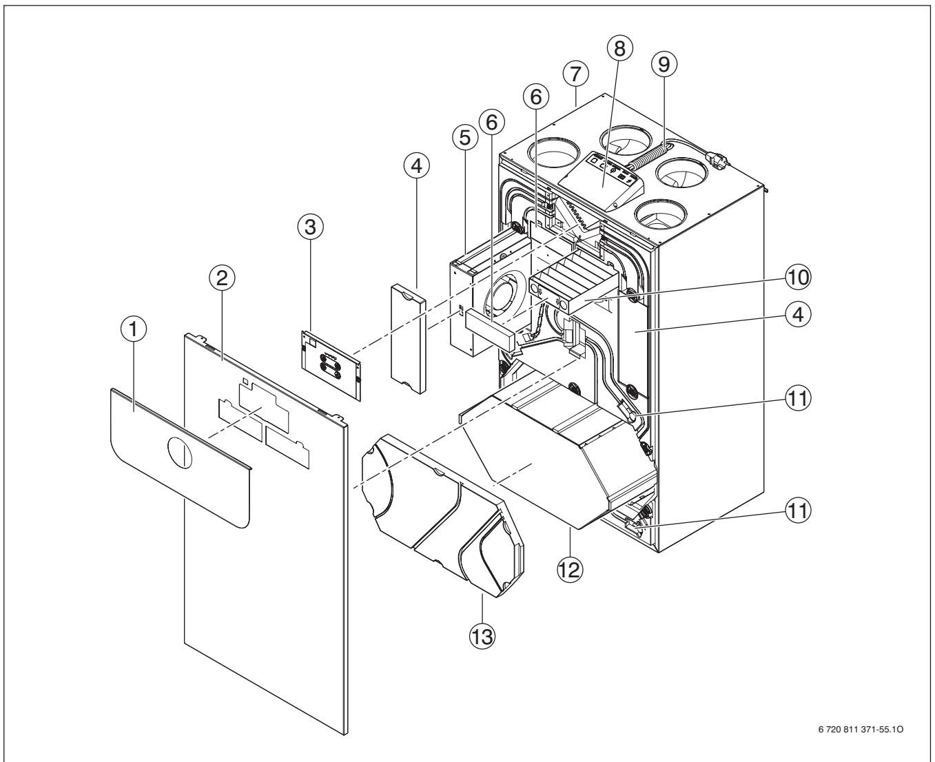
Rys. 25 Urządzenie wentylacji mieszkania AerastarComfort LP 140-2
