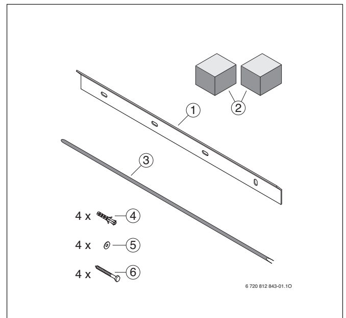
Rys. 21 Zakres dostawy
