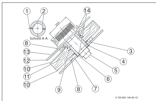
Rys. 82 Szkic przekroju – montaż przepustu dachowego DDF 160/1 (wymiary w mm)
