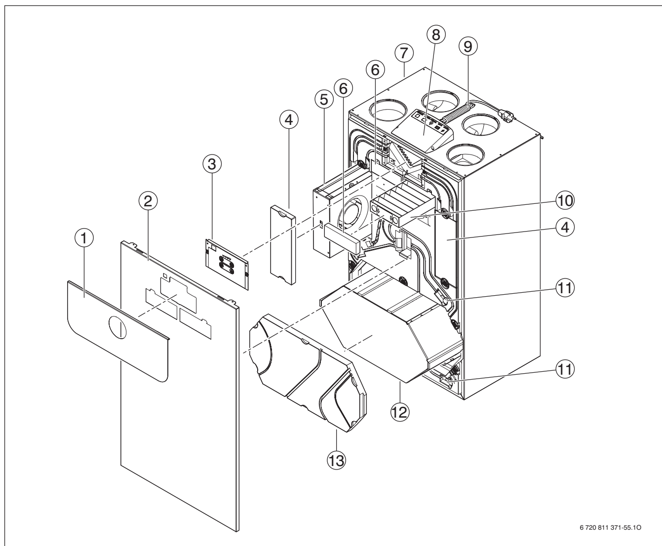
Rys. 26 Urządzenie wentylacji mieszkania LP 230-2
