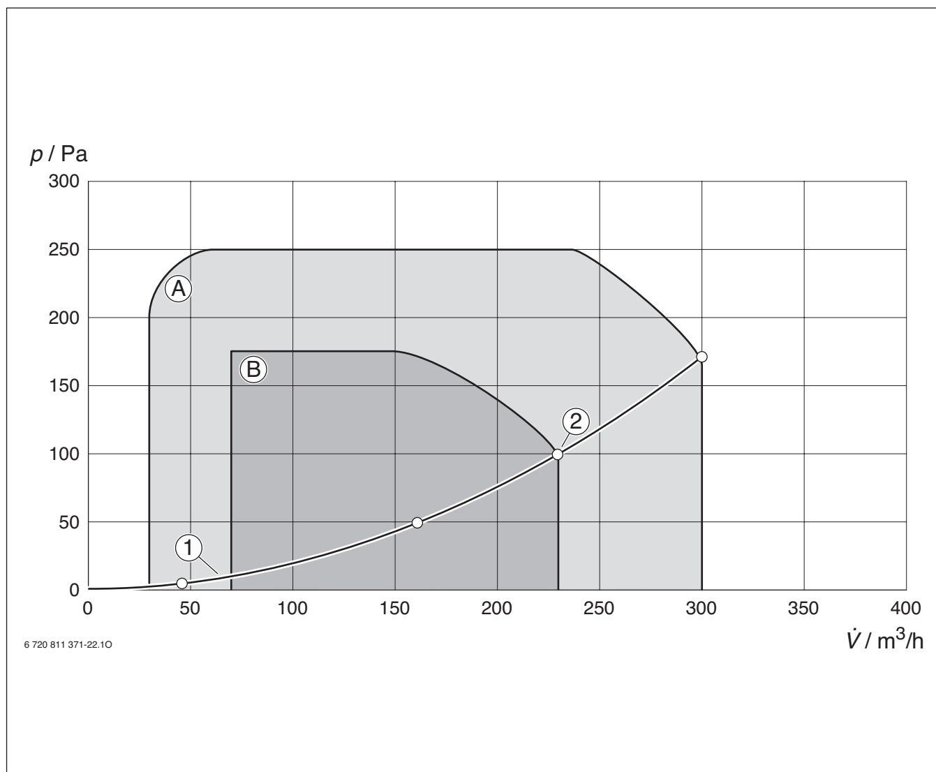
Rys. 34 Charakterystyki wzrostu ciśnienia/strumienia objętości LP 230-2
