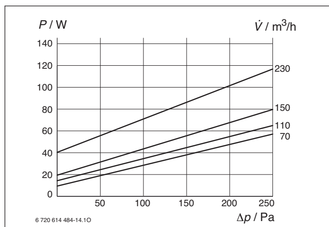
Rys. 37 Charakterystyki AerastarComfort LP 230-2
