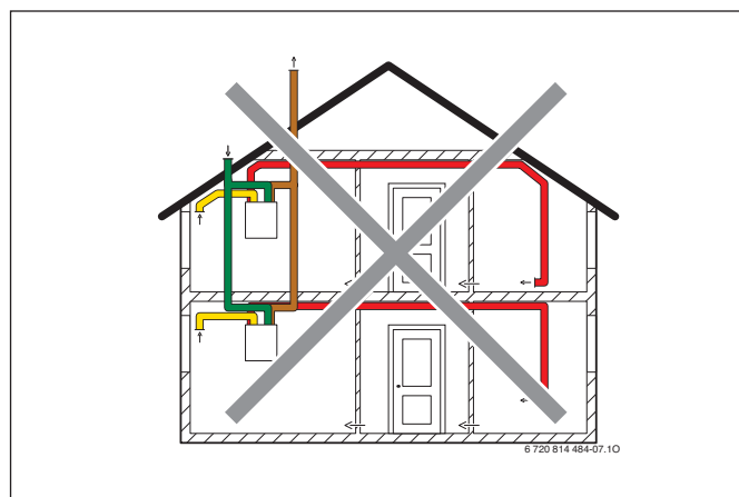
Rys. 177 AerastarComfort LP ...-2 i przewody zbiorcze powietrza wywiewanego/zewnętrznego
