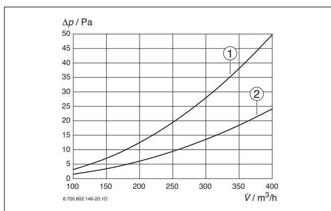
Rys. 83 Straty ciśnienia w przepuscie dachowym DDF 160/1 przyłączy DN 160
