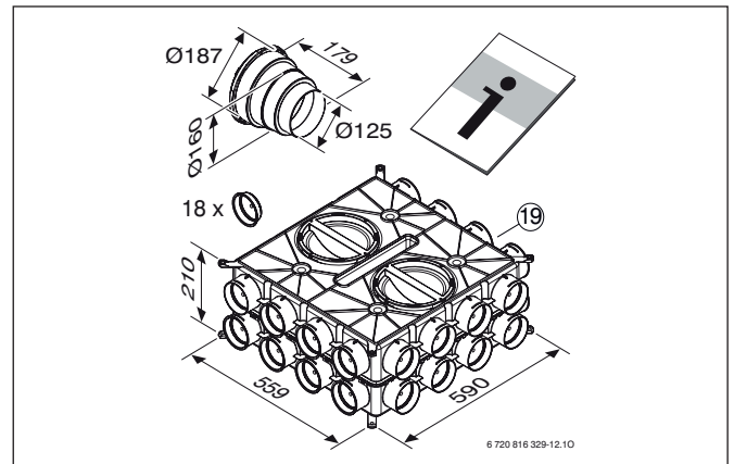
Rys. 97 VK 160 [7] VK 160
