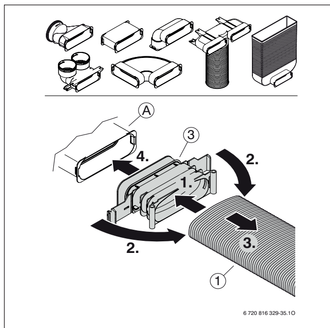
Rys. 131 FK 140 + FKV.../FKB.../FKU.../RRB 75
