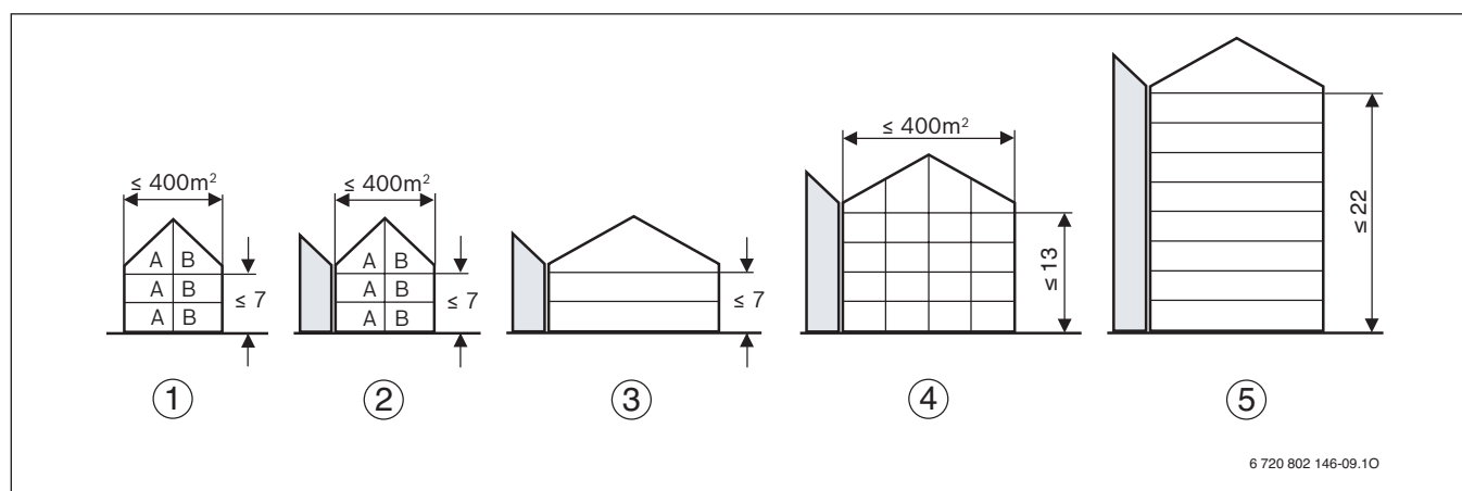
Rys. 179 Klasy budynków (wymiary w m)
