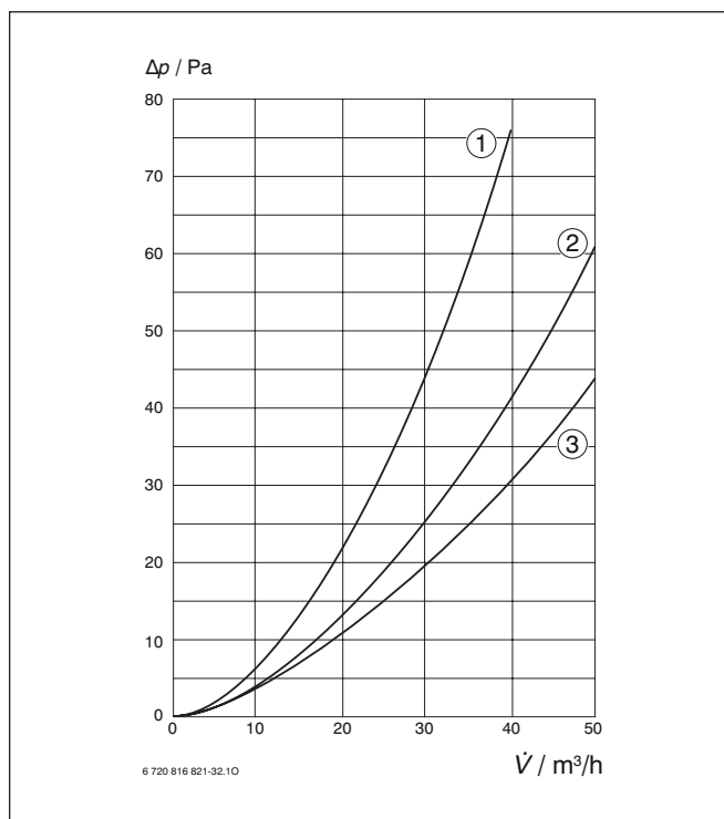
Rys. 164 Strata ciśnienia
