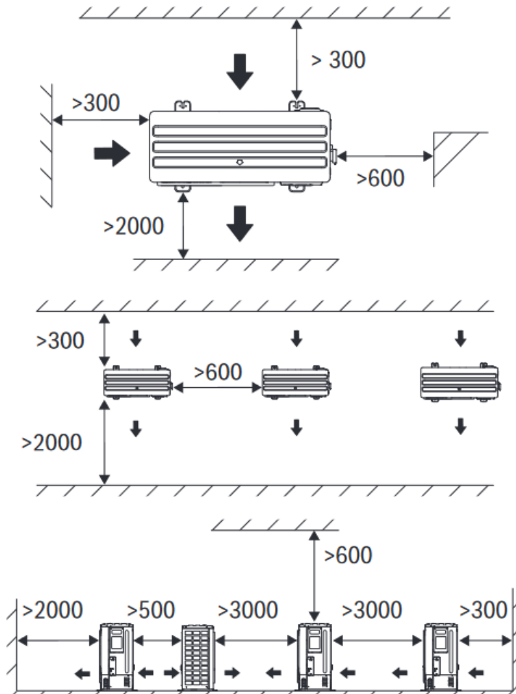
Fig. 2 - Distâncias mínimas de instalação (Unidades em mm)
