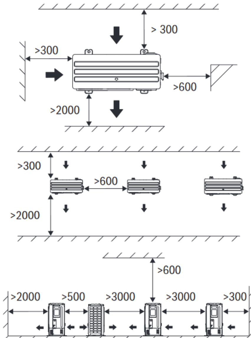
Fig. 2 - Distâncias mínimas de instalação (Unidades em mm)
