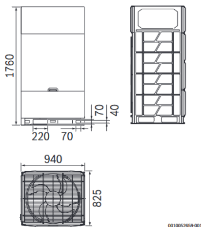
Fig. 1 – Dimensões AF5301...25 kW a AF5301...45 kW (Unidades em mm)
