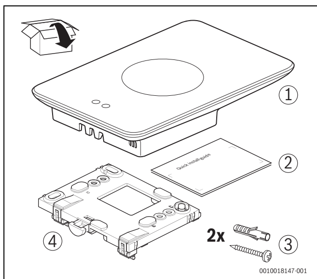
Obr. 1 Rozsah dodávky
