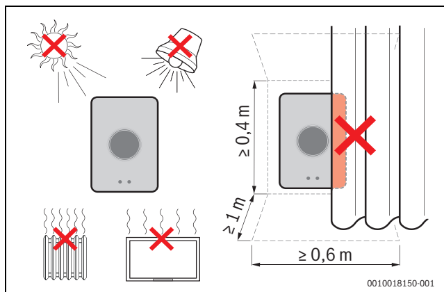
Obr. 4 Miesto inštalácie regulátora, kritériá
