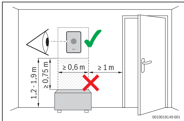
Obr. 3 Miesto inštalácie regulátora, odstup
