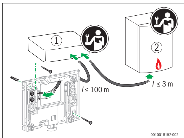
Obr. 6 Pripojenie adaptéra EasyControl
