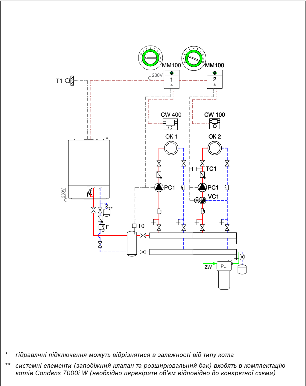
Рис. 10 Гідравлічна схема
