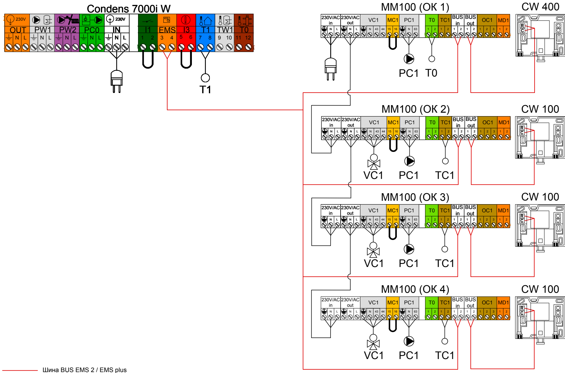
Рис. 15 Електрична схема
