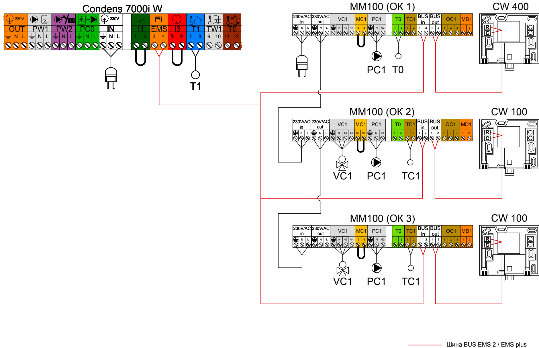
Рис. 13 Електрична схема
