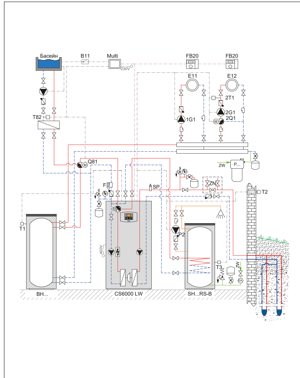
Рис. 82 Гідравлічна схема
