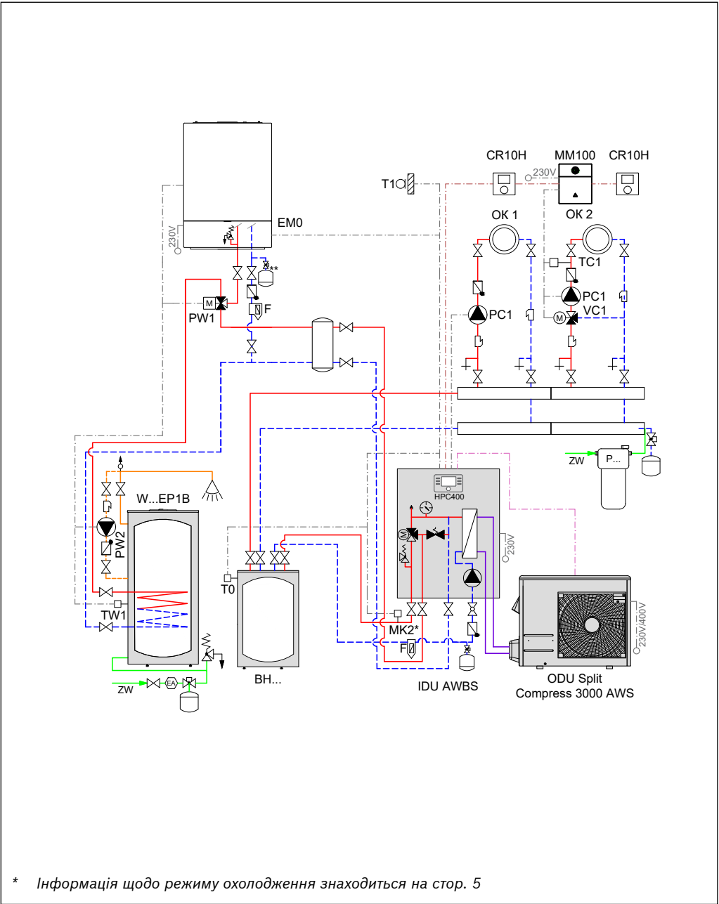
Рис. 58 Гідравлічна схема
