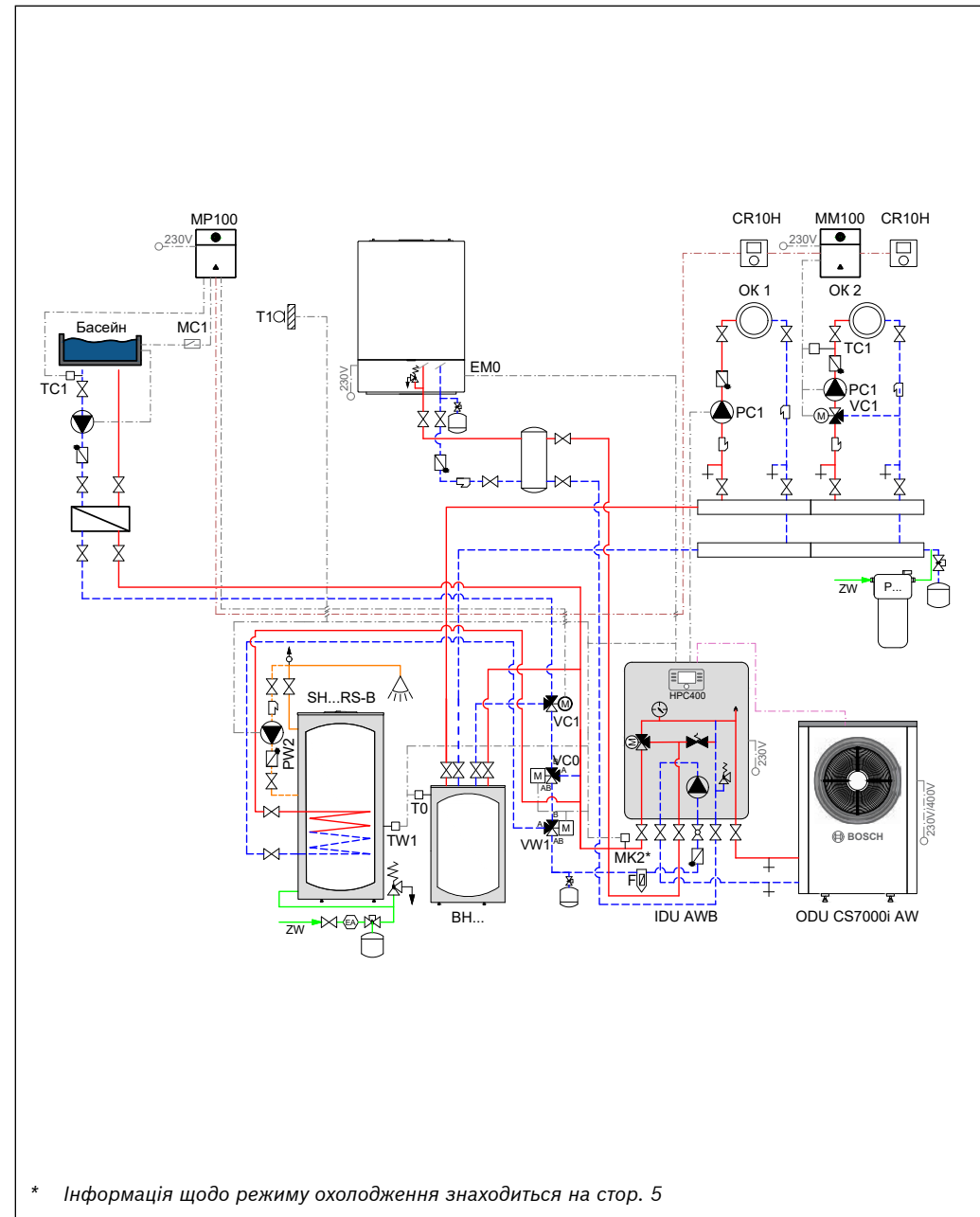
Рис. 56 Гідравлічна схема
