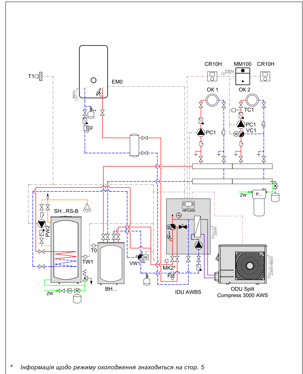
Рис. 66 Гідравлічна схема
