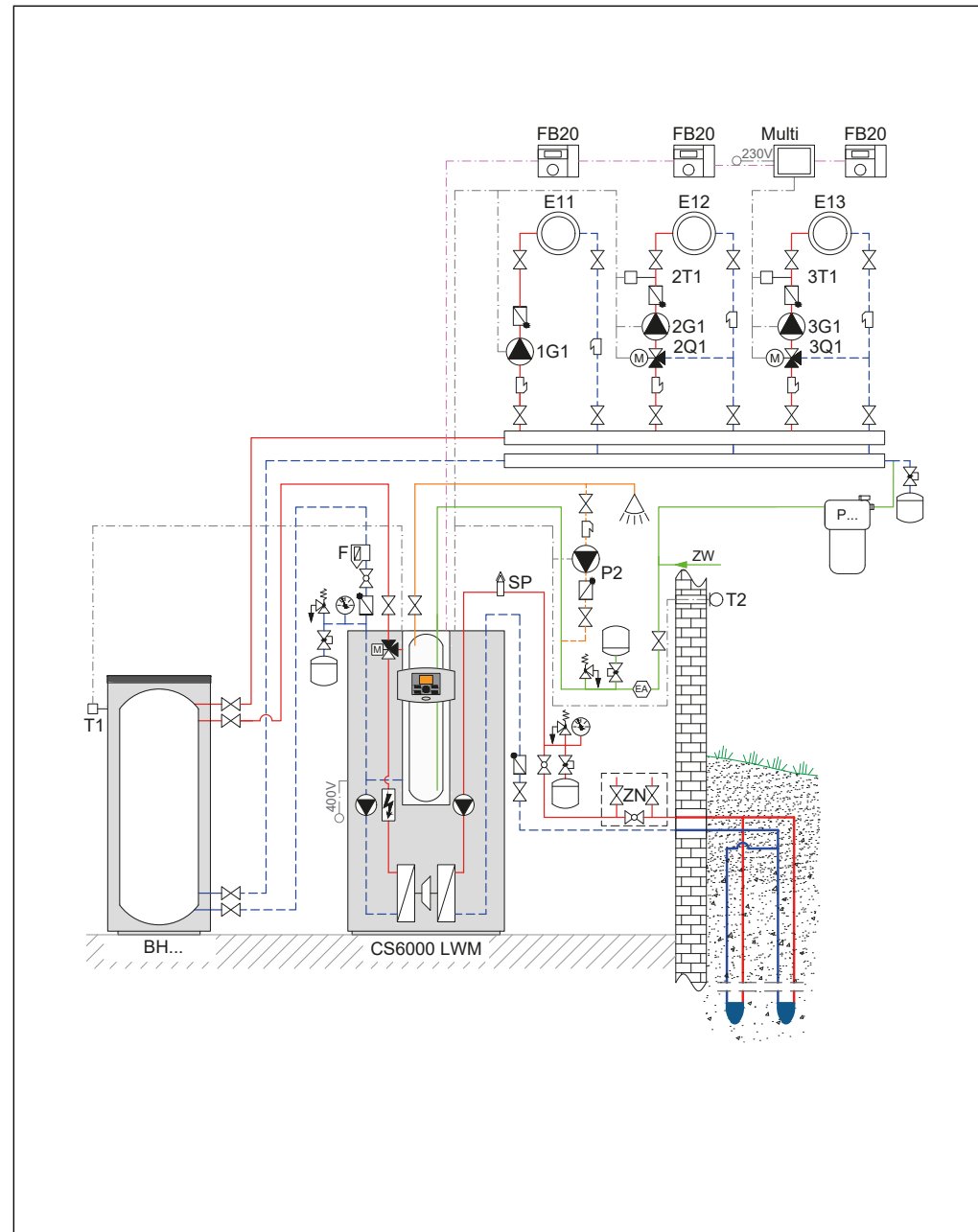
Рис. 72 Гідравлічна схема
