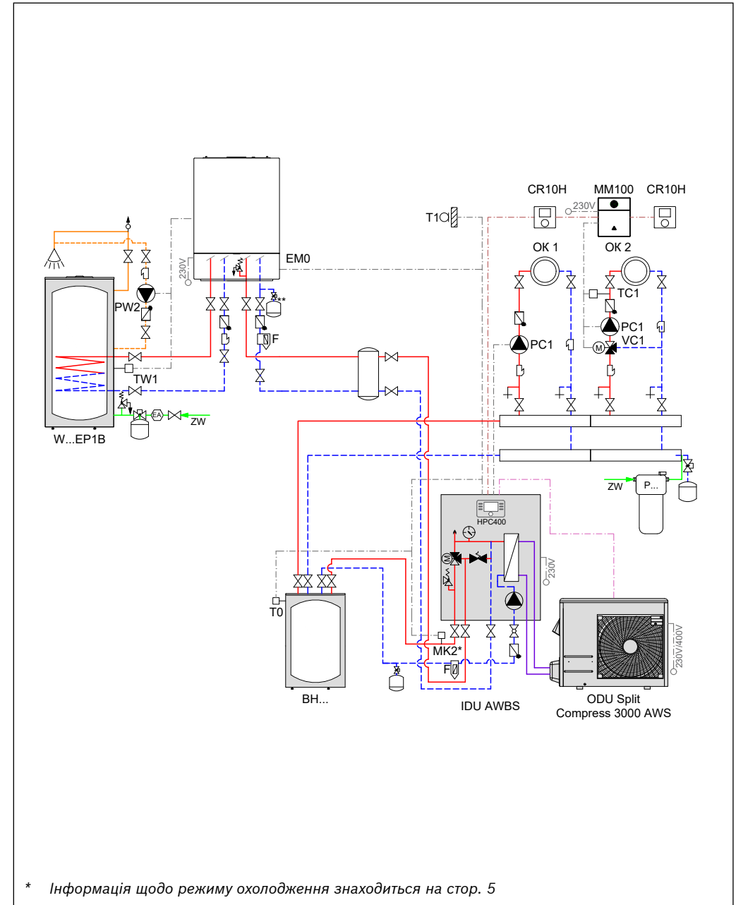
Рис. 62 Гідравлічна схема
