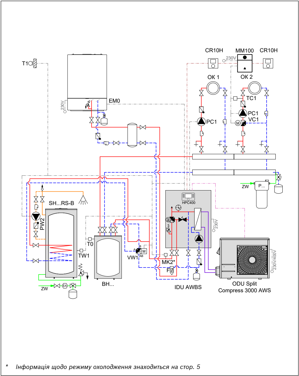
Рис. 46 Гідравлічна схема
