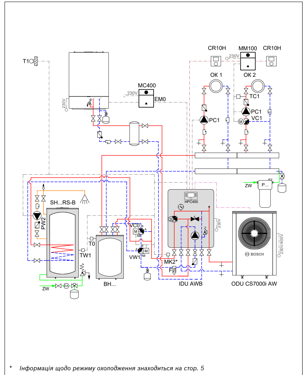
Рис. 52 Гідравлічна схема
