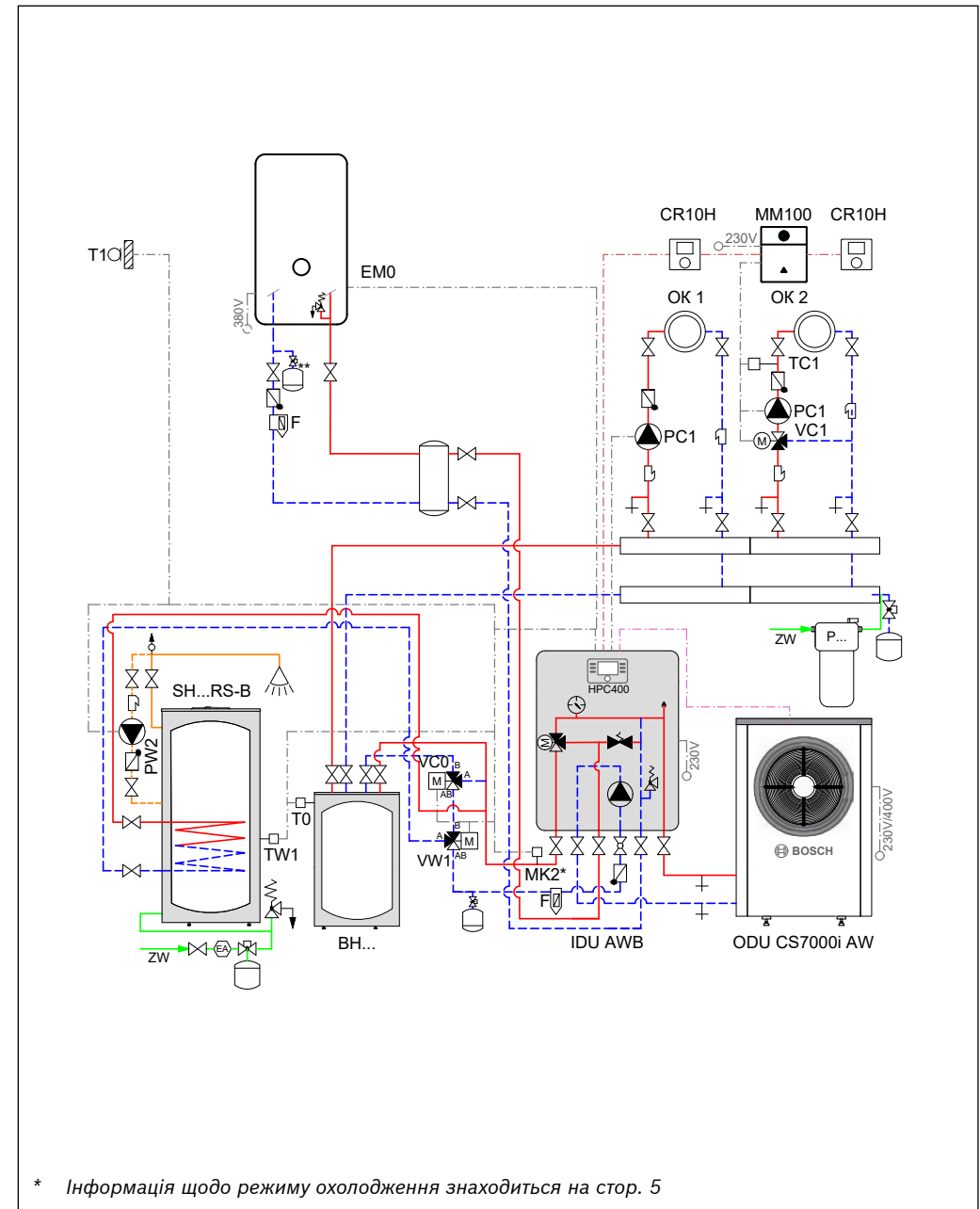
Рис. 68 Гідравлічна схема
