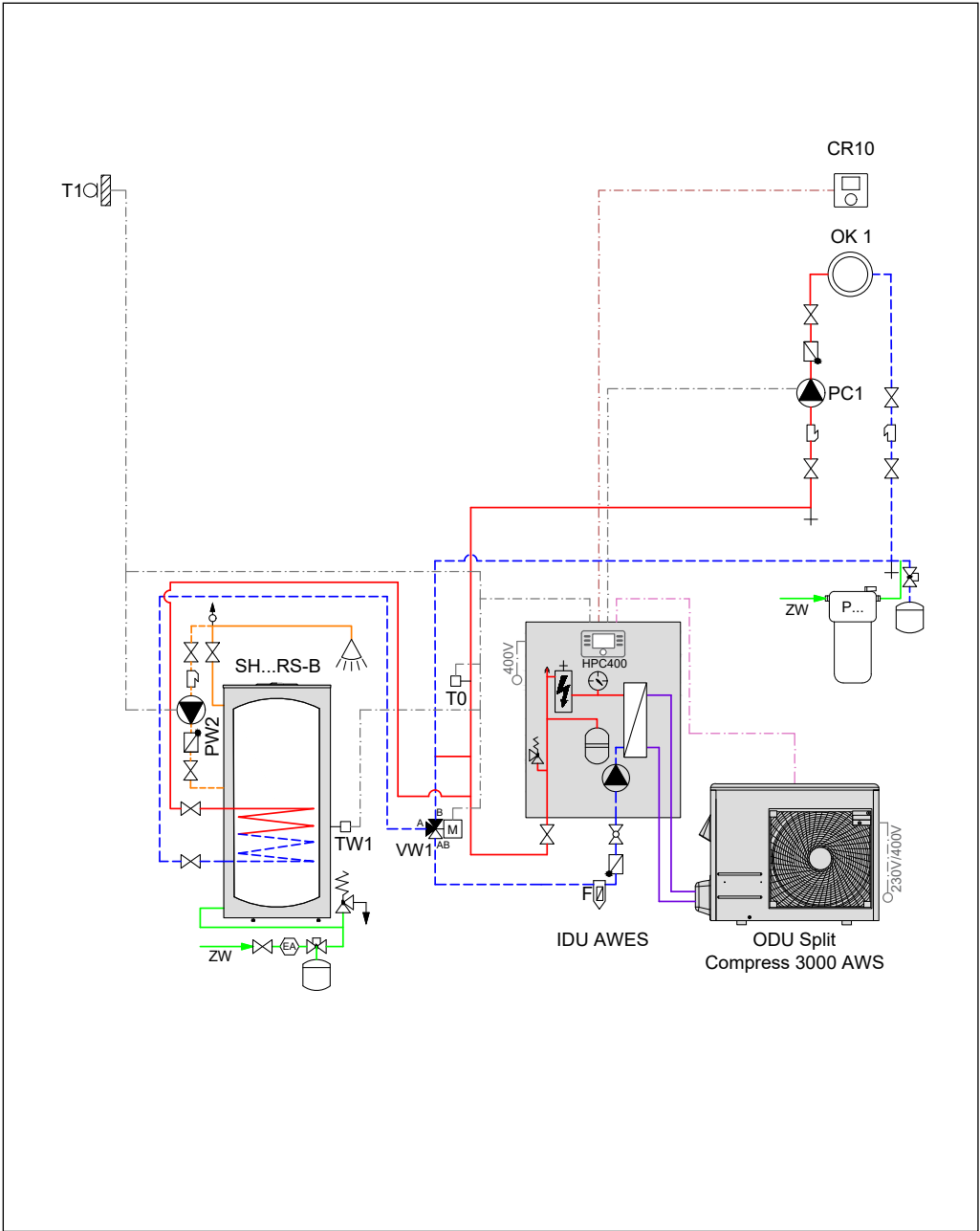
Рис. 38 Гідралічна схема
