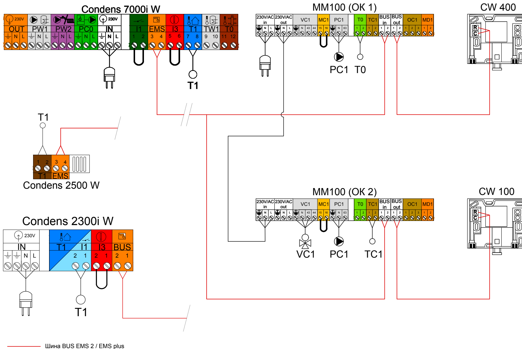
Рис. 5 Електрична схема
