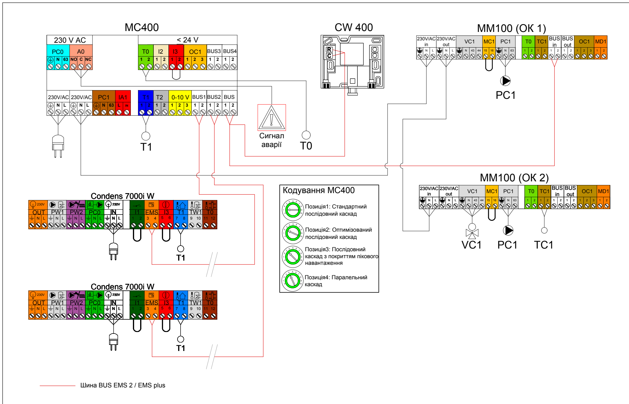
Рис. 25 Електрична схема
