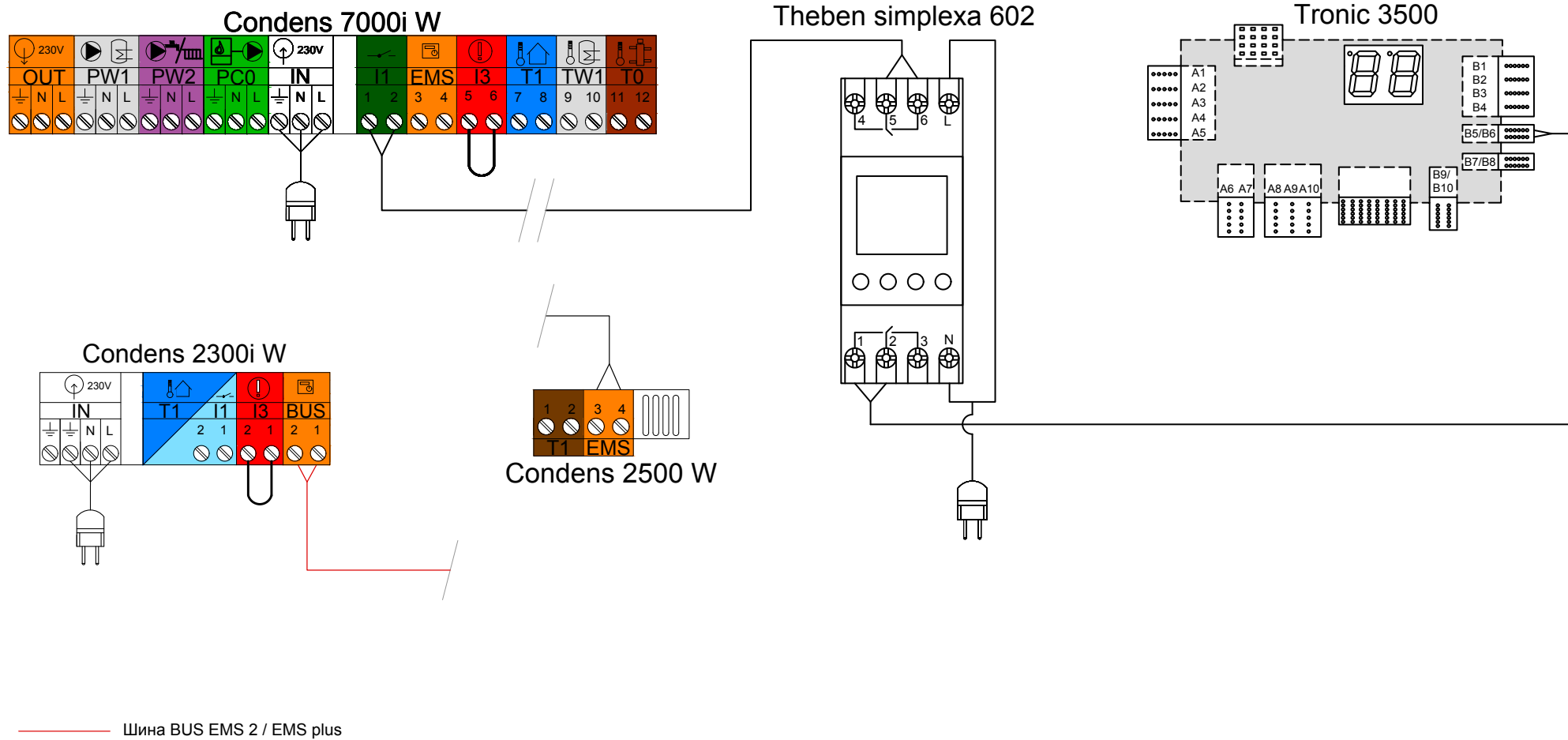
Рис. 37 Електрична схема
