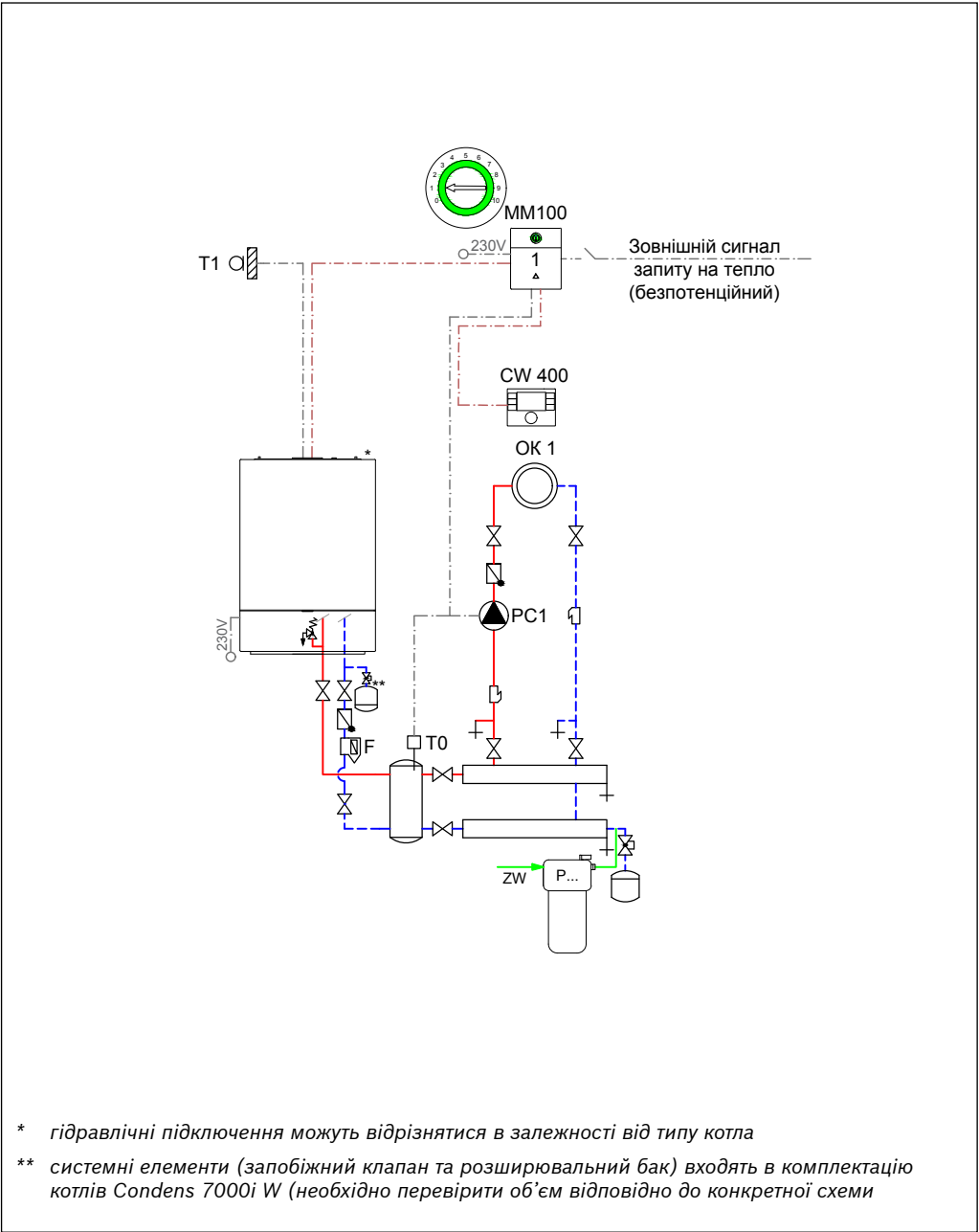
Рис. 22 Гідравлічна схема
