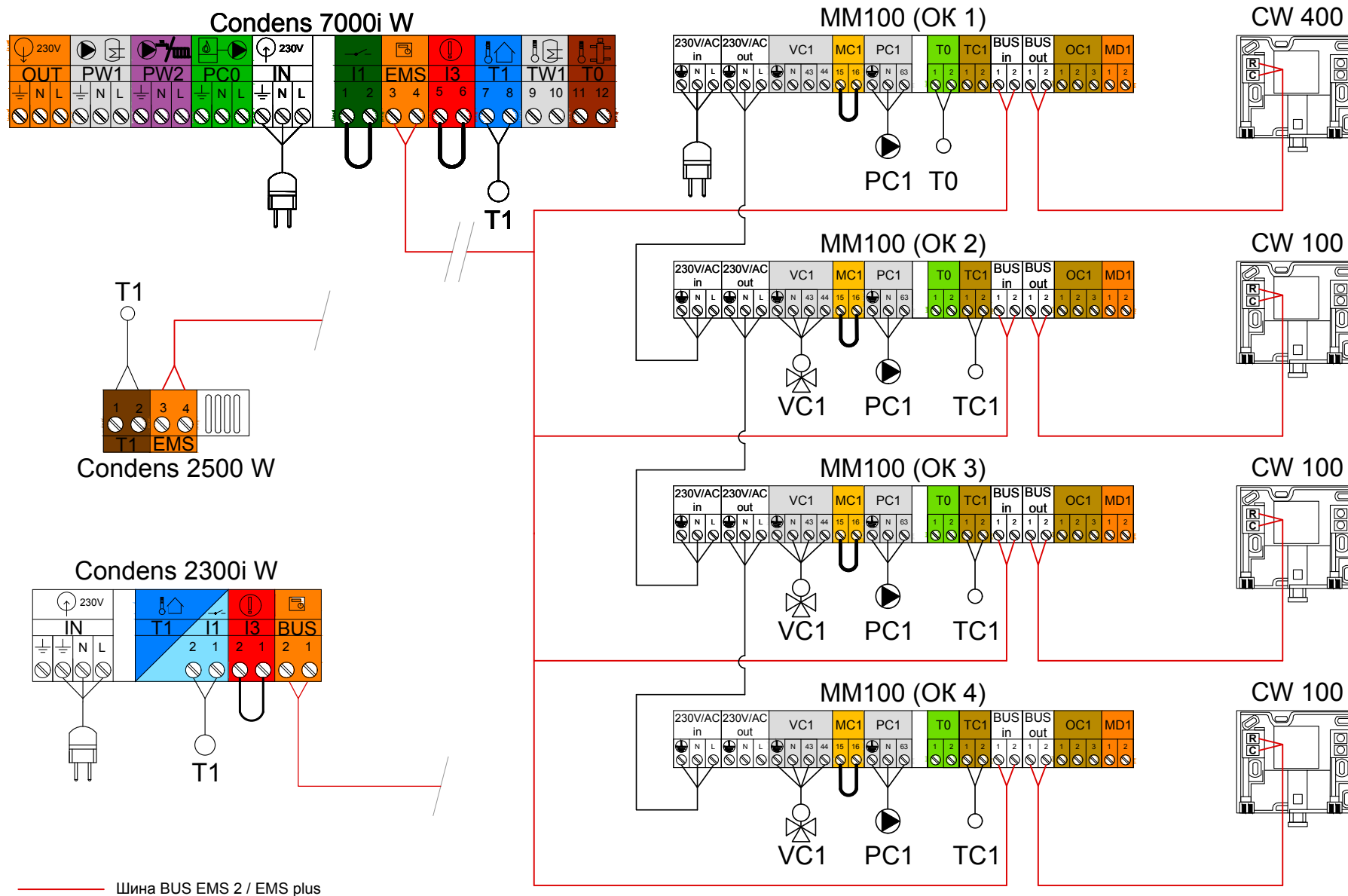
Рис. 9 Електрична схема
