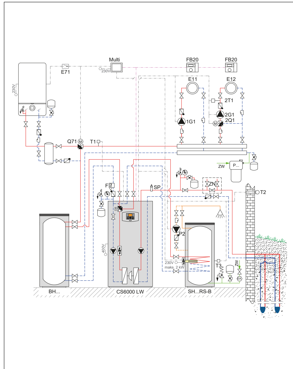
Рис. 80 Гідравлічна схема
