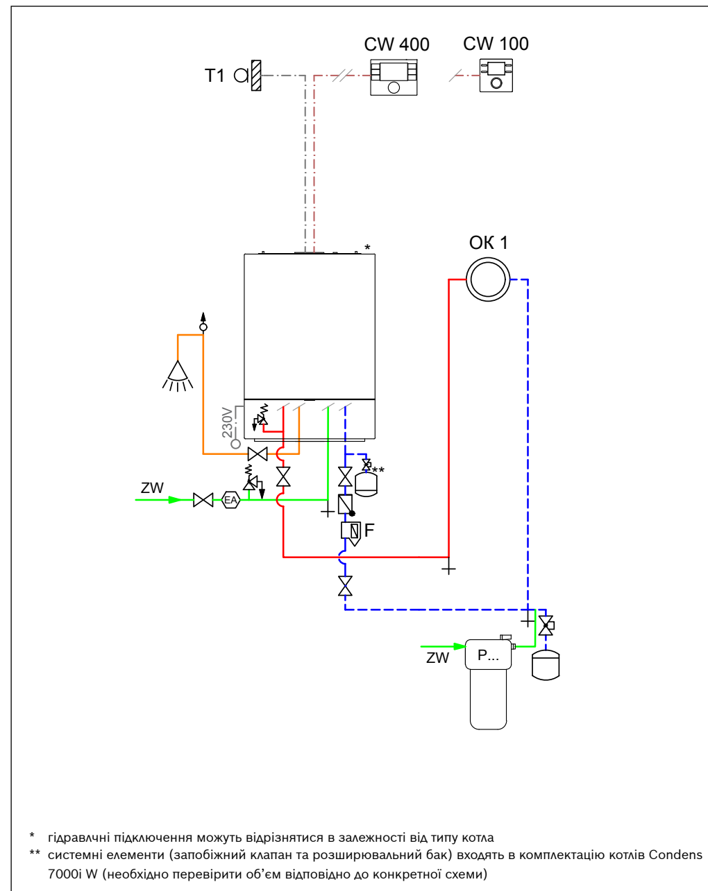
Рис. 2 Гідравлічна схема
