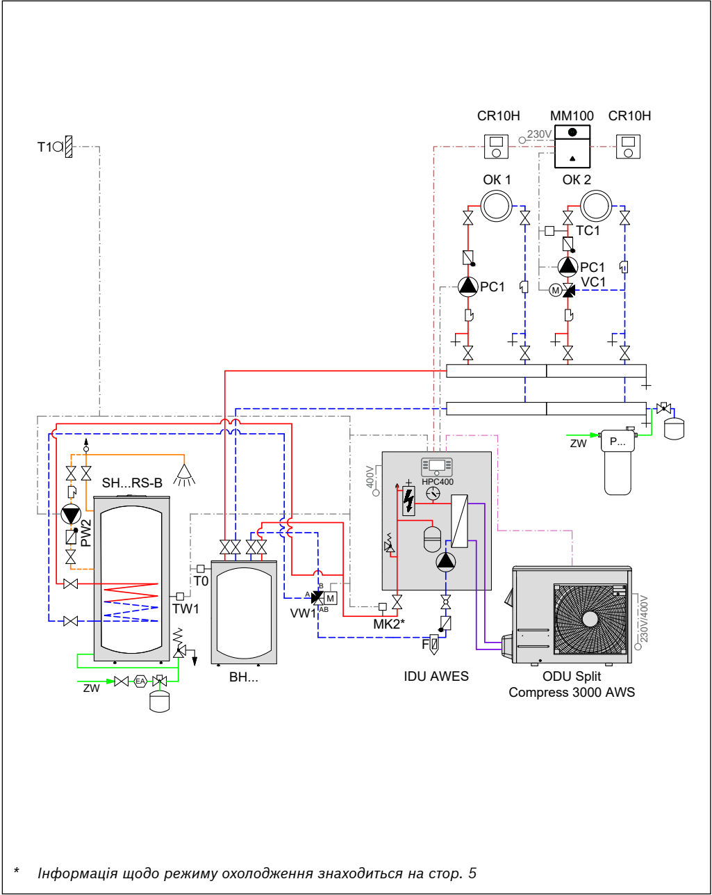
Рис. 42 Гідравлічна схема
