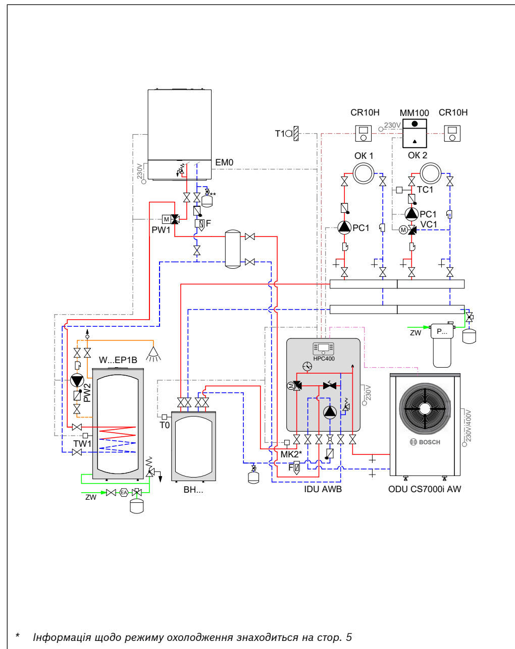
Рис. 60 Гідравлічна схема
