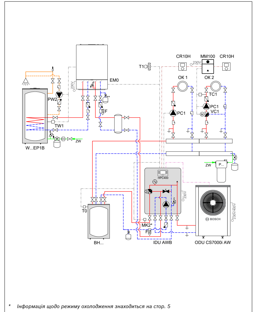
Рис. 64 Гідравлічна схема
