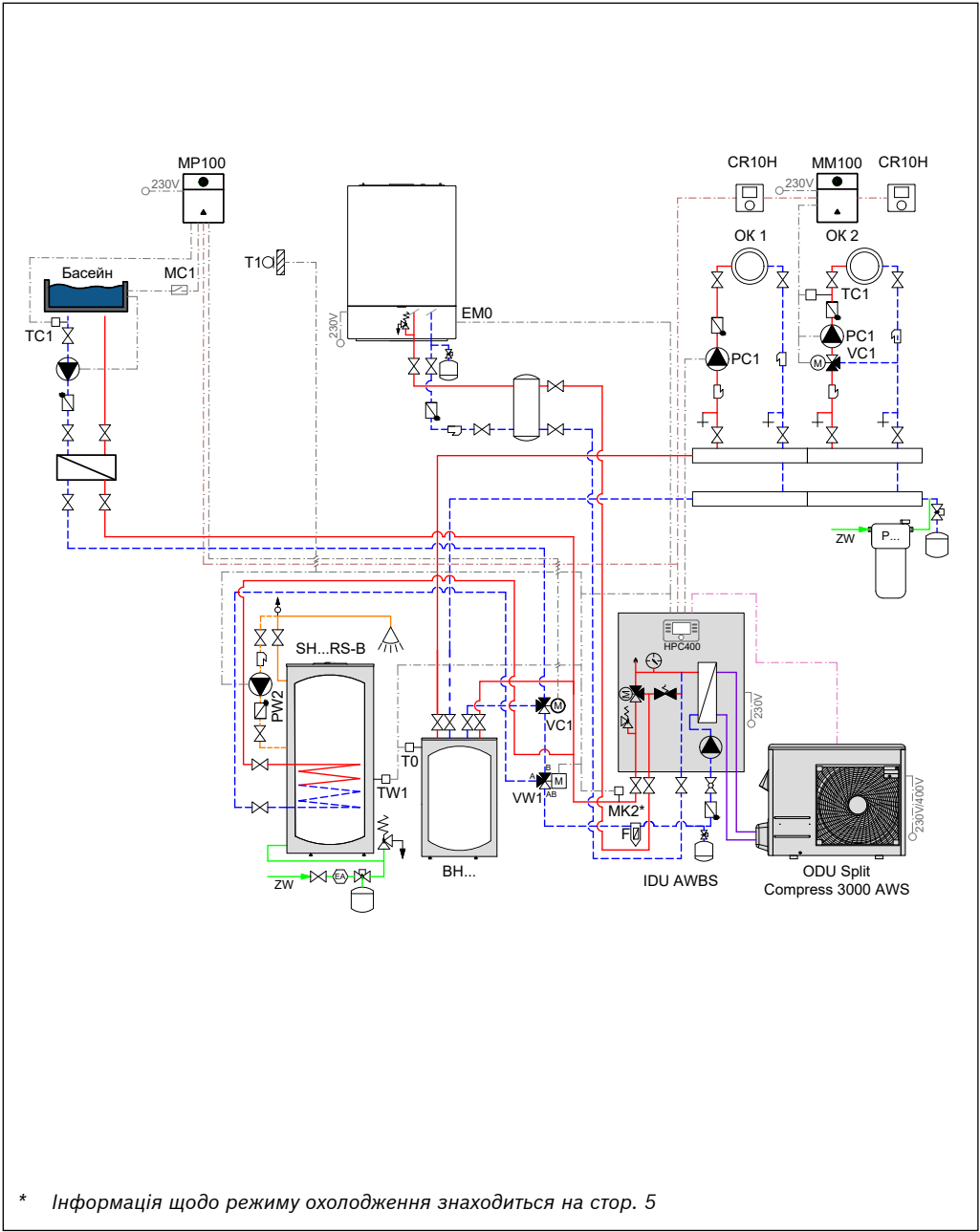
Рис. 54 Гідравлічна схема
