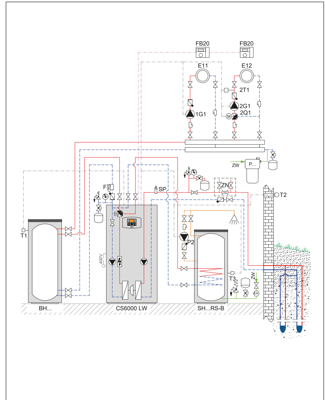
Рис. 74 Гідравлічна схема
