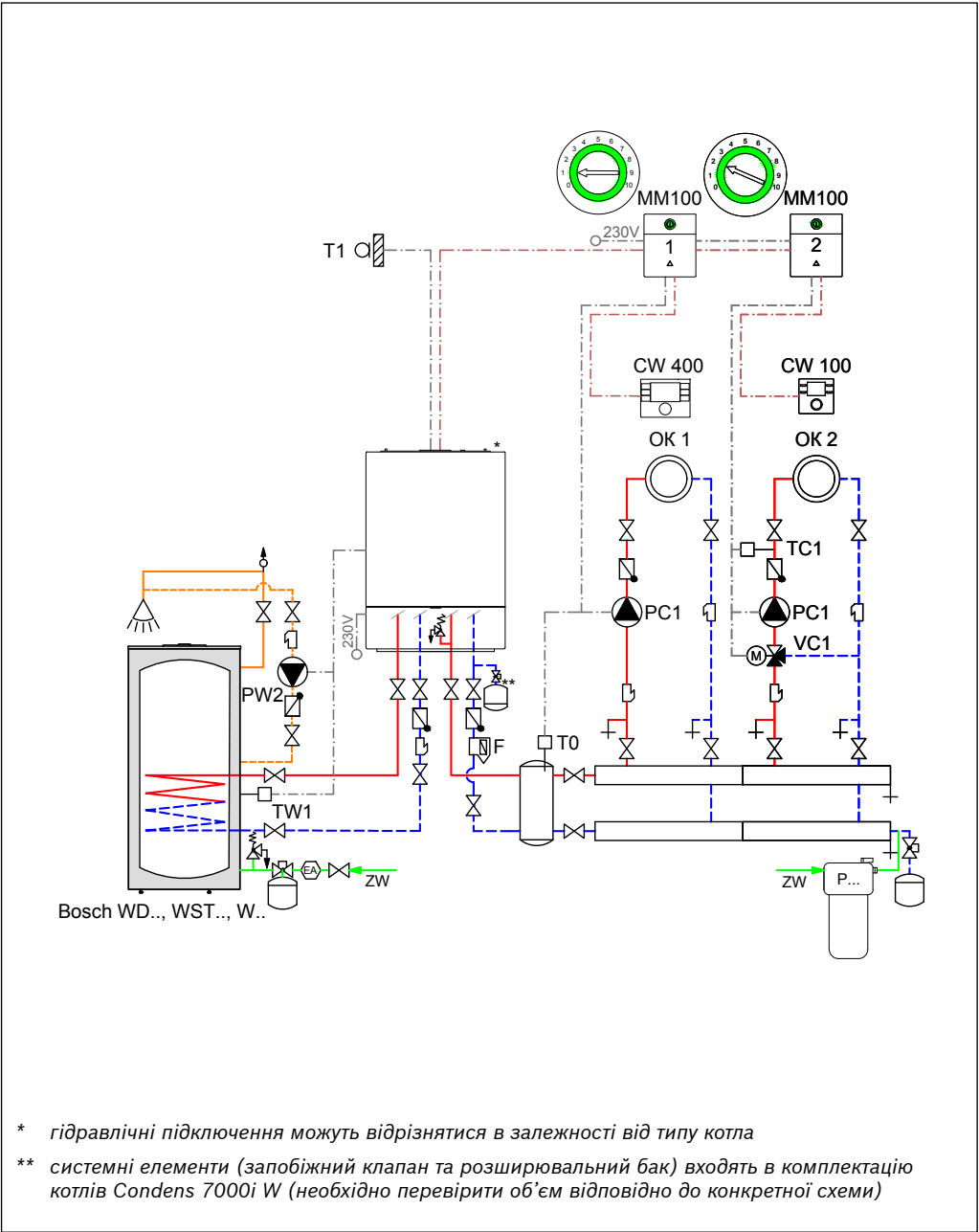
Рис. 18 Гідравлічна схема
