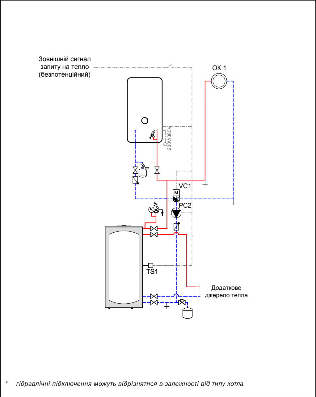
Рис. 34 Гідравлічна схема
