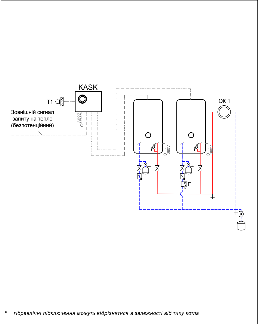
Рис. 32 Гідрравлічна схема
