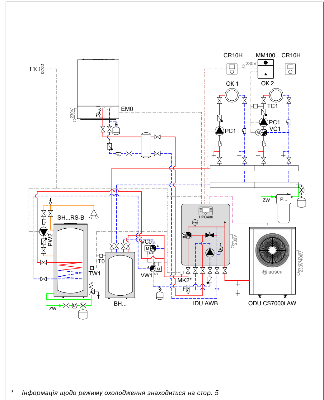
Рис. 48 Гідравлічна схема
