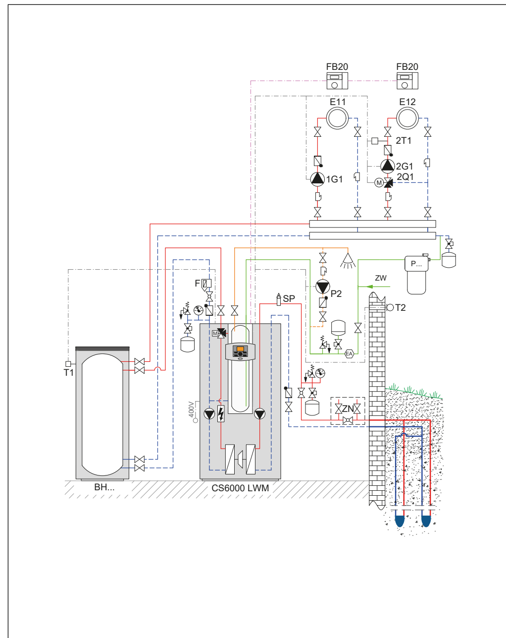
Рис. 70 Гідравлічна схема
