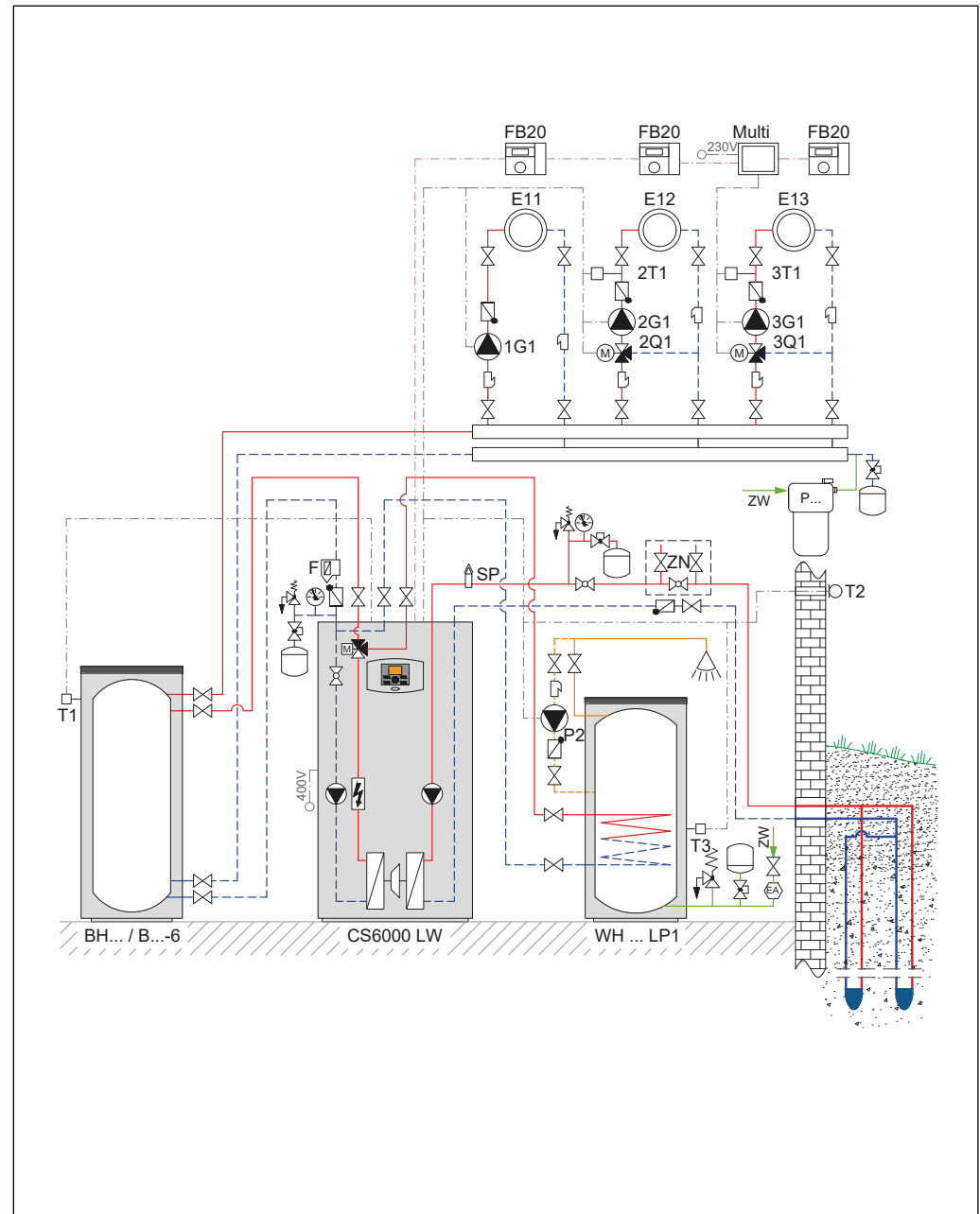
Рис. 76 Гідравлічна схема
