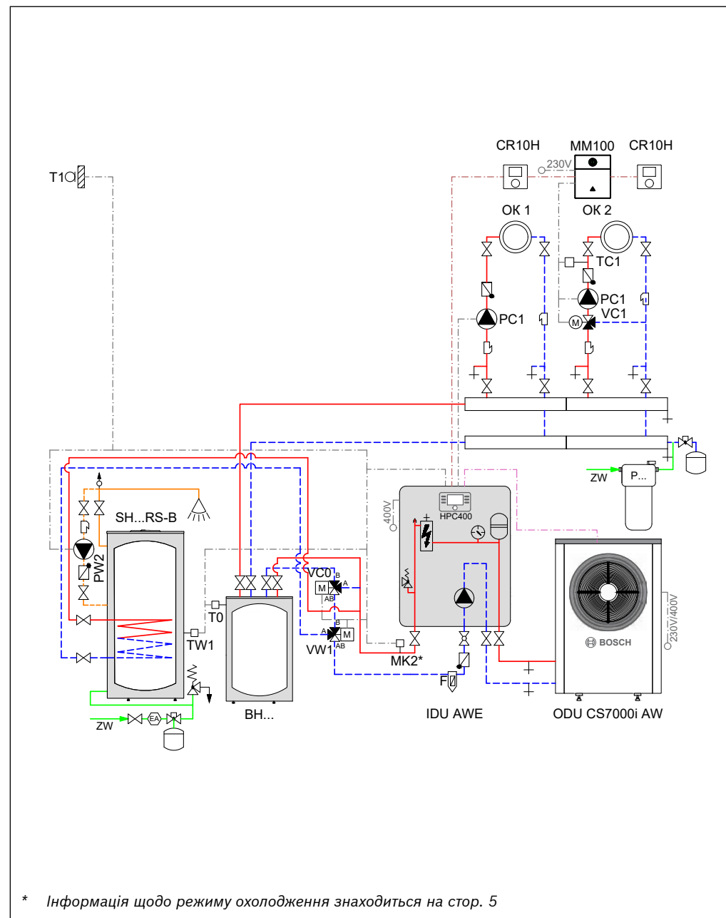
Рис. 44 Гідравлічна схема
