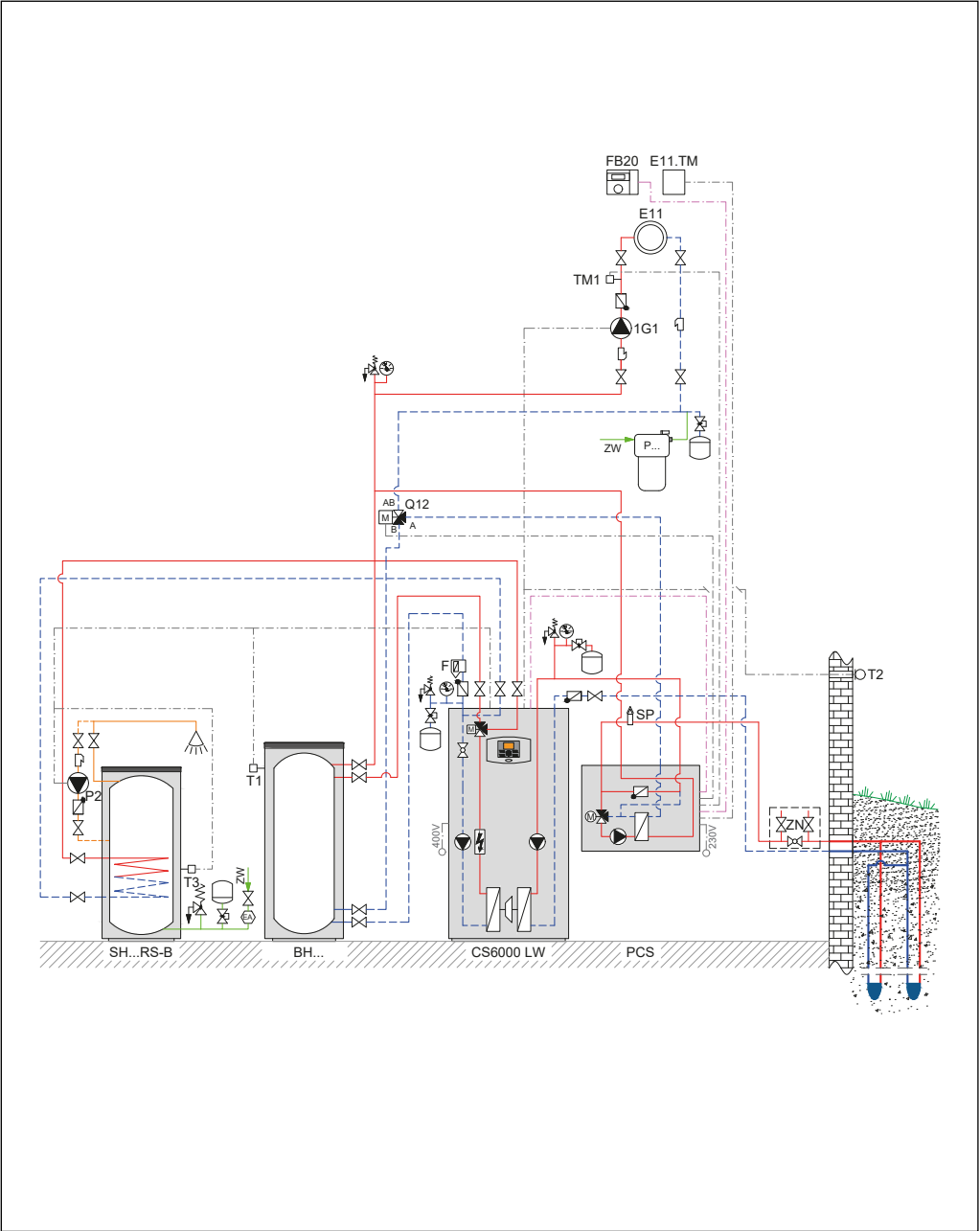
Рис. 84 Гідравлічна схема
