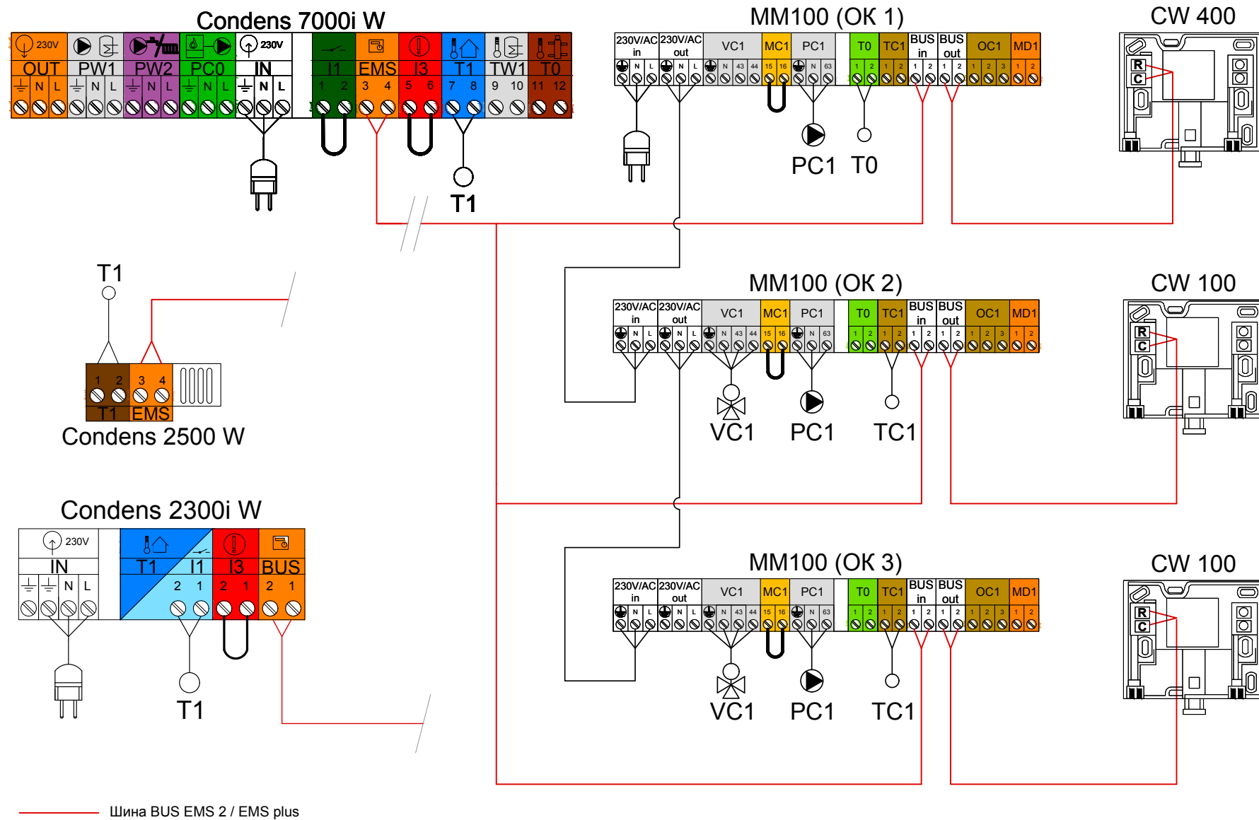
Рис. 7 Електрична схема
