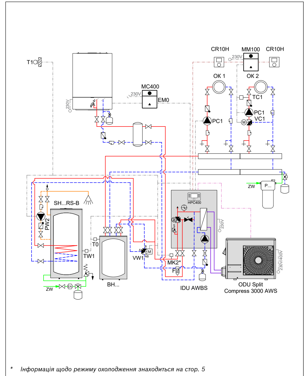
Рис. 50 Гідравлічна схема
