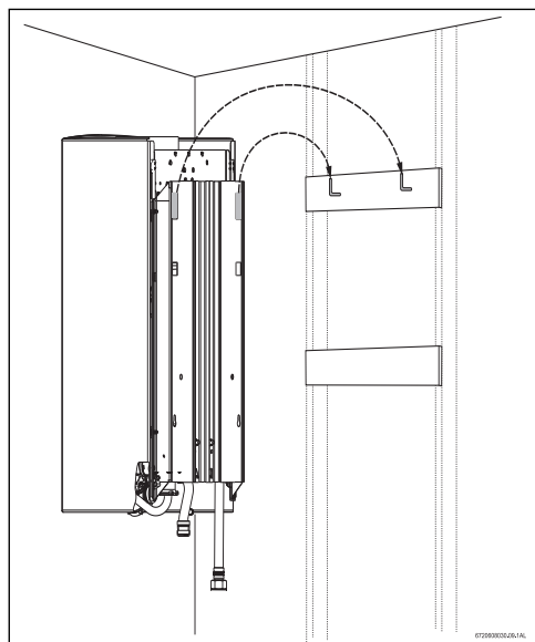
Fig. 8 Accrochage du chauffe-eau au mur
