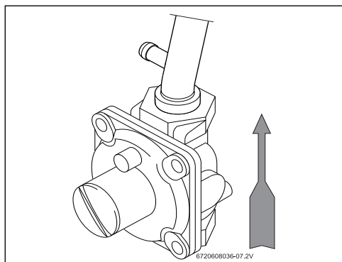
Fig. 12 Installation du détendeur de gaz
