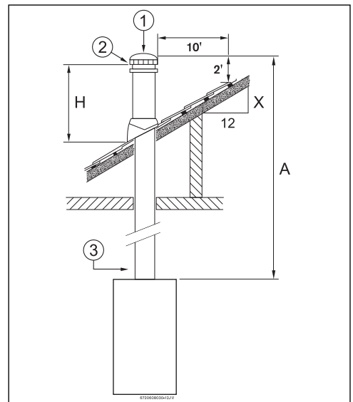
Fig. 10 Toit en pente
