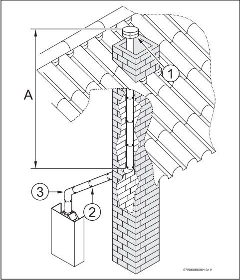
Fig. 11 Cheminée en maçonnerie
