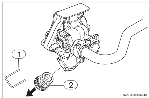
Fig. 24 Emplacement du bouchon de vidange et du filtre
