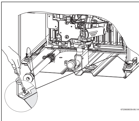
Fig. 6 Retrait du capot avant
