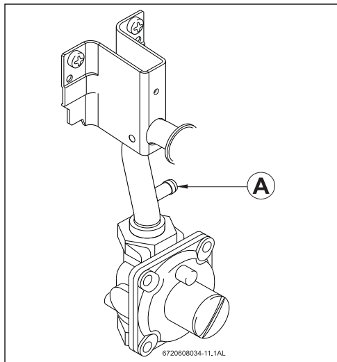
Fig. 13 Point de mesure de la pression de gaz
