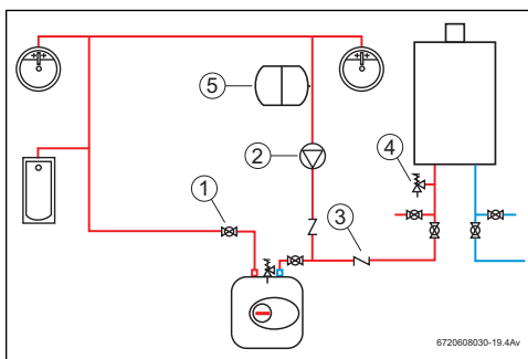
Fig. 15 Application de recirculation
