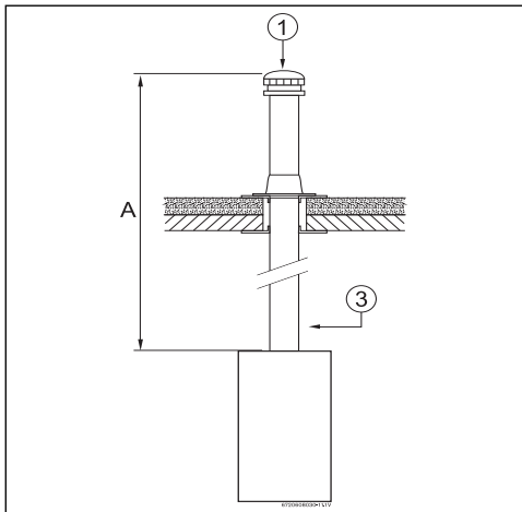
Fig. 9 Toit plat
