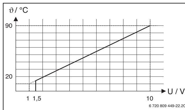
Sl.2 Linearni odnos između signala 0-10 V ( U u volt) i zatražene temperature polaznog voda \theta (u °C postocima naspram područja minimalne do maksimalne temperature polaznog voda [osnovna postavka 20 °C do 90 °C])
