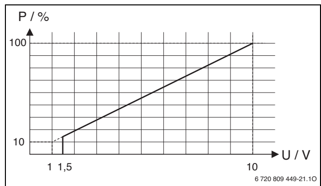
Att. 1 Lineārā attiecība starp 0-10 V signālu (U voltos) un pieprasīto jaudu P (procentos attiecībā uz sistēmas maksimālo jaudu)
