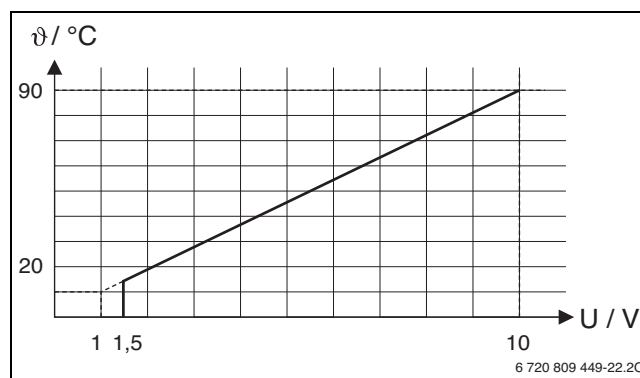
sl. 2 Linearna zavisnost između signala od 0-10 V (napon u voltima) i potrebne temperature polaznog voda \theta (u °C u odnosu na opseg od minimalne temperature polaznog voda do maksimalne temperature polaznog voda [osnovno podešavanje 20 °C do 90 °C])
