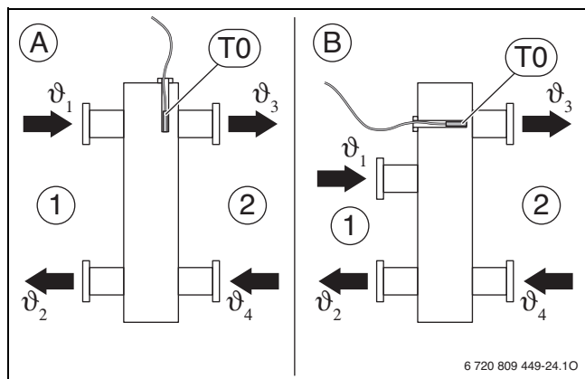
Joon. 4 Pealevoolu temperatuurianduri asukoht (T 0 )
