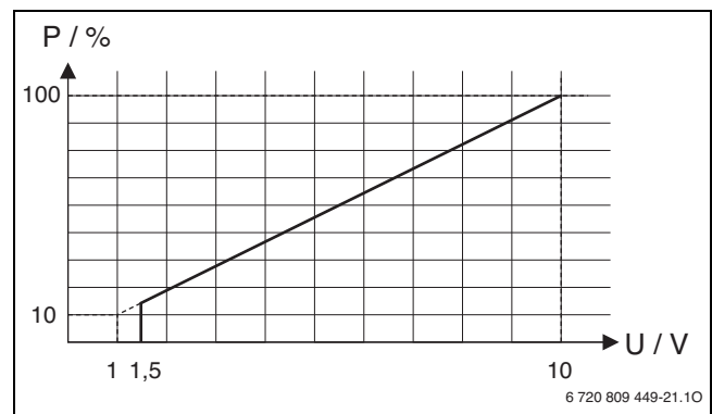
Рис. 1 Линейная зависимость между сигналом 0-10 В (напряжение в Вольтах) и требуемой мощностью P (в процентах от максимальной мощности установки)
