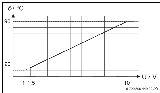
2. ábra Lineáris összefüggés a 0-10 V-os jel ( U fesz. V-ban) és az igényelt előremenő hőmérséklet között ( \theta °C-ban a minimális előremenő hőmérséklettől a maximális előremenő hőmérsékletig tartományra vonatkoztatva [alapbeállítás 20 °C ... 90 °C])
