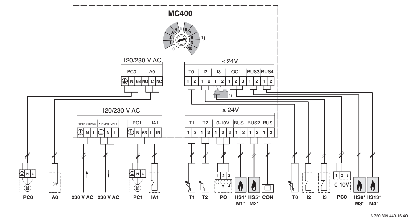
Legenda za sliku gore i sliku 24 do 26 (bez oznake priključnih stezaljki):
