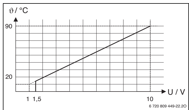
Att. 2 Lineāra saistība starp 0-10 V signālu (U voltos) un pieprasītās turpgaitas temperatūras θ (°C attiecās uz minimālās līdz maksimālās turpgaitas temperatūras diapazonu [pamatīestatījums 20 °C līdz 90 °C])
