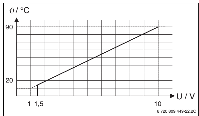
Pav. 2 Tiesinis ryšys tarp 0-10 V signalo ( U , voltais) ir reikalaujamos tiekiamo srauto temperatūros \theta (°C diapazono nuo minimalios tiekiamo srauto temperatūros iki maksimalios tiekiamo srauto temperatūros atžvilgiu [gamyklinis nustatymas nuo 20 °C iki 90 °C])
