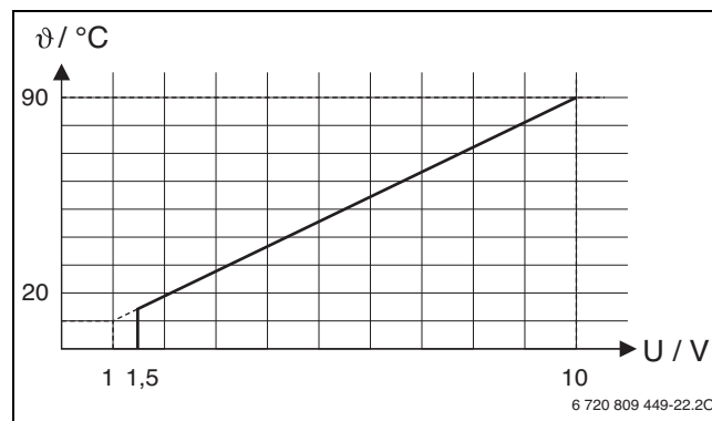
Fig. 2 Combinația liniară dintre semnalul 0-10 V (U în volți) și temperatura solicitată a turului θ (în °C bazată pe domeniul de temperatură minimă a turului până la temperatura maximă a turului [setare din fabrică 20 °C până la 90 °C])
