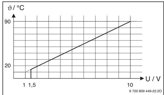
Sl.2 Linearna zveza med signalom 0–10 V ( U v Voltih) in zahtevano temperaturo dviznega voda \theta (v °C glede na območje od minimalne do maksimalne temperature dviznega voda [osnovna nastavitvev 20 °C do 90 °C])
