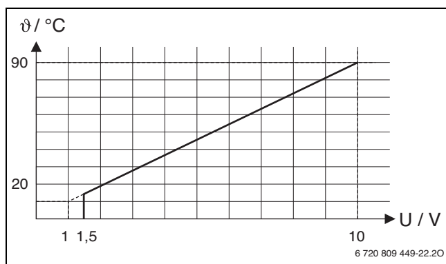
Рис. 2 Лінійна залежність між сигналом 0-10 В ( U у Вольтах) та необхідною температурою лінії подачі \theta (у °C відповідно до області від мінімальної до максимальної температури лінії подачі [заводські налаштування від 20 °C до 90 °C])
