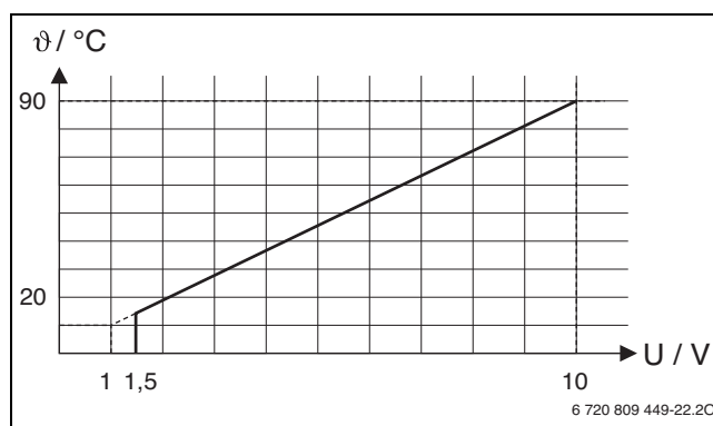
Фиг. 2 Линейна зависимост между сигнала 0 – 10 V ( U във волтове) и изискваната температура на подаване \theta (в °C за обхвата минимална температура до максимална температура на подаване [основна настройка 20 °C до 90 °C])
