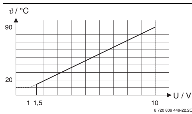
Joon. 2 Lineaarne sõltuvus 0–10 V signaali (U, voltides) ja vajaliku pealevoolutemperatuuri vahel \theta (°C vahemikus minimaalsest pealevoolutemperatuurist kuni maksimaalse pealevoolutemperatuurini [põhiseadistus 20 °C kuni 90 °C])
