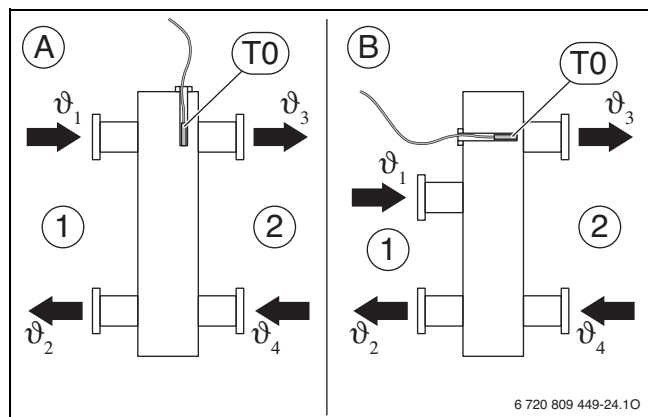
Sl. 4 Položaj tipala temperature dviznega voda (T0)
