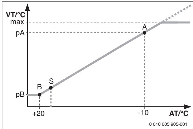
Рис. 73 Отопительная кривая
