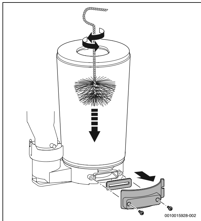
Рис. 48 Чистка теплообменника
