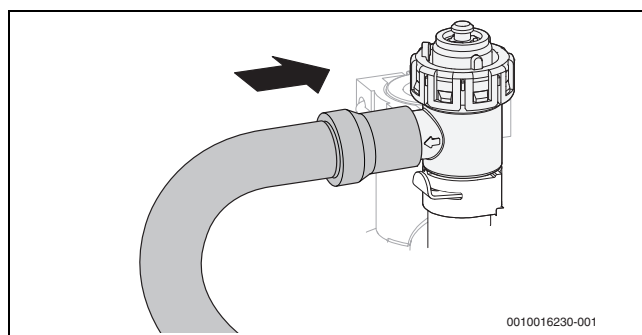
Рис. 24 Подсоединение шланга к предохранительному клапану
