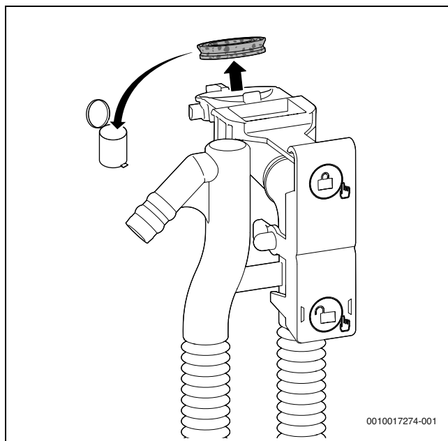
Рис. 53 Демонтаж уплотнения сверху на сифоне для отвода конденсата
