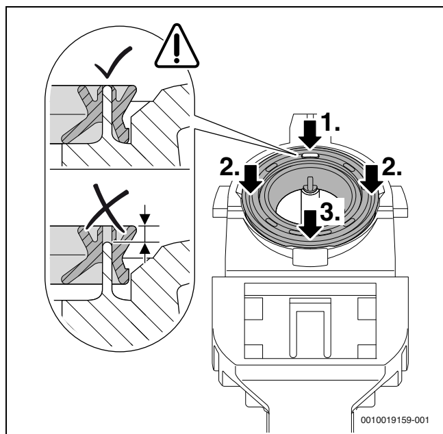
Рис. 55 Прижатие уплотнения
