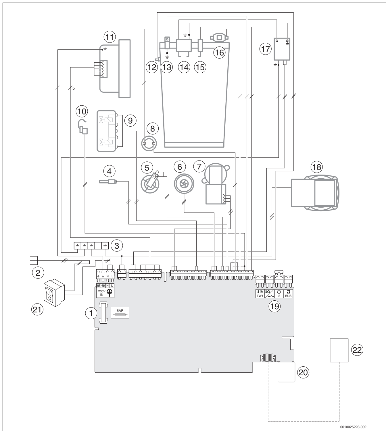
Рис. 72 Электрические соединения
