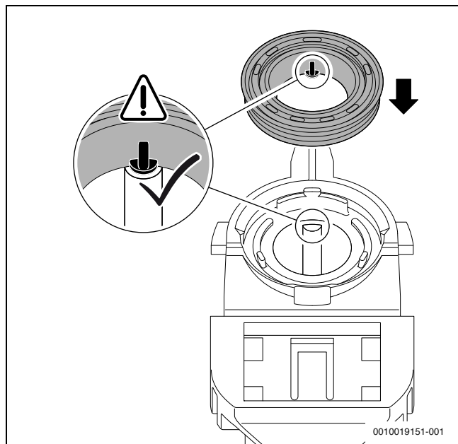
Рис. 54 Выравнивание нового уплотнения на сифоне для отвода конденсата
