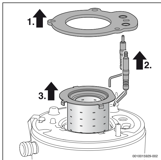
Рис. 45 Выньте горелку
