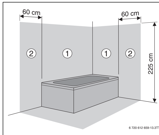
Рис. 27 Зоны безопасности
