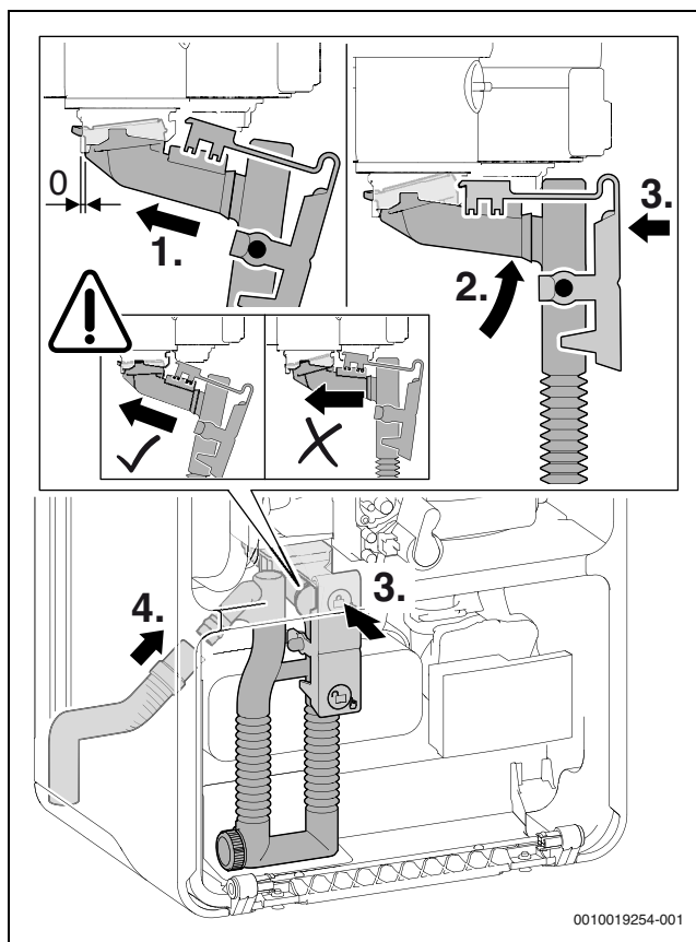
Рис. 56 Установка сифона для отвода конденсата
