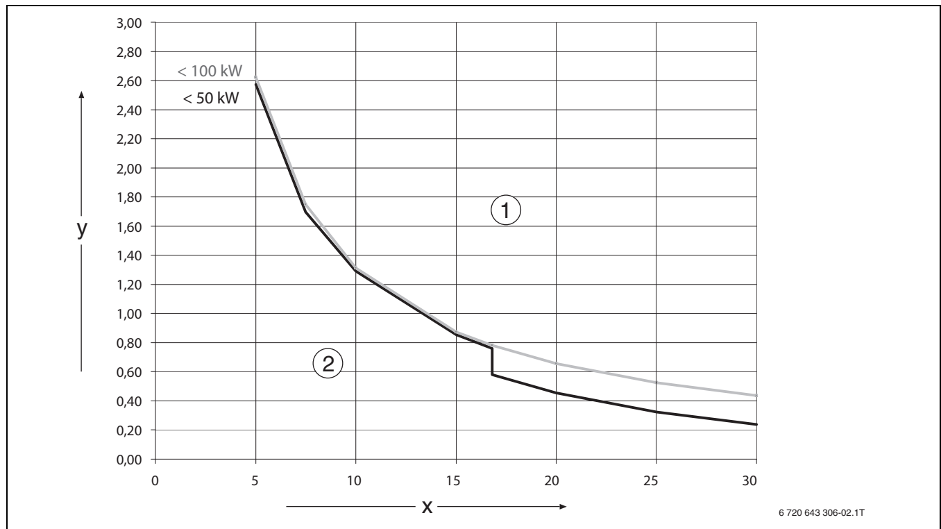
Рис. 1 Требования к воде заполнения и подпитки для котлов < 100 кВт с теплообменником из алюминиевых материалов
