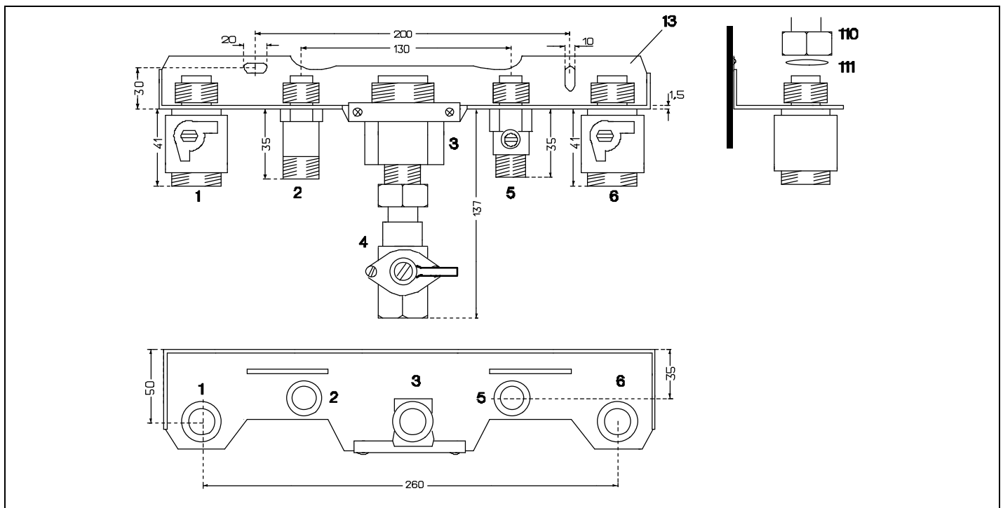
Fig. 2 montageplaat / plaque de montage
