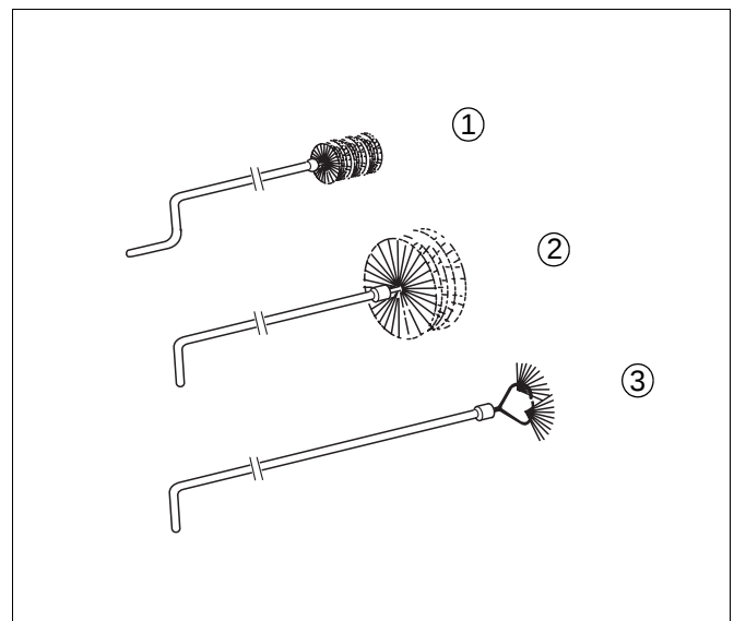
Abb. 77 Reinigungsbürsten
