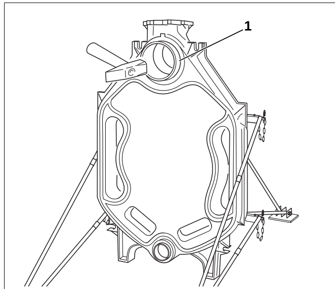
Abb. 14 Nippel einschlagen
