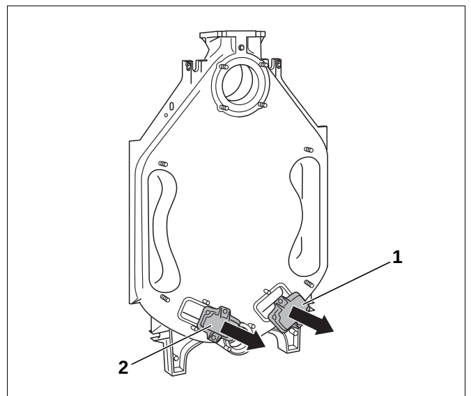
Abb. 10 Reinigungsdeckel demontieren
