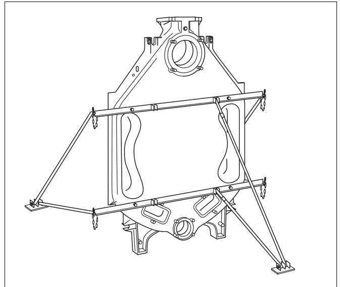
Abb. 11 Montagehilfe befestigen
