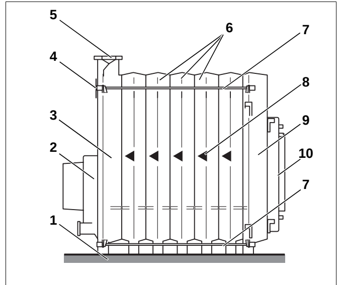
Abb. 8 Kesselblock
