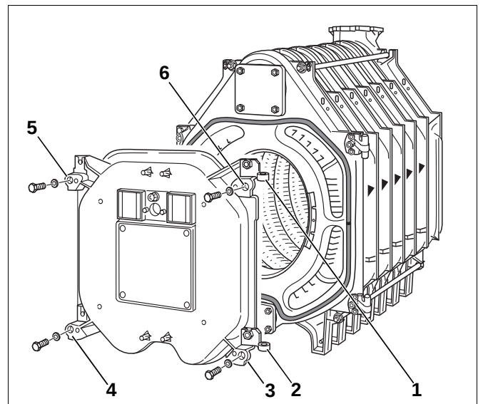
Abb. 34 Brennertür einhängen
