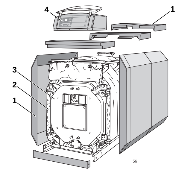
Abb. 1 Öl-/Gas-Spezialheizkessel TG 52
