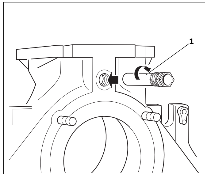
Abb. 25 Tauchhülse montieren
