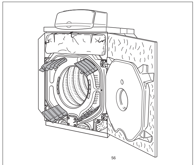
Abb. 70 Position der Heizgaslenkplatten prüfen
