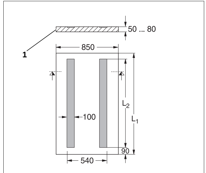
Abb. 7 Fundamentabmessungen (Maße in mm)
