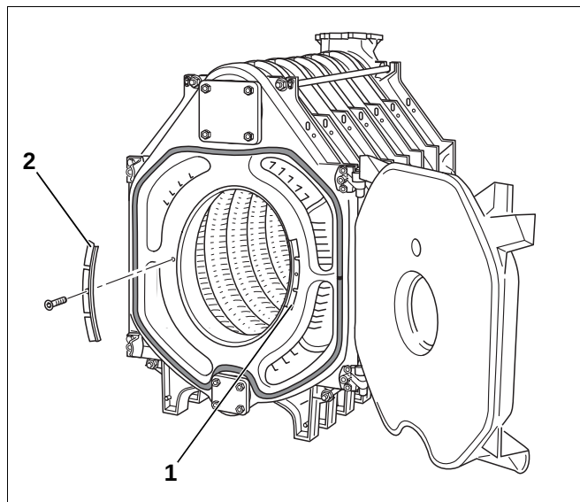
Abb. 35 Position der Heizgassperrplatten
