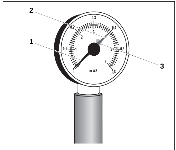
Abb. 81 Hydrometer für offene Heizungsanlagen
