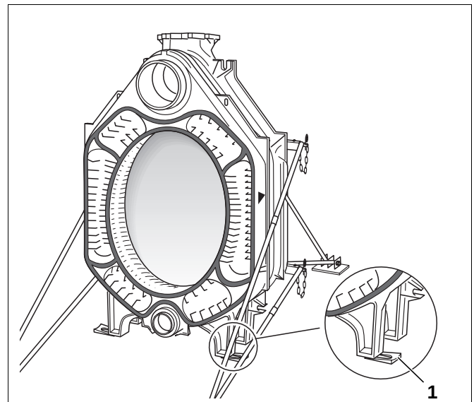
Abb. 21 Kesselgliedfußkeile verwenden
