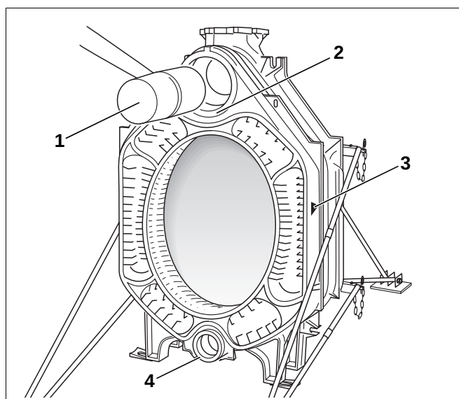
Abb. 18 Mittelglied anschlagen
