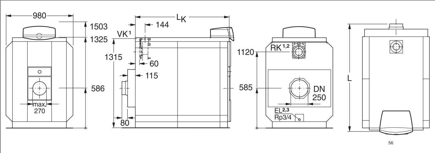
Abb. 3 Technische Daten für TG 52 (Maße in mm)
