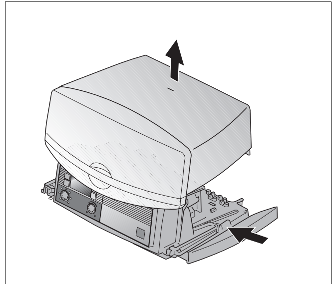
Abb. 63 Abdeckhaube abnehmen
