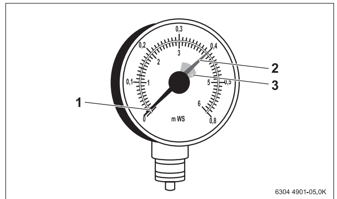
Abb. 30 Hydrometer für offene Anlagen
