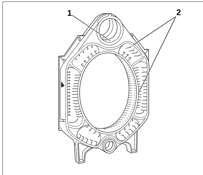
Abb. 17 Mittelglied vorbereiten
