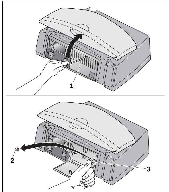
Abb. 84 Sicherheitstemperaturbegrenzer (STB) entriegeln
