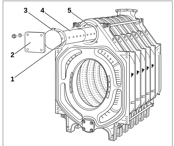
Abb. 24 Einspeiserohr montieren
