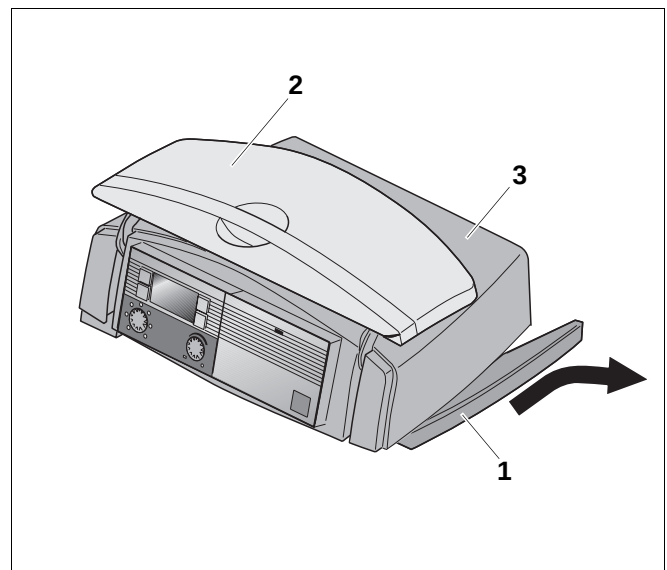
Abb. 62 Abdeckhaube des Schaltfeldes lösen
