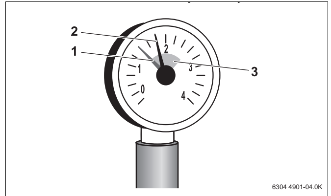
Abb. 29 Manometer für geschlossene Anlagen
