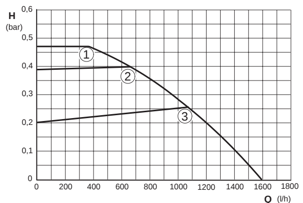
Bild 43 Konstantdruck
