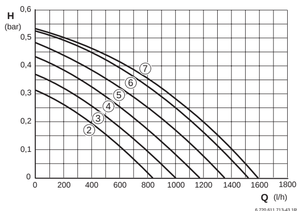
Bild 48 Kennlinien
