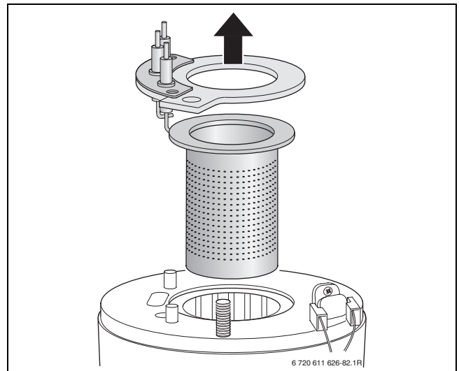
Bild 60 Brenner herausnehmen
