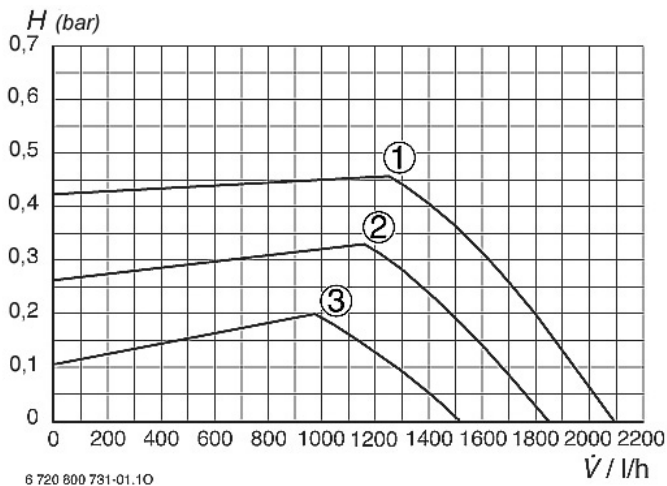
Fig. 48 pression constante (chaudière ZB)
