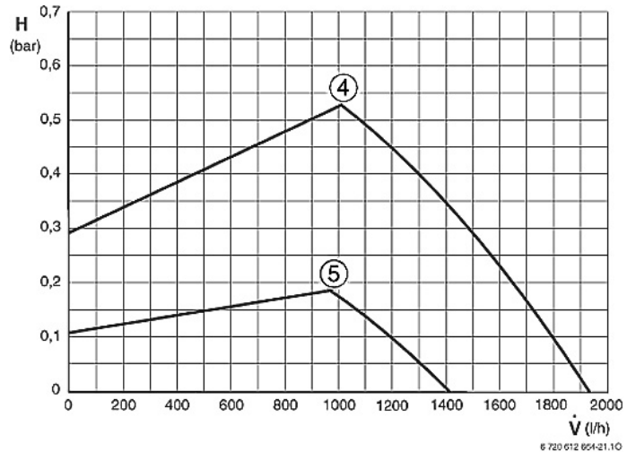
Fig. 47 pression proportionnelle (chaudières ZWB & ZSB)
