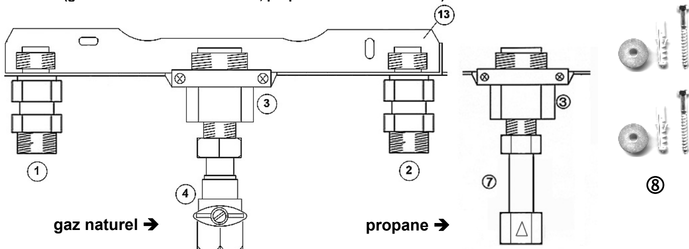
Fig. 12 Plaque de montage pour TOP 42-3 ZB (gaz naturel = n°. 7 719 002 135, propane = n°. 7 719 003 943)
