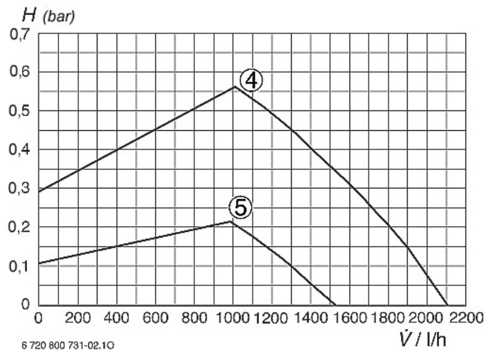
Fig. 49 pression proportionnelle (chaudière ZB)
