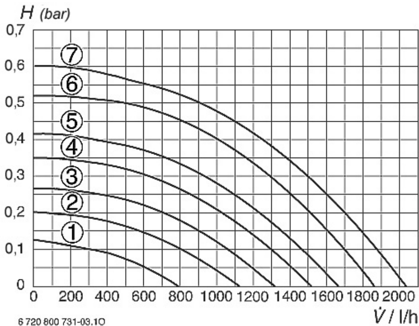
Fig. 51 position circulateur intelligent (chaudière ZB)
