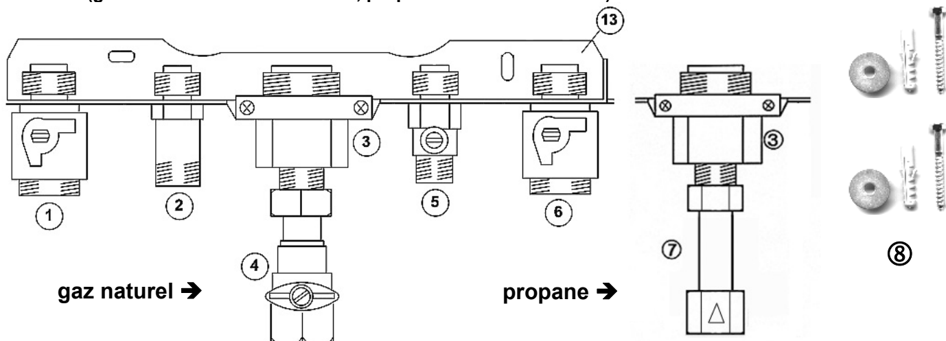
Fig. 10 Plaque de montage pour TOP 30-3 ZWB, TOP 42-3 ZWB & TOP 28-3 ZSB (gaz naturel = n°. 7 719 002 134, propane = n°. 3 119 001 823)
