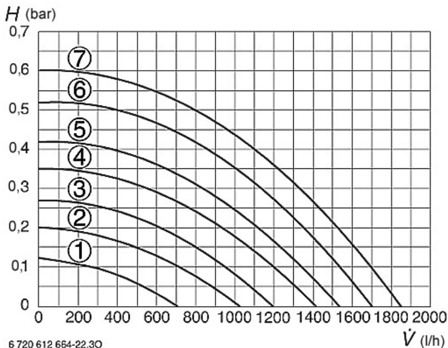
Fig. 50 position circulateur intelligent (chaudières ZWB & ZSB)
