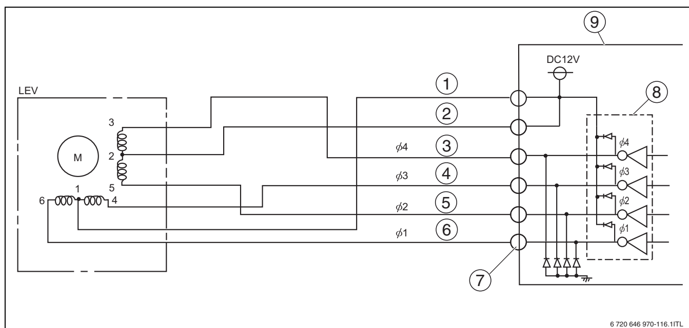
Bild 64 Schaltplan linearer Expansionsventile LEV
