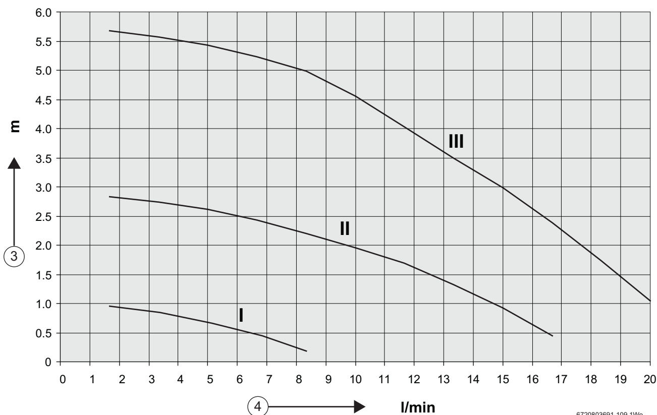
Bild 49 Verfügbare Förderhöhe
