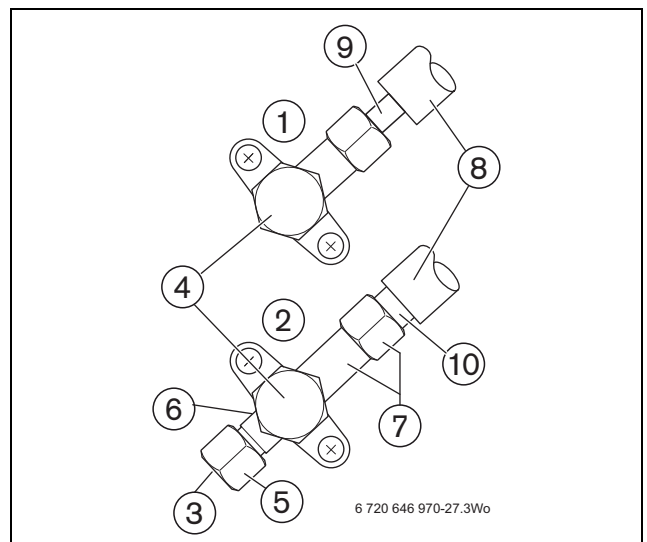
Bild 33 Absperrventile Kältemittelkreislauf
