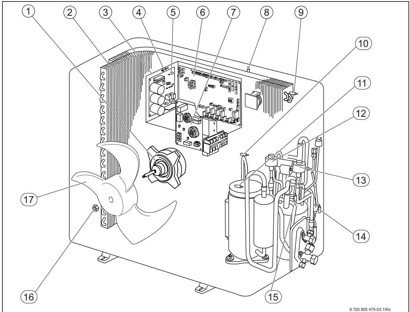
Bild 74 Lüftermotor ersetzen
