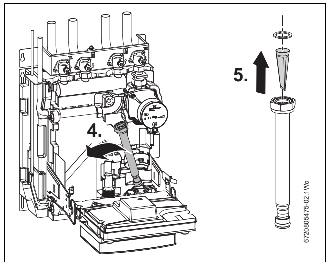
Bild 59 Ausbau des Filters
