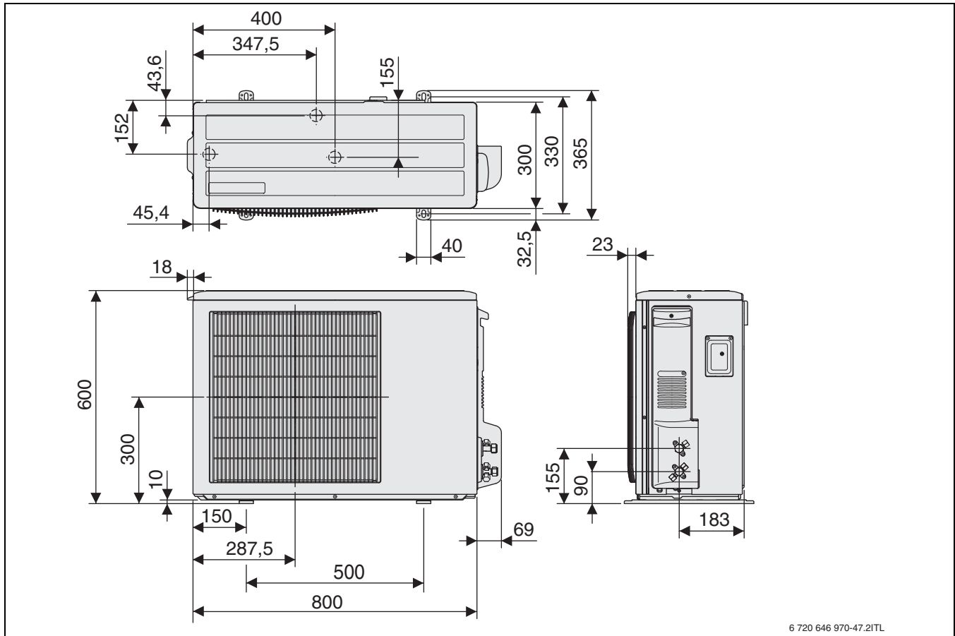
Bild 17 Abmessungen Außeneinheit
