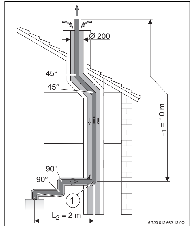
Bild 19 Einbausituation einer Abgasführung nach C_{93x}
