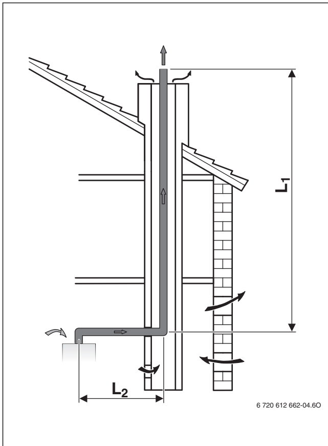
Bild 8 Abgasführung im Schacht nach B 23
