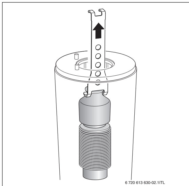
Bild 98 Oberen Verdrängungskörper herausnehmen
