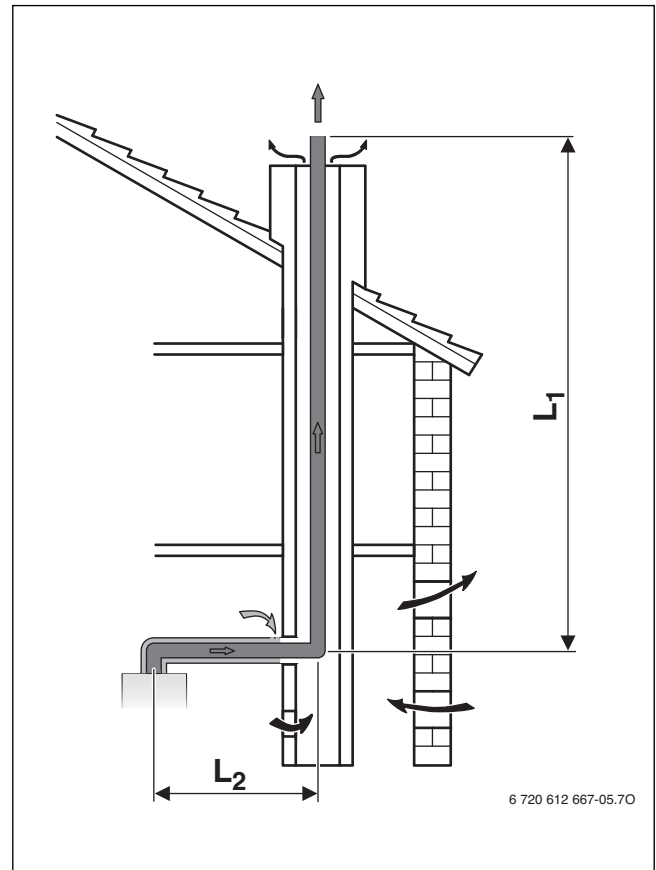
Bild 10 Abgasführung im Schacht nach B 33x
