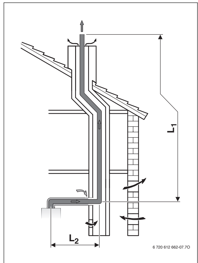
Bild 11 Abgasführung im Schacht nach B 33x
