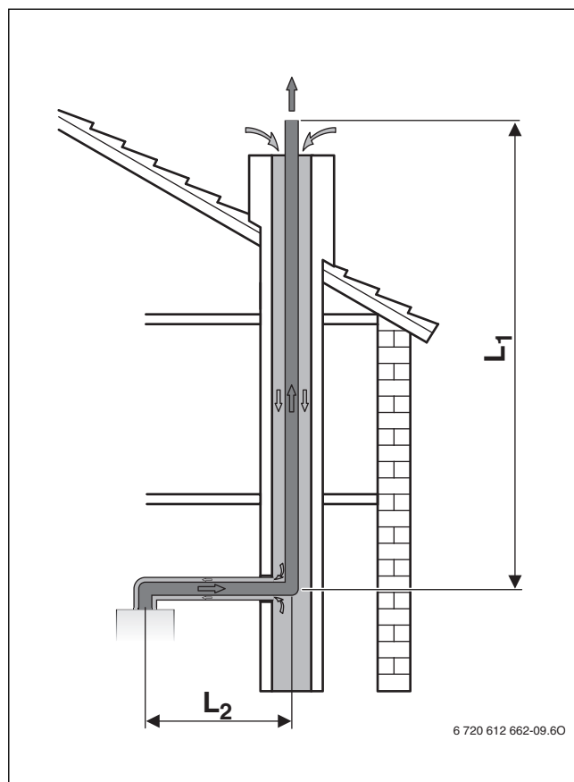
Bild 16 Abgasführung im Schacht nach C 93x
