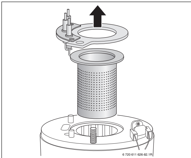
Bild 88 Brenner herausnehmen
