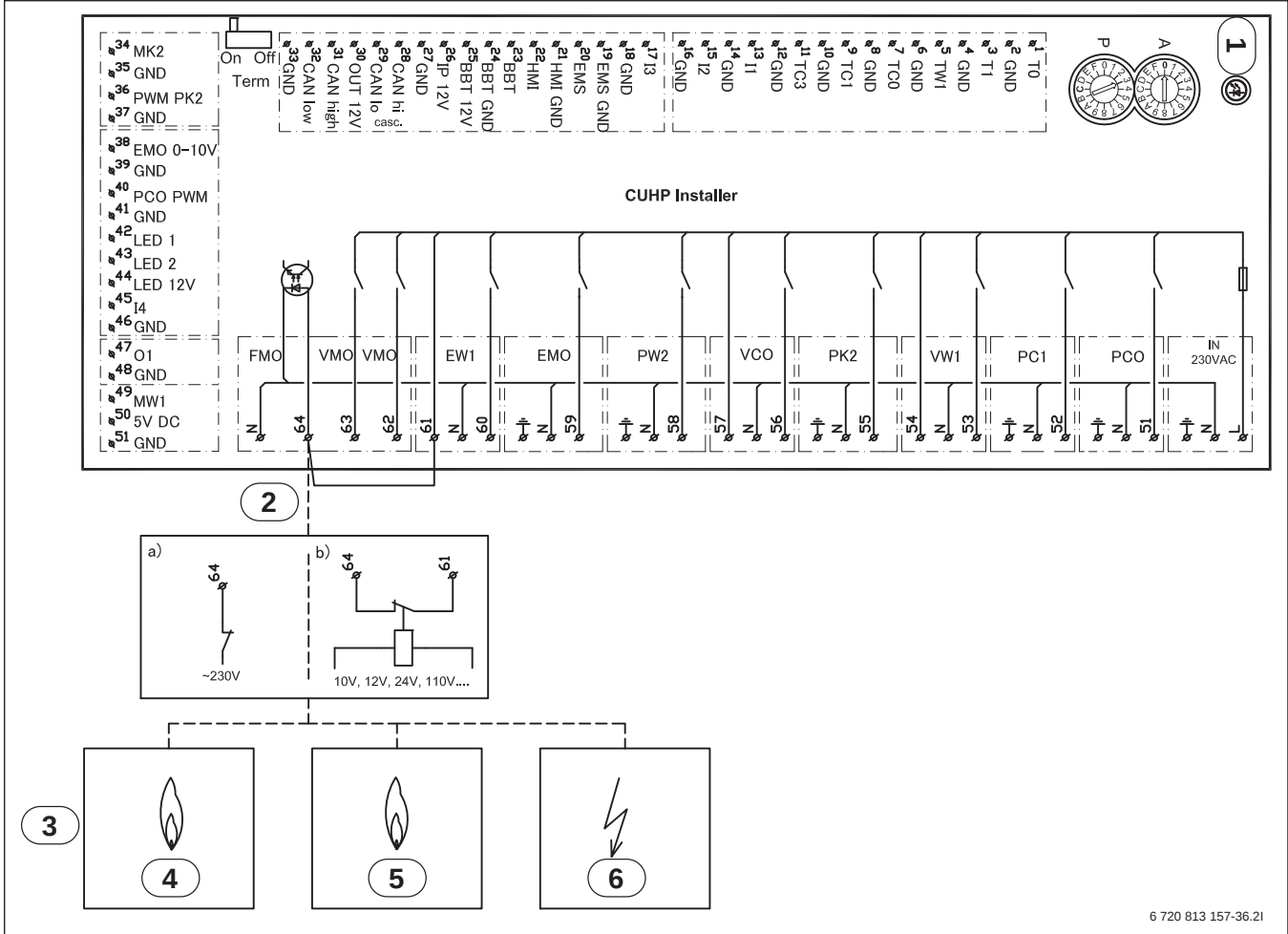
Bild 58 Schaltschema des Installationsmoduls, Alarm für externen Zuheizier (z. B. Heizkessel)
