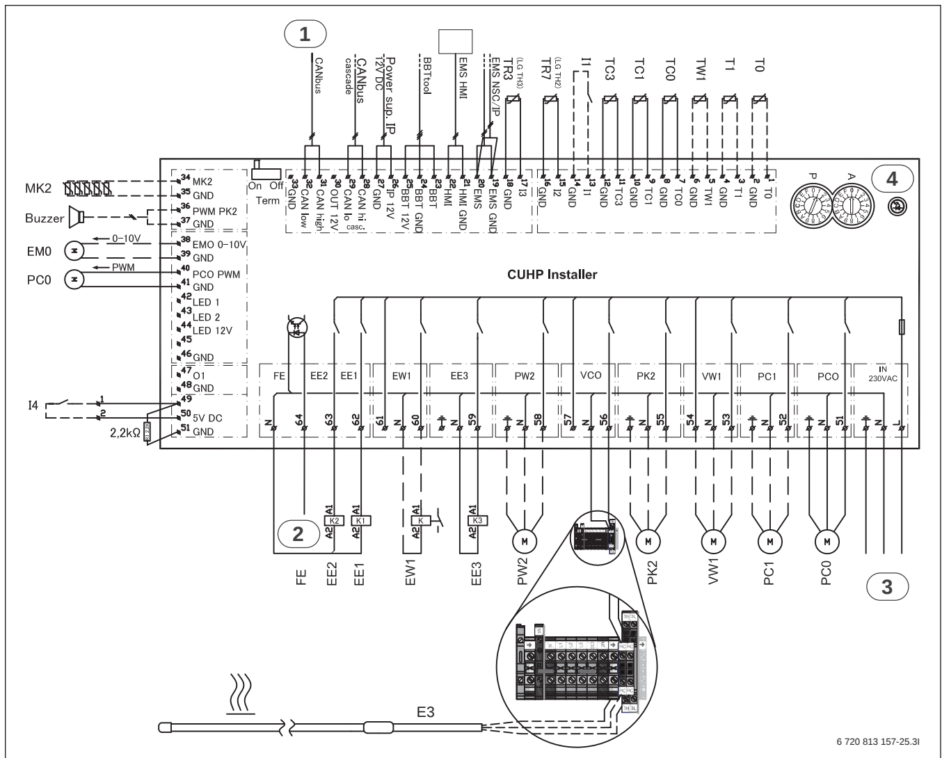
Bild 52 Installationsmodul SEC 20, in der Inneneinheit mit integriertem elektrischen Zuheiz (ASE 6/ASE 13)
