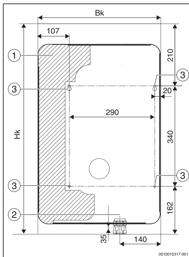
Мал. 9 Розміри отворів для кріплення опалювального котла на стіні та для кабелю живлення опалювального котла Tronic Heat 3500 15–24 кВт
