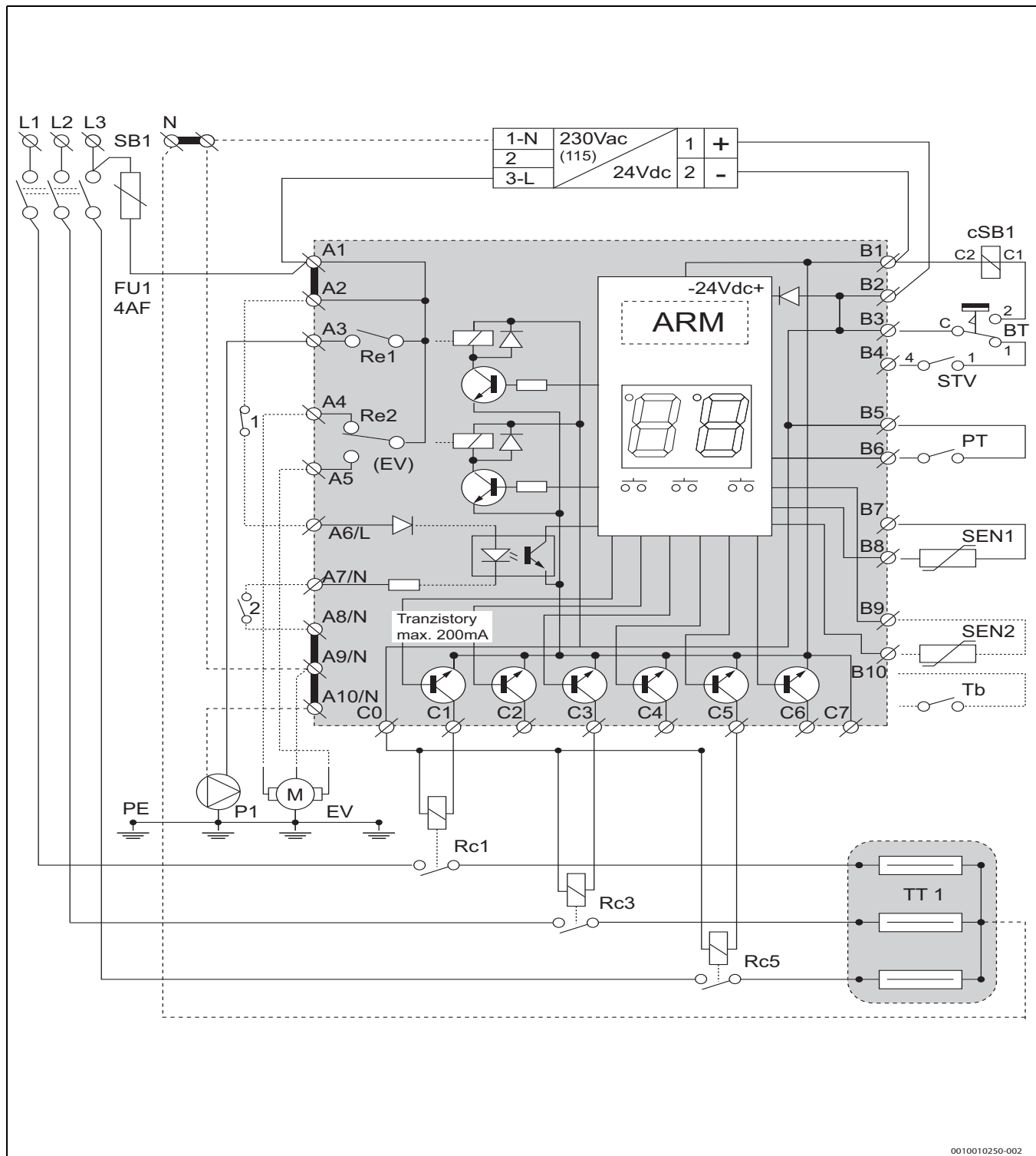
Мал. 20 Схема техобслуговування опалювального котла Tronic Heat 3500 (4–12 кВт), 3х 400/230 В АС
