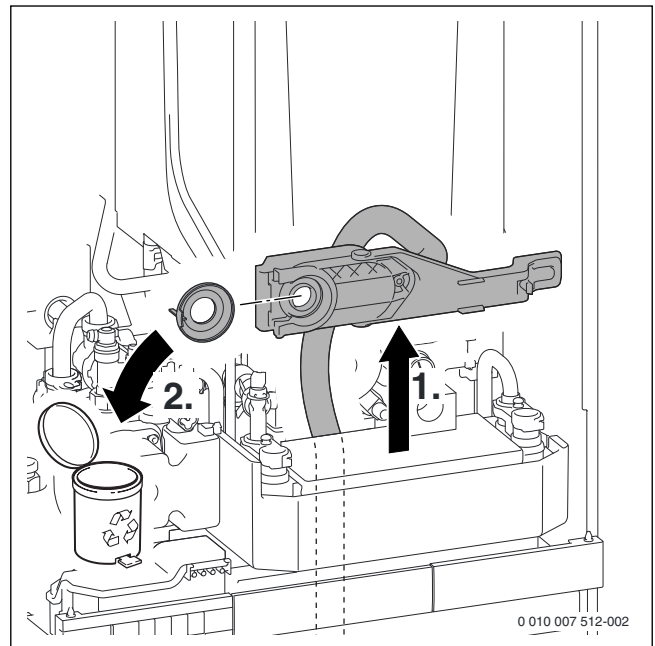
Fig. 40 Retirer le filtre de la position d'entretien et retirer le couvercle de protection
