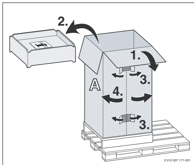
Fig. 35 Déballer le ballon
