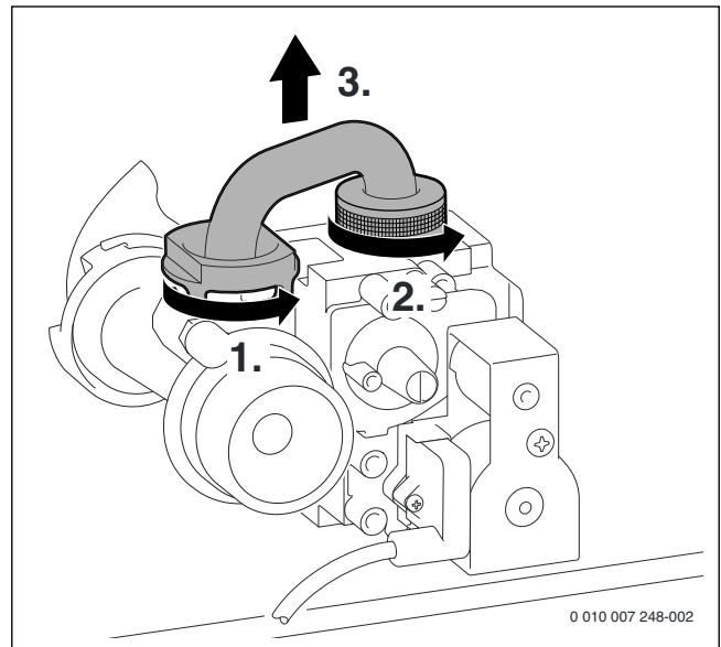
Fig. 103 Retirer le tuyau de gaz
