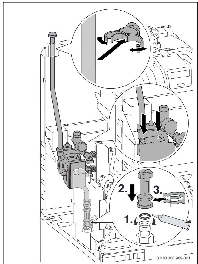
Fig. 57 Accrocher le groupe solaire dans le support et raccorder le débitmètre au ballon
