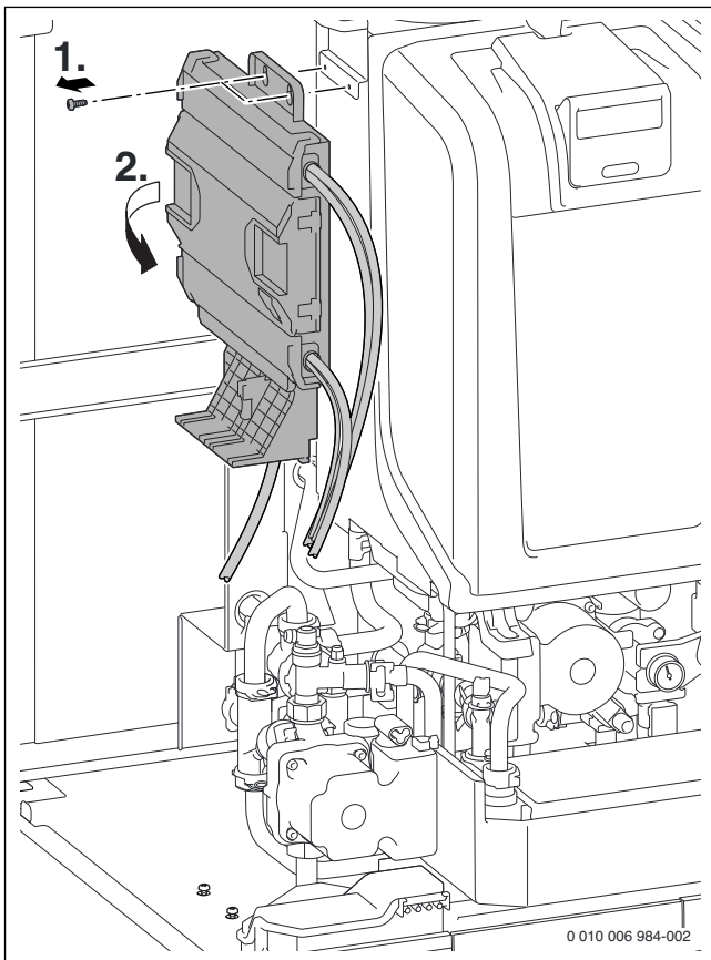
Fig. 46 Retirer l'appareil de commande
