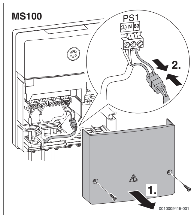
Fig. 60 Raccorder le connecteur du limiteur de température solaire MS1 dans le module MS 100
