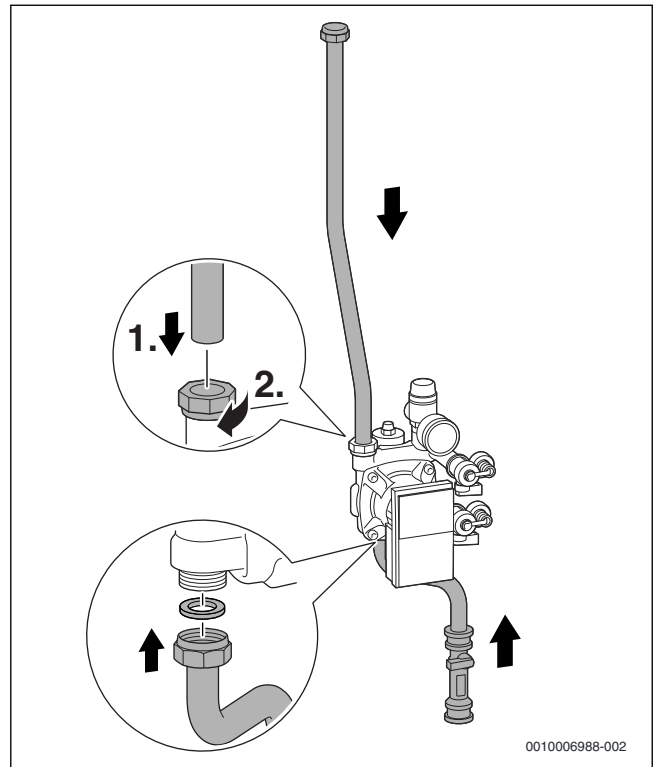
Fig. 56 Monter le tuyau solaire de retour et le limiteur de débit au groupe solaire
