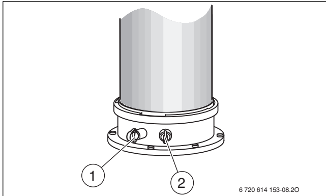
Fig. 86 Embout de mesure des fumées et de l'air de combustion
