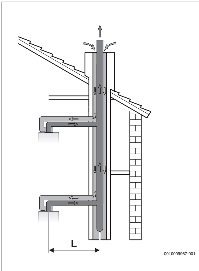
Fig. 28 Affectation multiple avec tube séparé selon C 43
