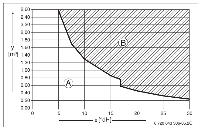
Fig. 30 Conditions requises pour l'eau de remplissage et d'appoint sur les appareils < 50 kW
