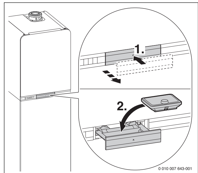
Fig. 70 Insérer le régulateur de chauffage
