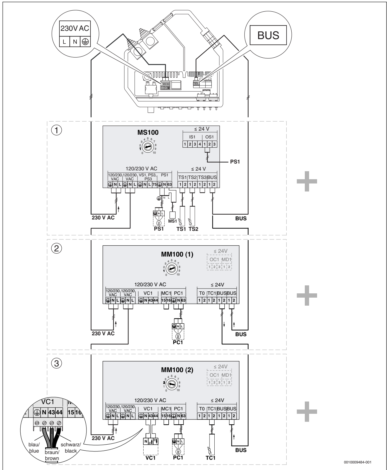
Fig. 66 Raccordement des modules MS 100 et MM 100, si existants
