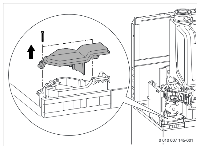
Fig. 63 Retirer le couvercle du boîtier de raccordement
