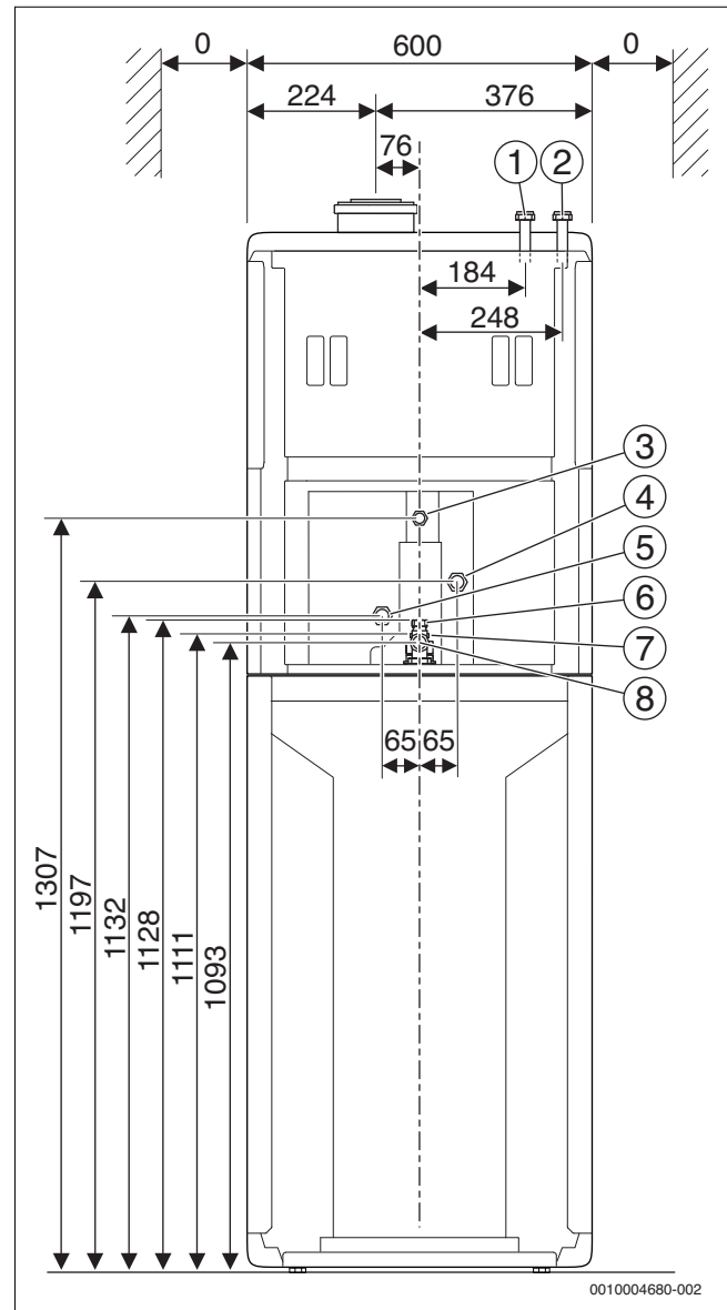
Fig. 3 Dimensions et raccordements sans accessoires (dimensions en mm) (distance recommandée par rapport au mur \geq 50 mm)
