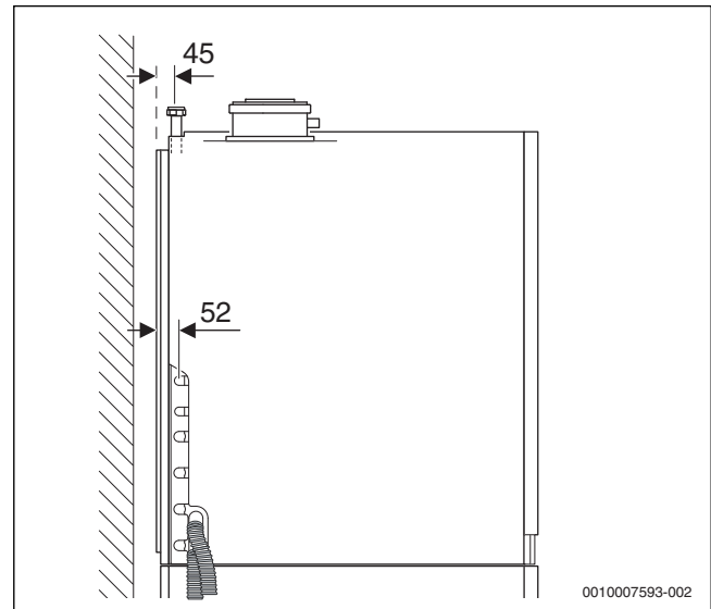
Fig. 8 Dimensions de raccordement de l'accessoire CS 12 - Kit d'extension 1 circuit de chauffage (en mm)
