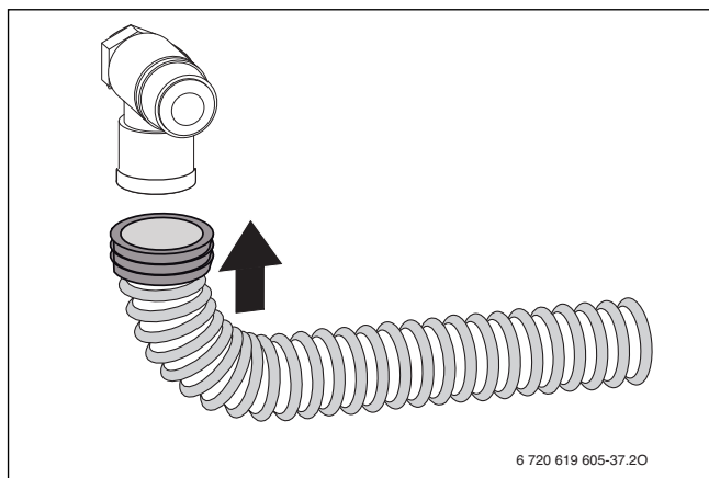
Fig. 32 Monter le flexible sur la soupape de sécurité
