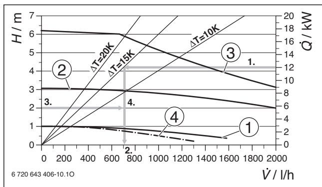
Fig. 115 Courbes caractéristiques de la pompe
