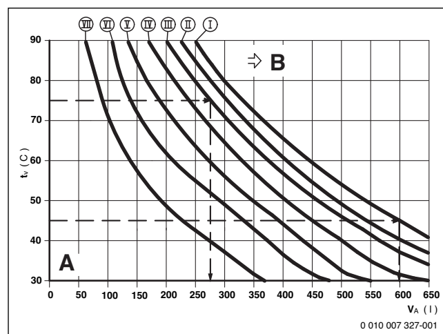
Fig. 31 Courbes caractéristiques du vase d'expansion 18 l
