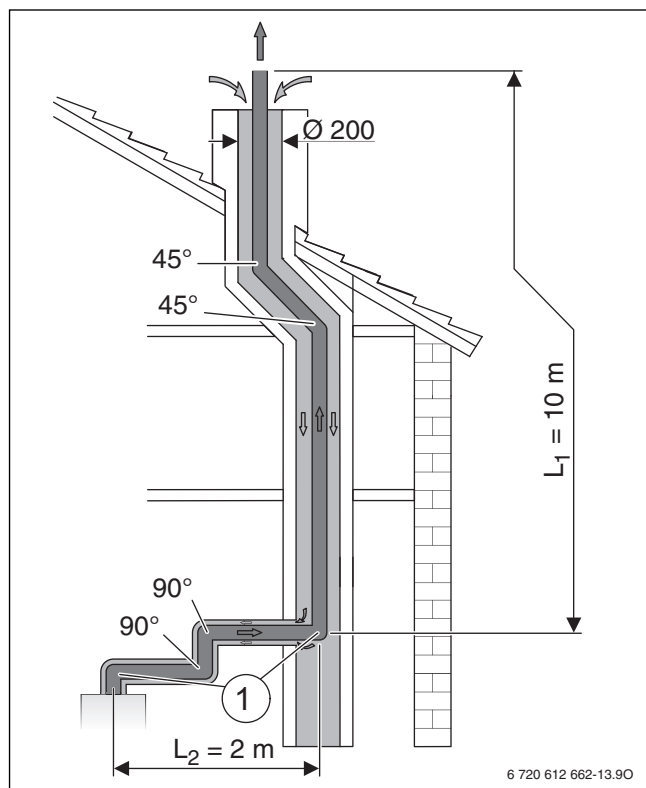
Fig. 26 Situation de montage d'un système d'évacuation des fumées selon C_{93}
