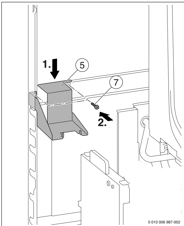
Fig. 55 Fixer le support du groupe solaire à l'aide de la vis
