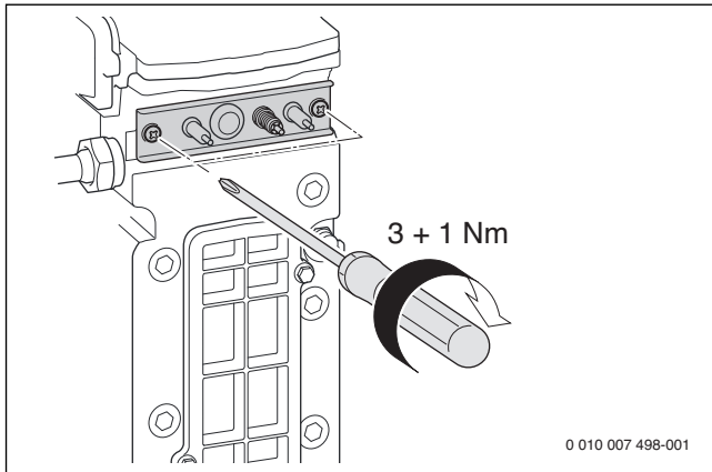
Fig. 87 Remonter le jeu d'électrodes
