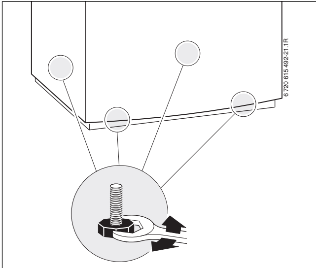
Fig. 37 Positionner le ballon
