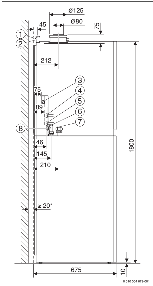
Fig. 2 Dimensions et raccordements sans accessoires (en mm)
