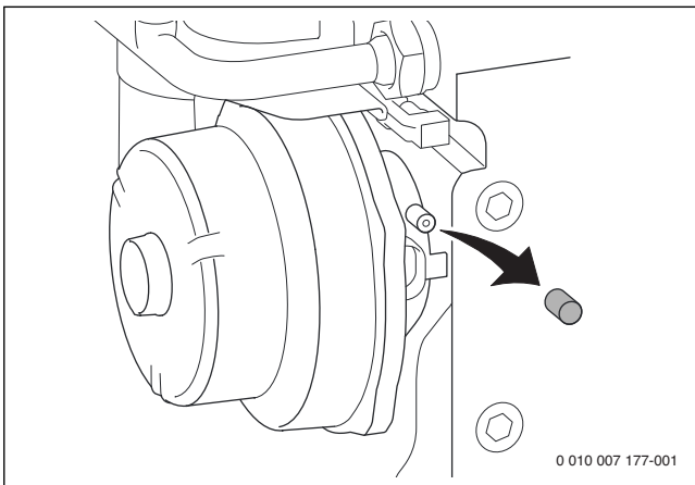
Fig. 92 Buse de mesure sur la chambre de mélange
