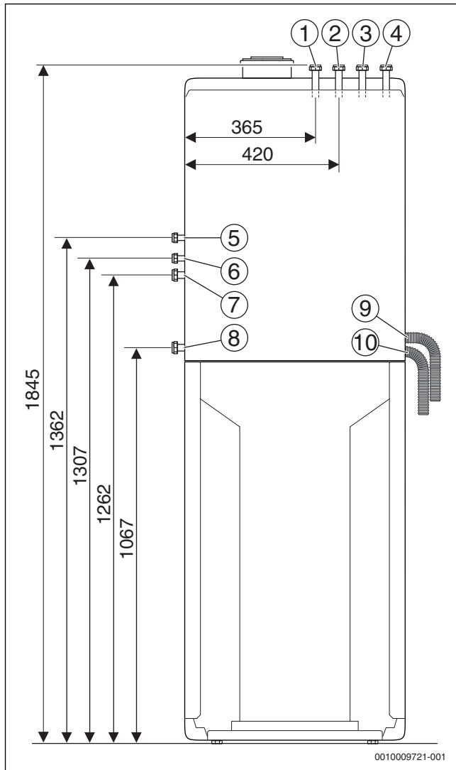
Fig. 7 Dimensions de raccordement de l'accessoire CS 12 - Kit d'extension 1 circuit de chauffage (en mm)
