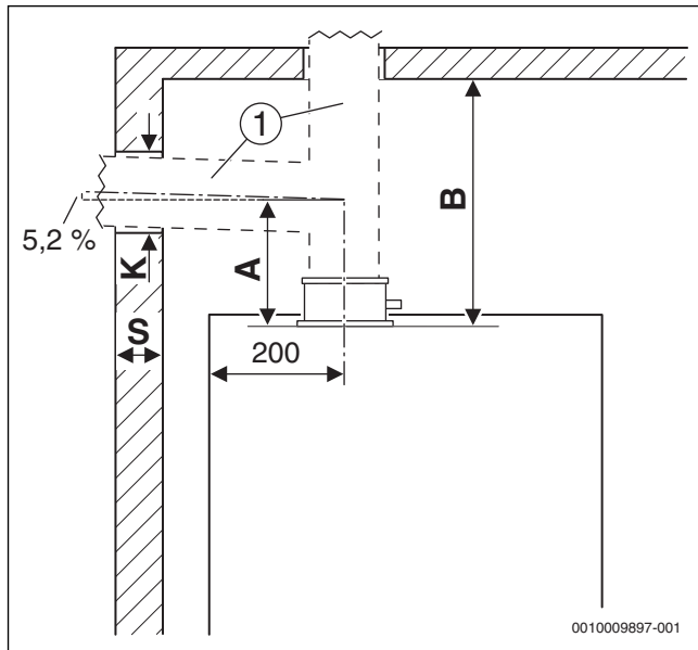
Fig. 11 Dimensions et distances minimales
