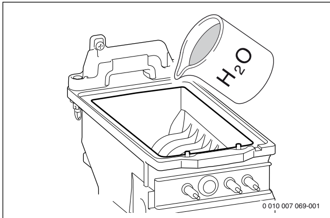
Fig. 95 Rinçage
