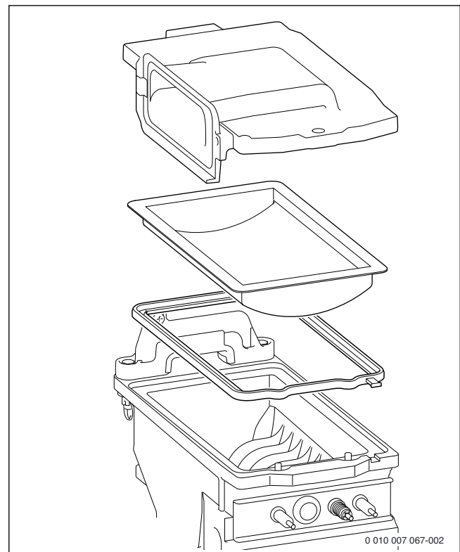
Fig. 90 Brûleur
