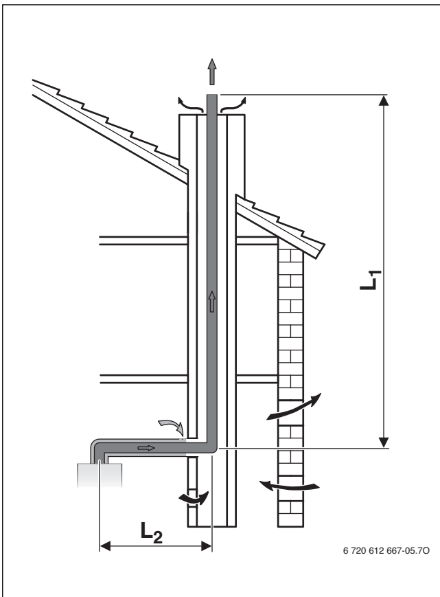
Fig. 17 Evacuation des fumées dans le conduit selon B 33
