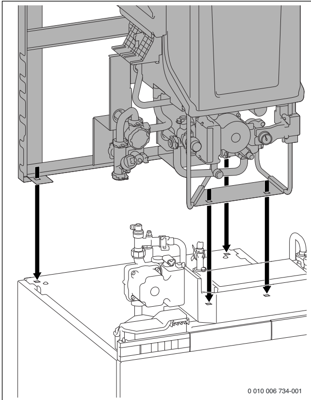
Fig. 38 Placer l'appareil sur le ballon
