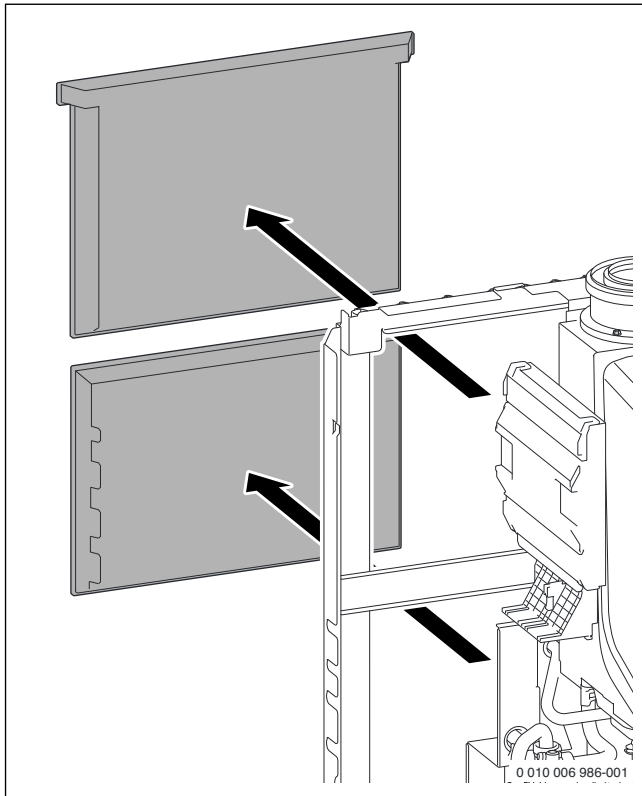
Fig. 54 Retirer les isolations thermique à l'arrière
