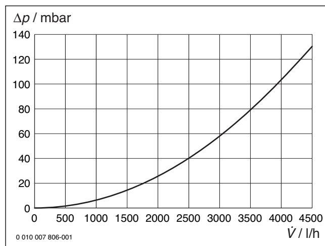
Fig. 111 Diagramme pertes de pression circuit de chauffage sans mélangeur (HK1)
