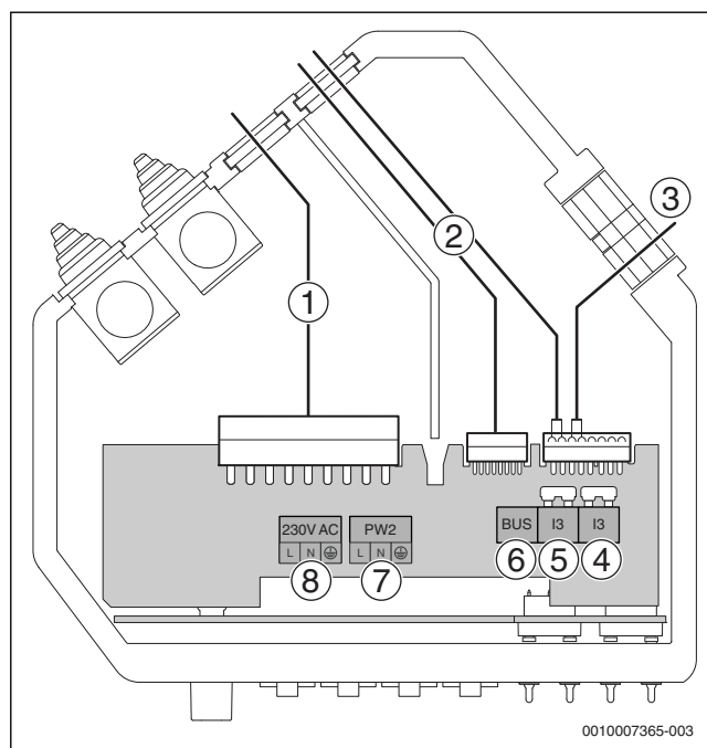
Fig. 65 Boîtier de raccordement
