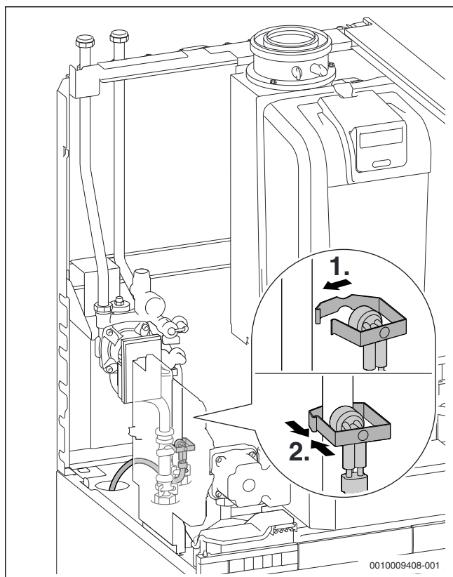
Fig. 59 Monter le limiteur de température solaire MS1 sur le tube de départ solaire
