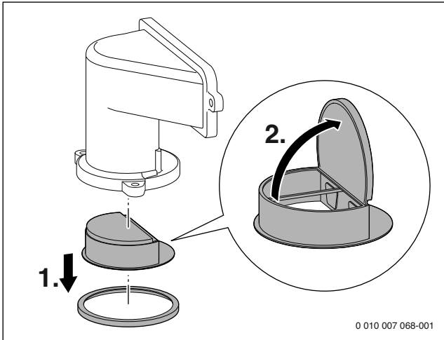
Fig. 100 Clapet anti-retour du dispositif de mélange
