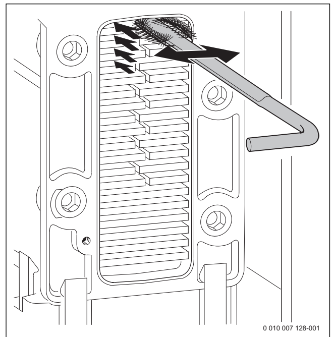
Fig. 94 Nettoyer l'échangeur de chaleur à l'aide de la brosse
