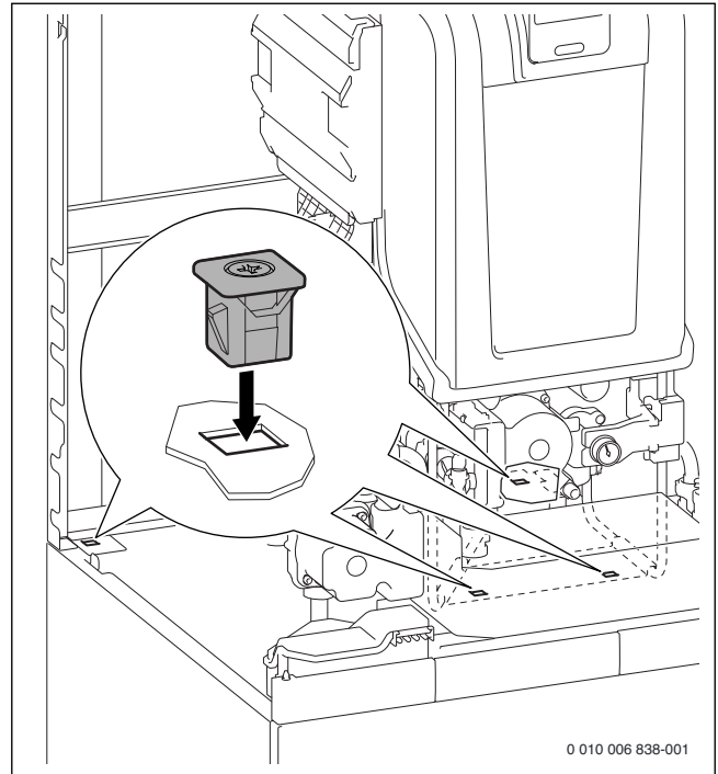
Fig. 39 Fixer l'appareil sur le ballon avec les 4 clips joints
