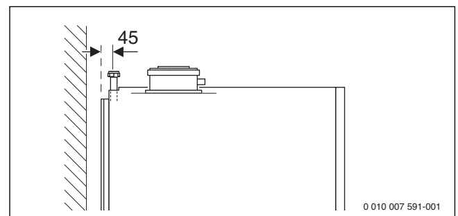
Fig. 6 Dimensions de raccordement de l'accessoire CS 11 - Kit de raccordement vertical (en mm)
