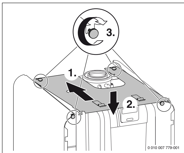
Fig. 76 Glisser le carénage supérieur vers l'arrière et fixer à l'avant et l'arrière avec les 4 vis
