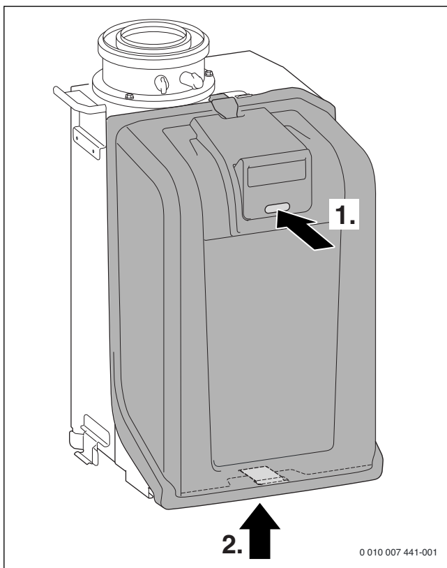
Fig. 83 Retirer le capot du brûleur
