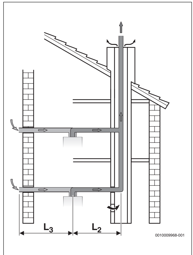
Fig. 29 Affectation multiple avec tube séparé selon C 83
