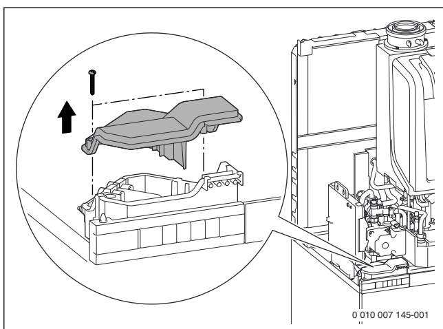
Fig. 50 Retirer le couvercle du boîtier de raccordement
