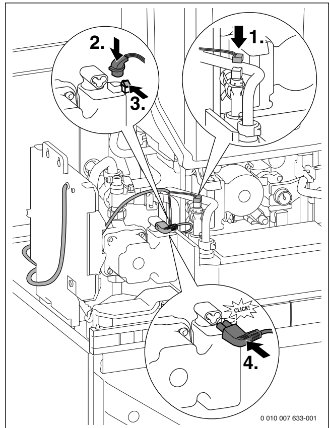
Fig. 48 Raccorder la pompe de charge ECS et la sonde de température ECS
