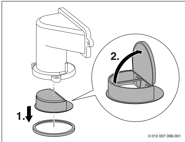
Fig. 91 Clapet anti-retour du dispositif de mélange
