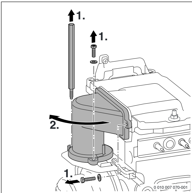
Fig. 99 Démontez le dispositif de mélange
