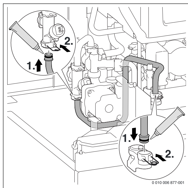
Fig. 44 Raccorder le tuyau entre la vanne à 3 voies et l'échangeur à plaque (départ)
