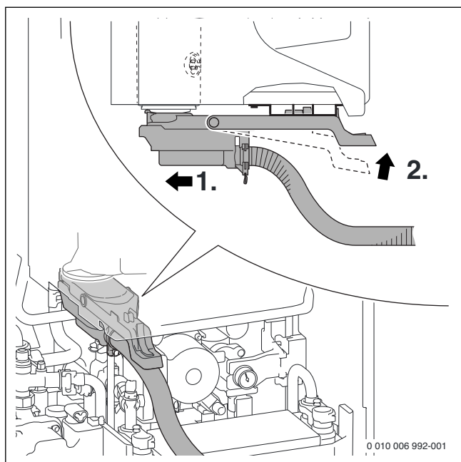
Fig. 41 Monter le filtre
