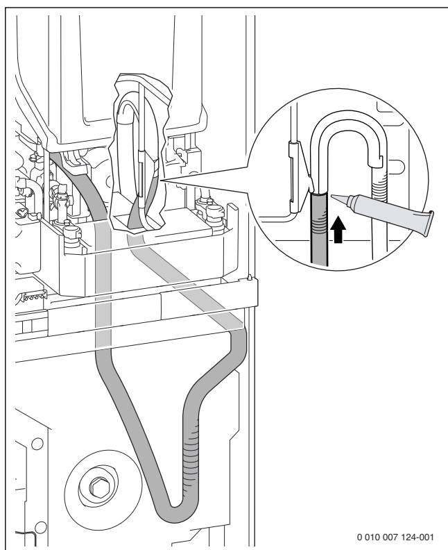
Fig. 42 Insérer le tube siphon sur l'élément d'extrémité
