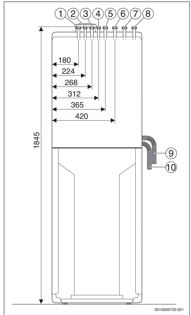
Fig. 5 Dimensions de raccordement de l'accessoire CS 11 - Kit de raccordement vertical (en mm)
