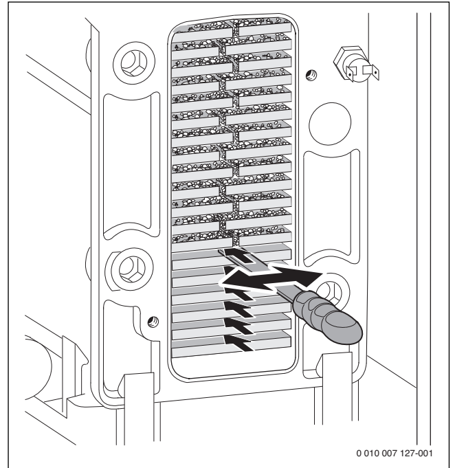
Fig. 93 lame de nettoyage
