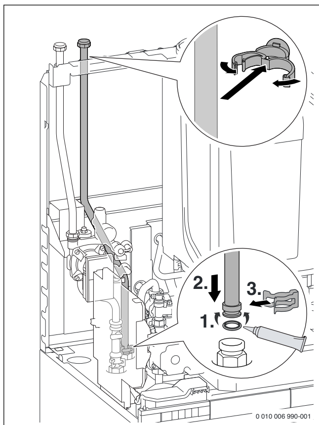
Fig. 58 Monter le tube de départ solaire et fixer le tube en haut
