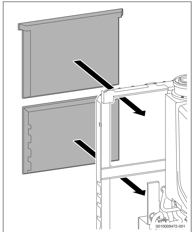
Fig. 74 Montage des isolations thermiques à l'arrière
