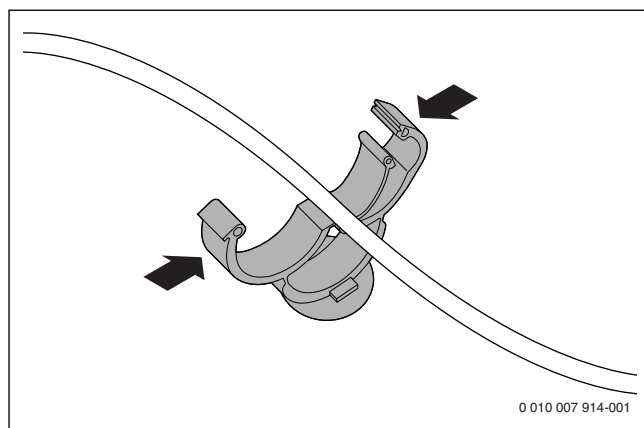
Fig. 52 Fixer le câble avec les clips
