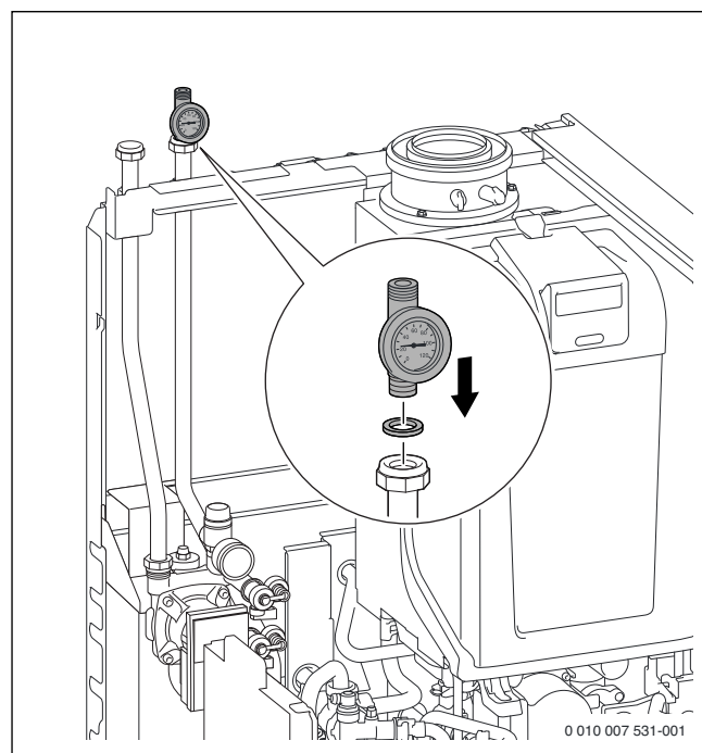
Fig. 61 Monter la vanne d'isolement avec thermomètre sur le tuyau de départ solaire
