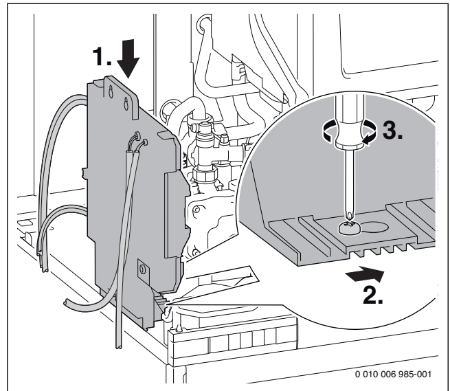
Fig. 47 Fixer l'appareil de commande sur le ballon
