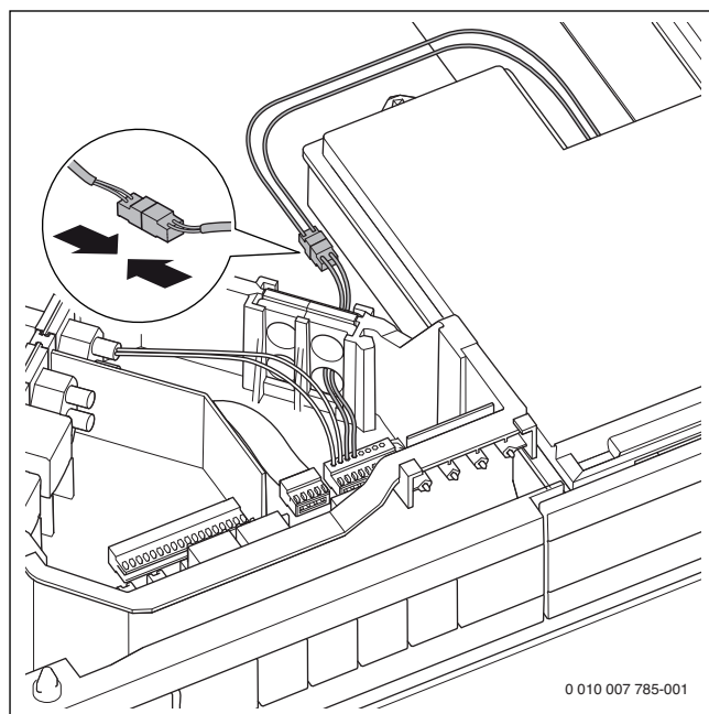
Fig. 53 Raccorder le tiroir du régulateur au boîtier de raccordement
