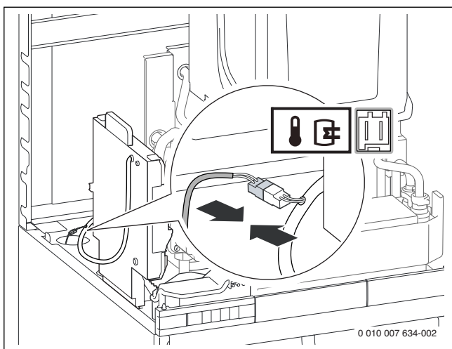
Fig. 49 Raccorder la sonde de température ballon
