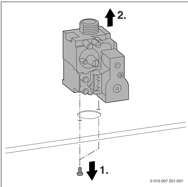
Fig. 105 Démonter le bloc gaz
