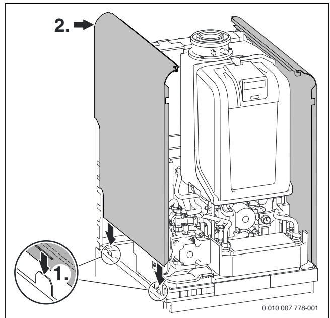
Fig. 75 Monter le carénage droit et gauche
