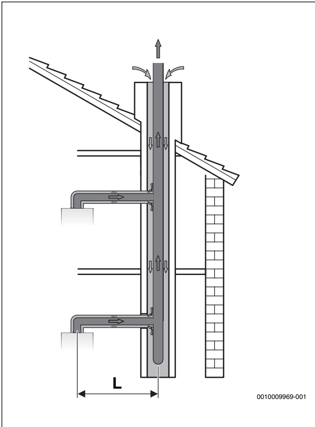
Fig. 27 Affectation multiple avec tube concentrique selon C 43
