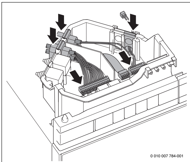
Fig. 51 Raccorder l'appareil de commande au boîtier de raccordement
