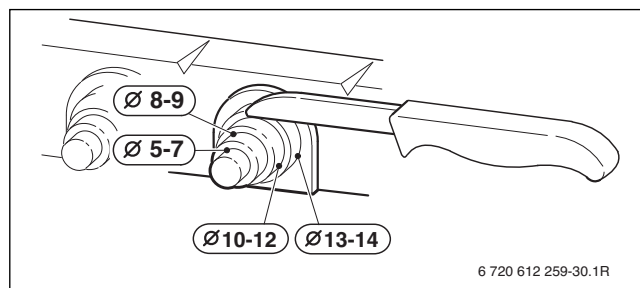
Fig. 64 Adapter le serre-câble au diamètre du câble
