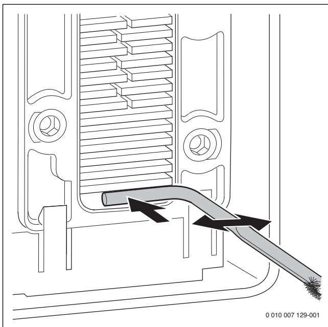
Fig. 96 Nettoyer le bac des condensats
