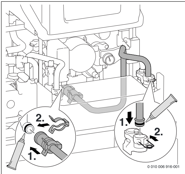
Fig. 45 Raccorder le tuyau entre l'échangeur à plaque et le corps de chauffe (retour)
