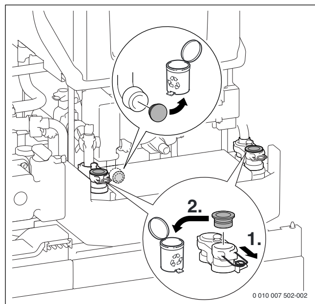
Fig. 43 Retirer le bouchon sur le corps de chauffe et l'échangeur à plaques
