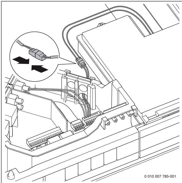
Fig. 56 Raccorder le tiroir du régulateur au boîtier de raccordement
