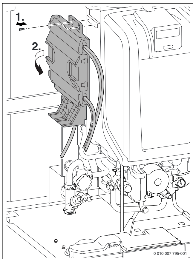
Fig. 50 Retirer l'appareil de commande
