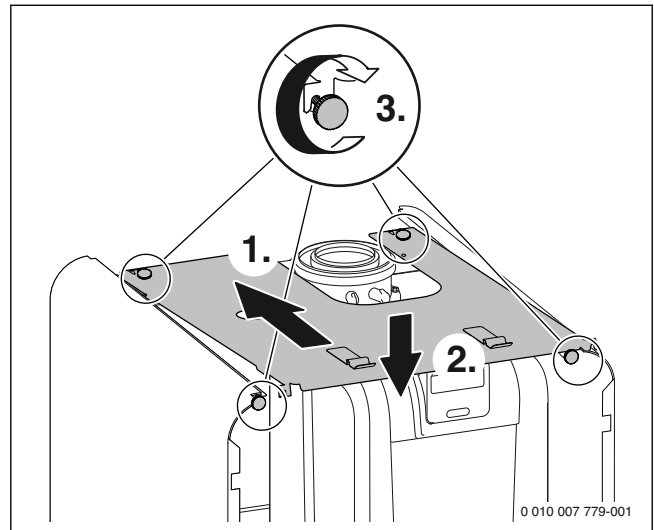
Fig. 72 Glisser le carénage supérieur vers l'arrière et fixer à l'avant et l'arrière avec les 4 vis
