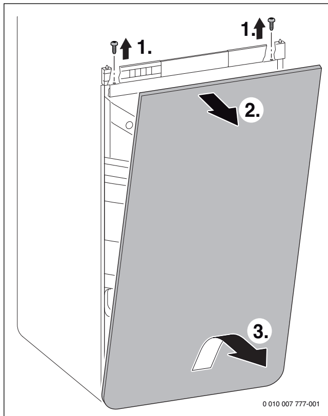
Fig. 40 Retirer le carénage avant du ballon
