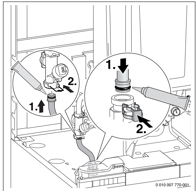
Fig. 48 Raccorder le tube raccord entre la vanne à 3 voies et le départ du ballon
