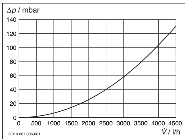
Fig. 106 Diagramme pertes de pression circuit de chauffage sans mélangeur (HK1)
