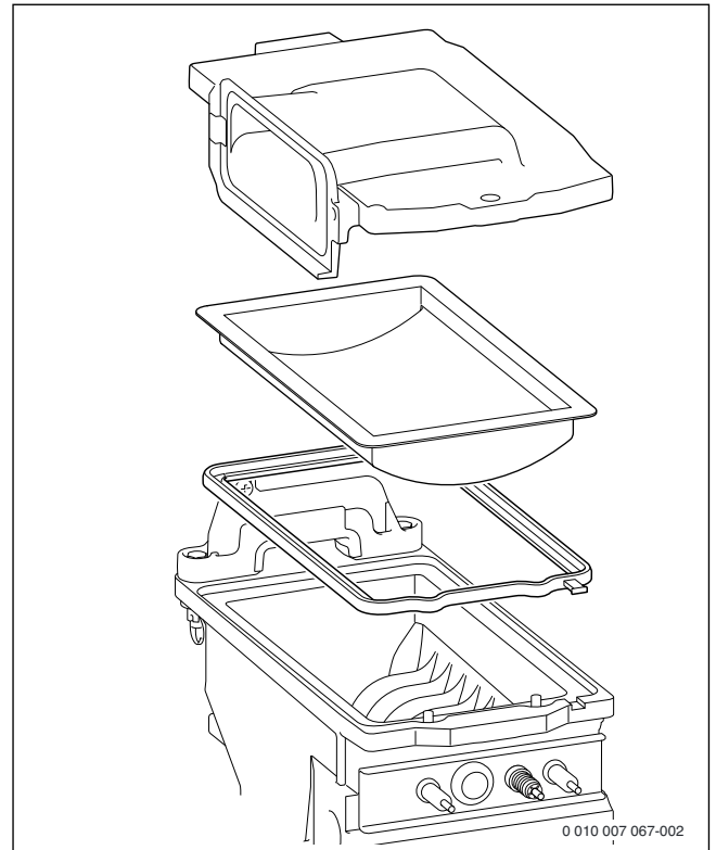
Fig. 86 Brûleur
