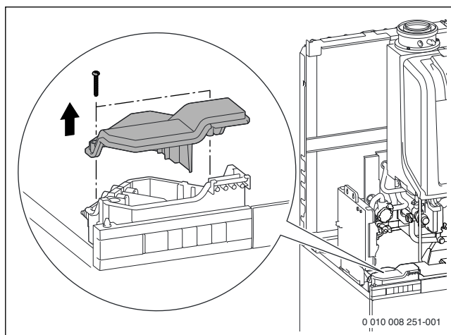
Fig. 60 Retirer le couvercle du boîtier de raccordement
