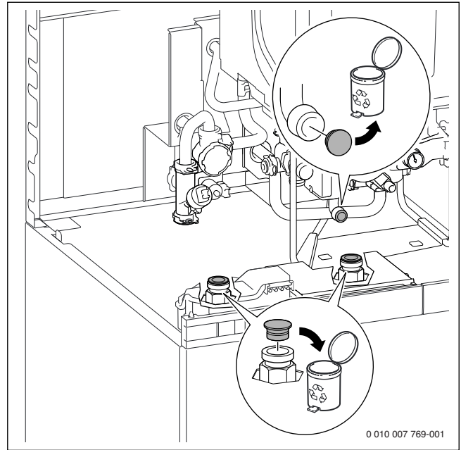
Fig. 47 Retirer le bouchon sur le bloc thermique et sur le départ et retour du ballon
