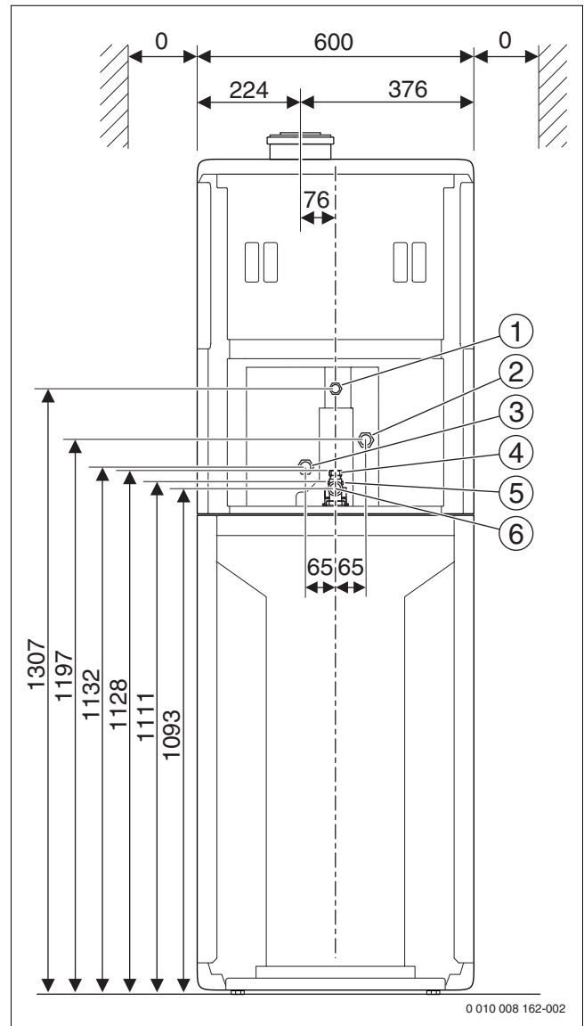
Fig. 3 Dimensions et raccordements sans accessoires (dimensions en mm) (distance recommandée par rapport au mur \geq 50 mm)
