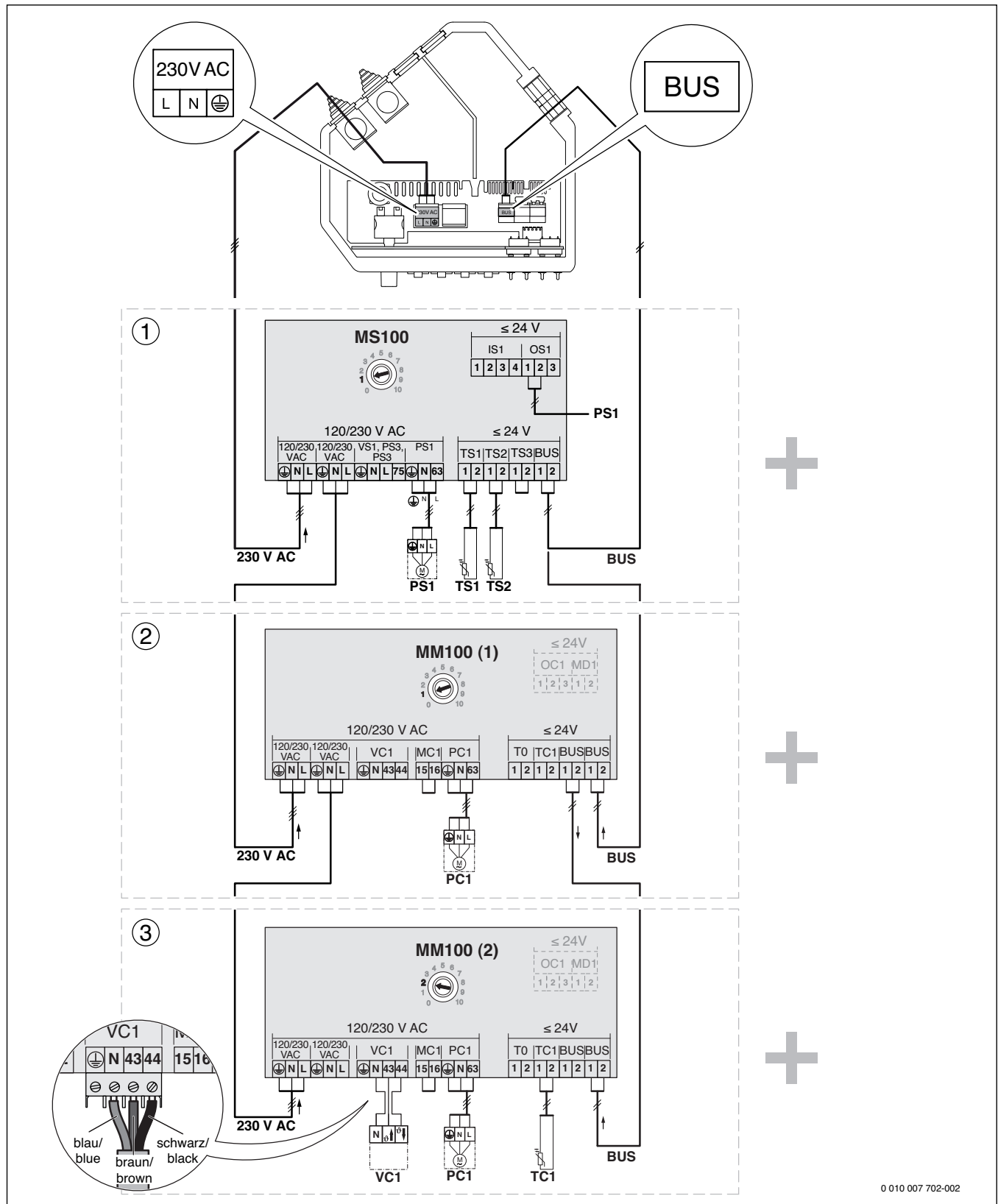
Fig. 63 Raccordement des modules MS 100 et MM 100, si existants
