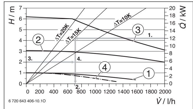
Fig. 110 Courbes caractéristiques de la pompe
