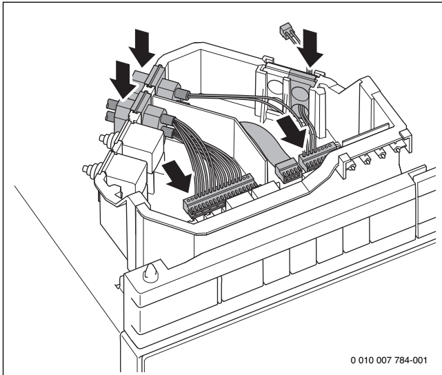
Fig. 54 Raccorder l'appareil de commande au boîtier de raccordement
