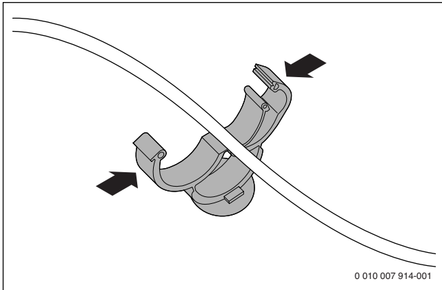
Fig. 55 Fixer le câble avec les clips
