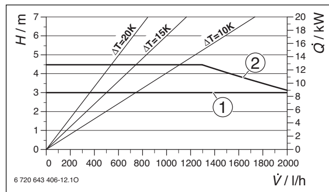
Fig. 114 Courbes caractéristiques de la pompe
