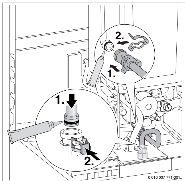
Fig. 49 Raccorder le tube raccord entre le retour du ballon et le bloc thermique
