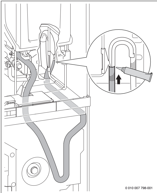
Fig. 46 Insérer le tube siphon sur l'élément d'extrémité
