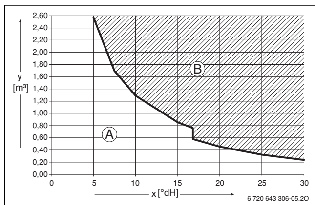
Fig. 35 Conditions requises pour l'eau de remplissage et d'appoint sur les appareils < 50 kW
