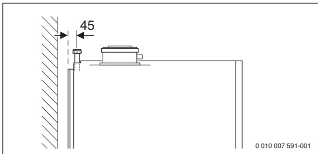
Fig. 13 Dimensions de raccordement de l'accessoire CS 14 - Kit de raccordement soutien chauffage (en mm)
