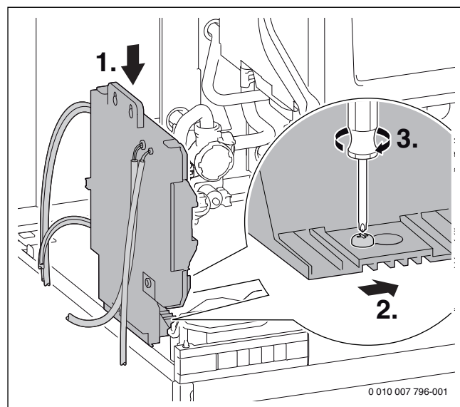
Fig. 51 Fixer l'appareil de commande sur le ballon
