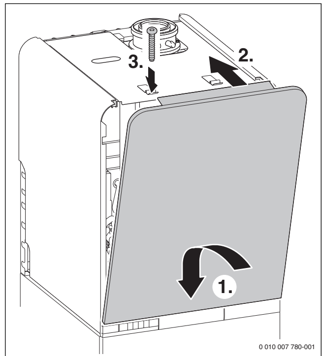
Fig. 73 Suspending le carénage avant et fixer à l'aide de la vis fournie
