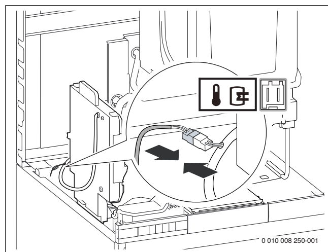
Fig. 52 Raccorder la sonde de température ballon
