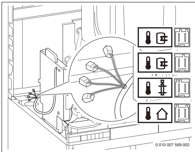
Fig. 64 Connecteur sur le boîtier de commande
