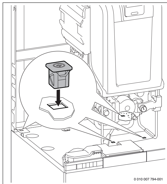
Fig. 43 Fixer l'appareil sur le ballon avec les 4 clips joints
