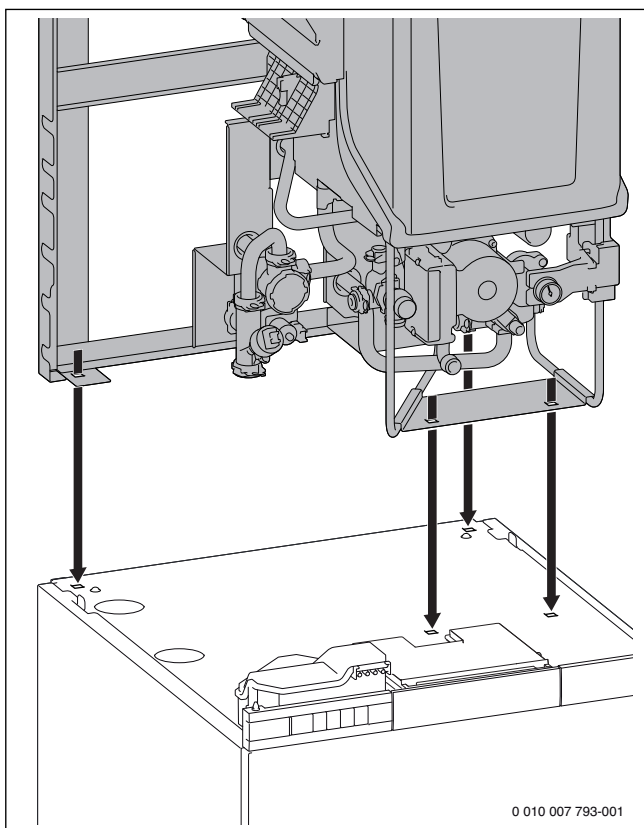
Fig. 42 Placer l'appareil sur le ballon
