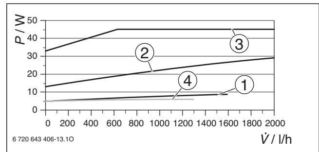
Fig. 111 Puissance absorbée
