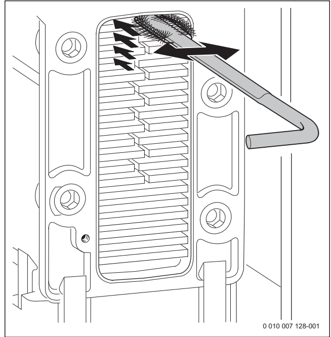
Fig. 90 Nettoyer l'échangeur de chaleur à l'aide de la brosse
