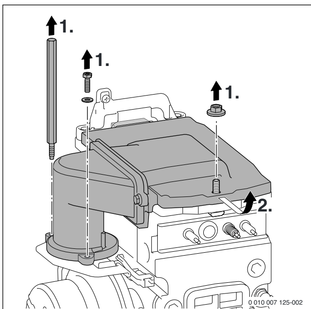
Fig. 85 Détacher le couvercle du brûleur
