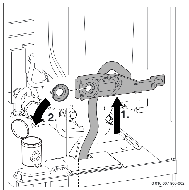
Fig. 44 Retirer le filtre de la position d'entretien et retirer le couvercle de protection
