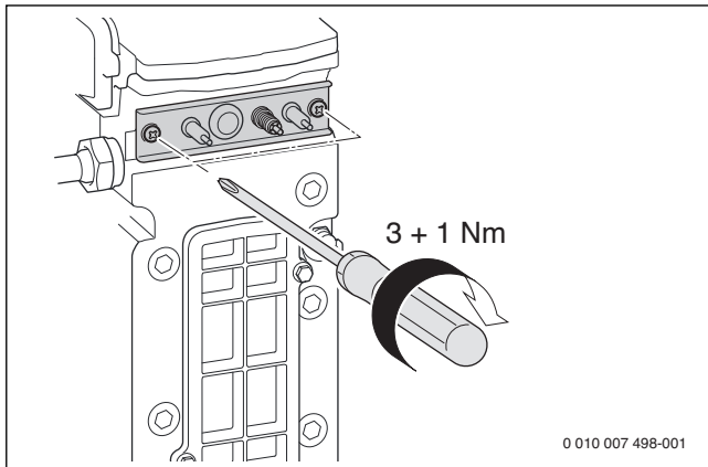
Fig. 83 Remonter le jeu d'électrodes
