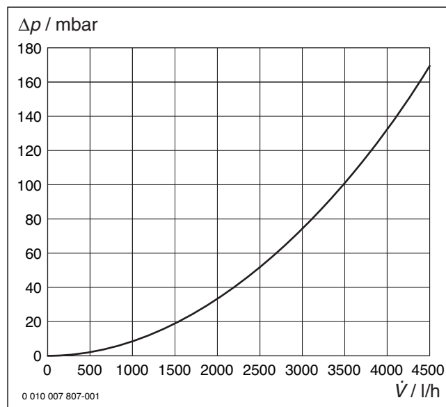
Fig. 107 Diagramme pertes de pression circuit avec mélangeur (HK2)
