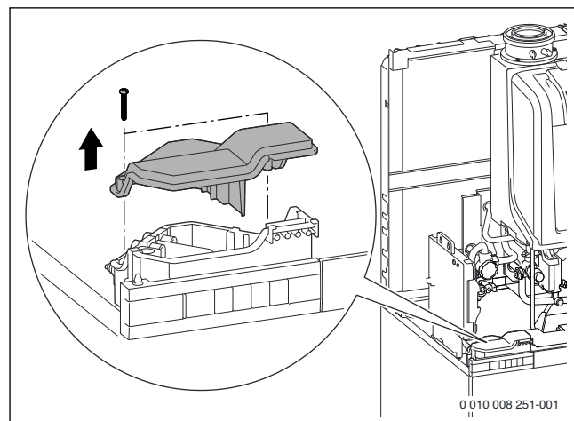
Fig. 53 Retirer le couvercle du boîtier de raccordement
