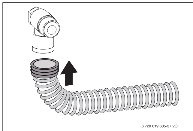
Fig. 37 Monter le flexible sur la soupape de sécurité
