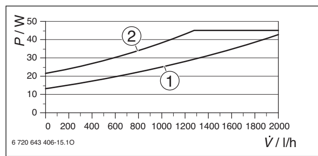
Fig. 115 Puissance absorbée
