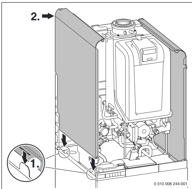
Fig. 71 Monter le carénage droit et gauche
