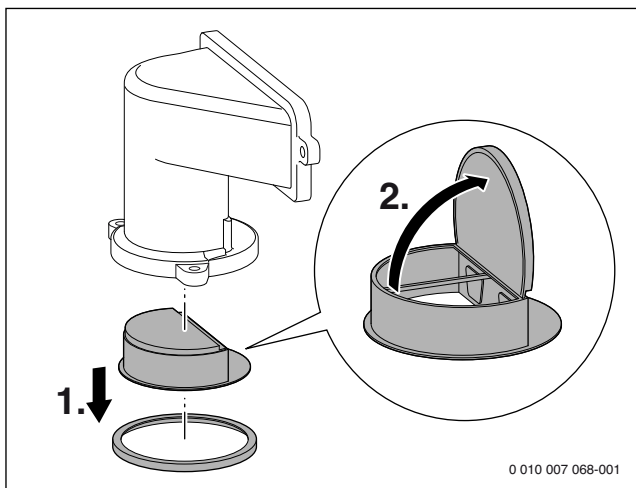
Fig. 96 Clapet anti-retour du dispositif de mélange
