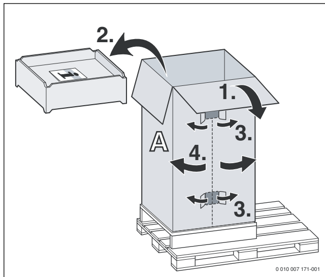
Fig. 39 Déballer le ballon
