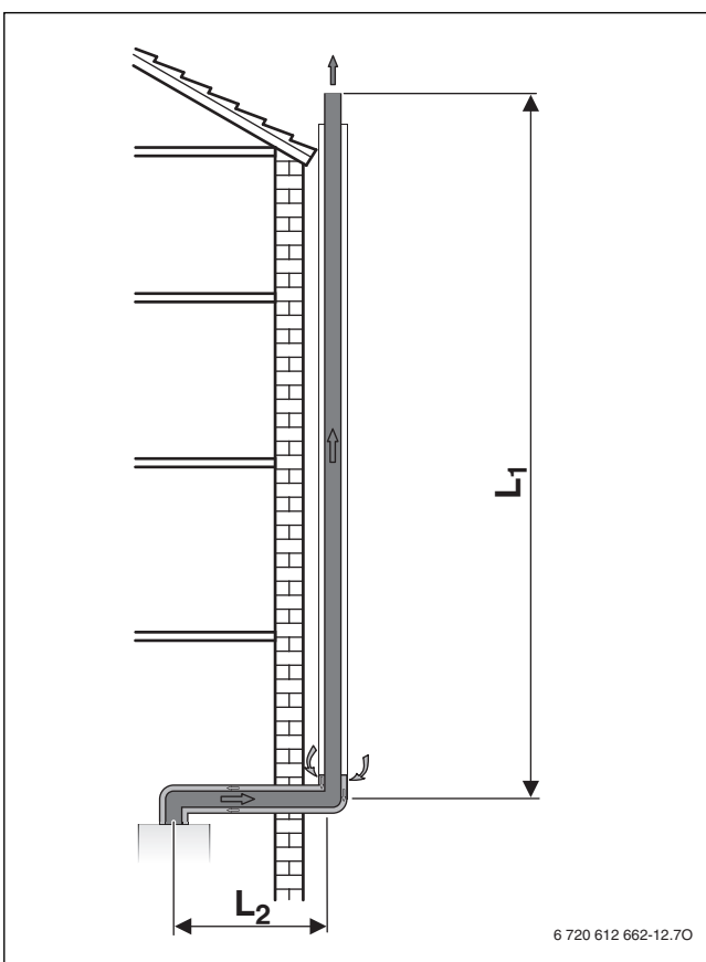
Fig. 30 Evacuation des fumées sur la façade selon C 53
