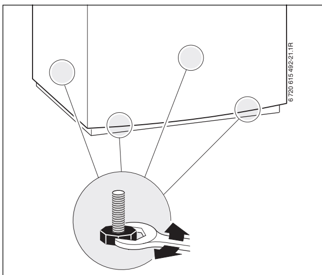
Fig. 41 Positionner le ballon
