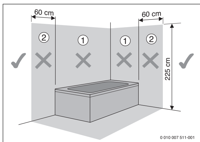
Fig. 59 Zones de protection
