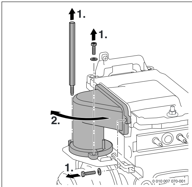
Fig. 95 Démontez le dispositif de mélange
