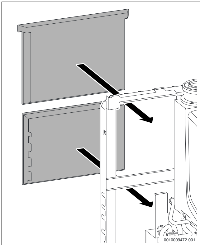
Fig. 70 Montage des isolations thermiques à l'arrière
