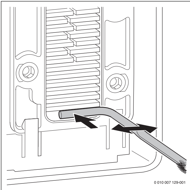
Fig. 92 Nettoyer le bac des condensats
