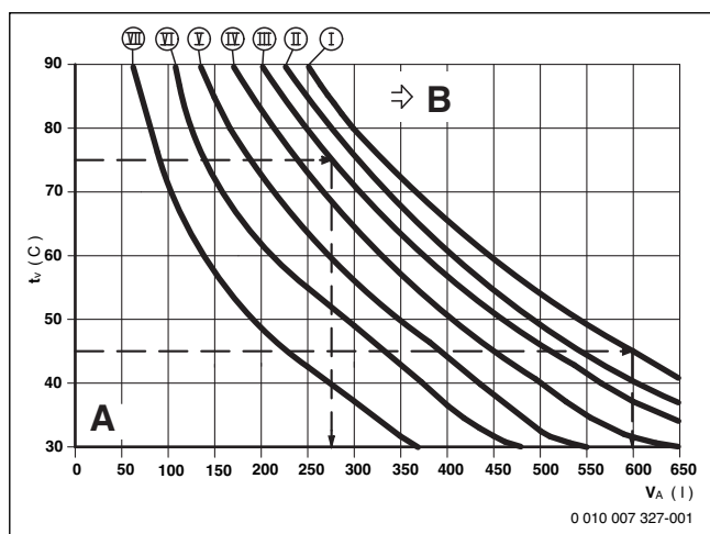
Fig. 36 Courbes caractéristiques du vase d'expansion 18 l
