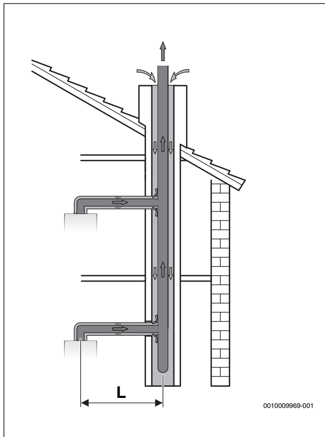
Fig. 32 Affectation multiple avec tube concentrique selon C 43
