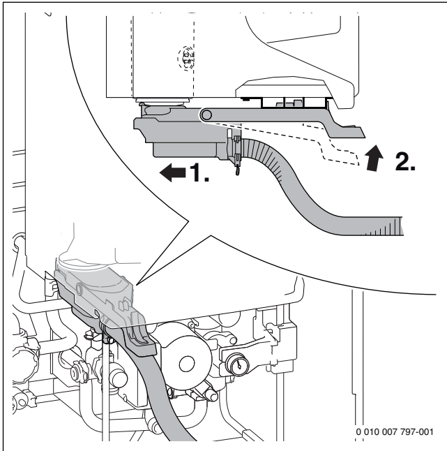
Fig. 45 Monter le filtre
