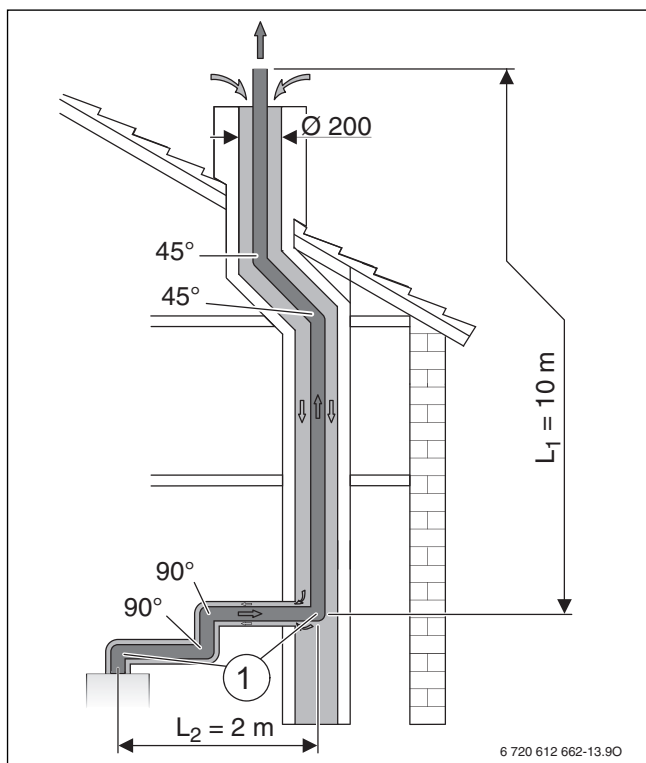
Fig. 31 Situation de montage d'un système d'évacuation des fumées selon C 93
