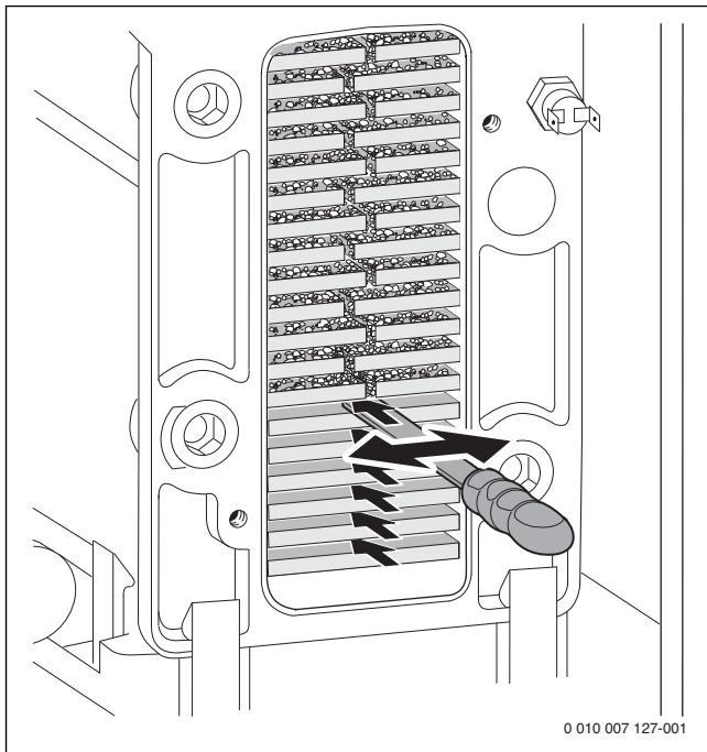
Fig. 89 lame de nettoyage
