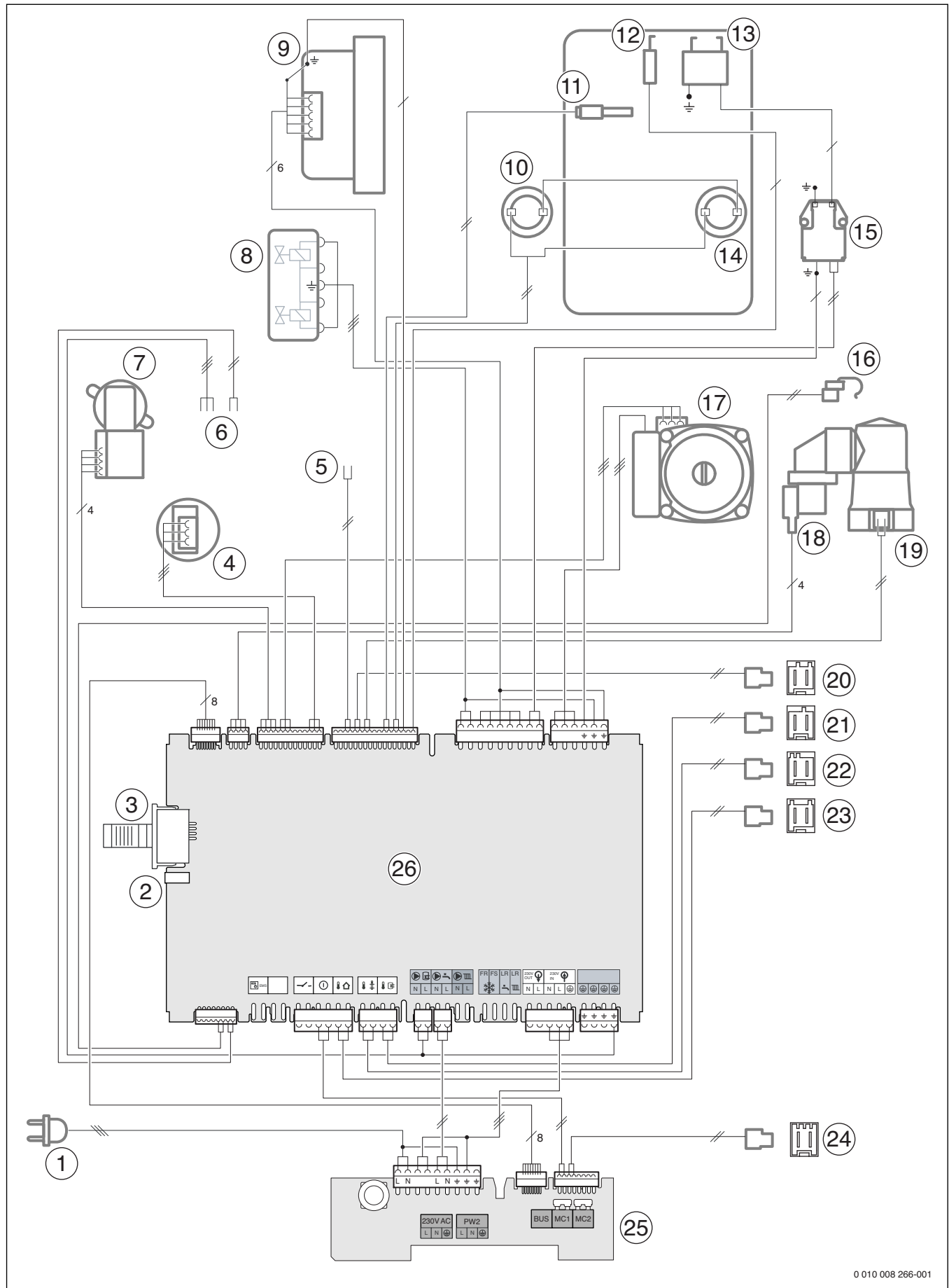
Fig. 104 Câblage électrique
