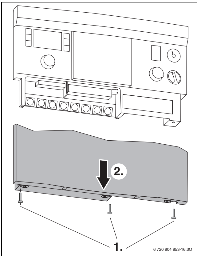
Bild 74 Abdeckung entfernen
