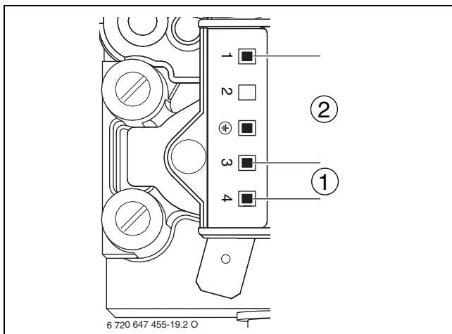
Bild 70 Messstellen an der Gasarmatur
