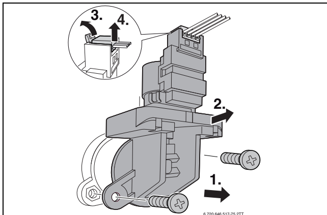
Bild 69 3-Wege-Ventil ausbauen
