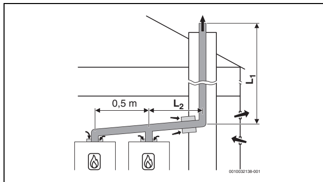
Bild 27 Kaskade mit 2 Geräten: Starre Abgasführung im Schacht nach B 23p /B 53p mit raumluftabhängiger Luftzufuhr am Gerät
