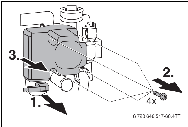
Bild 73 Heizungspumpe ausbauen
