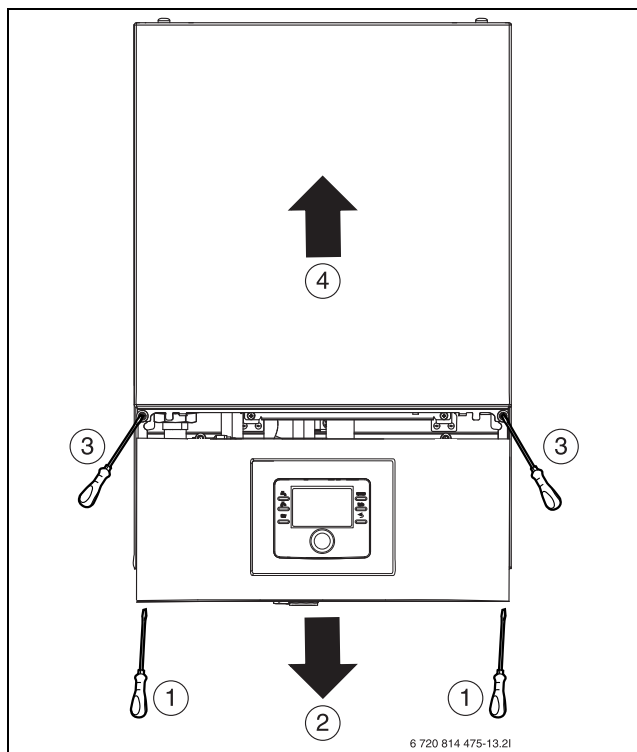
Bild 5 Frontverkleidung abnehmen
