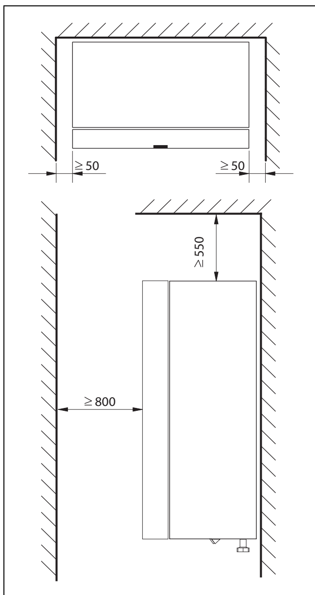
Bild 3 Mindestabstand (mm)
