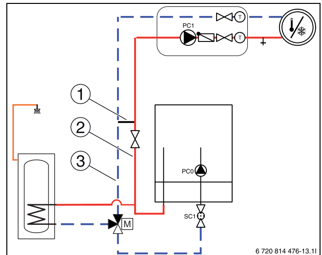
Bild 25 Inneneinheit mit Heizkreis und Warmwasserbereitung
