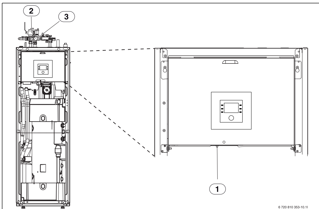
Fig. 5 Unité intérieure AWMS / AWMSS
