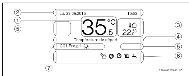
Fig. 4 Symboles sur l'écran principal (exemple)
