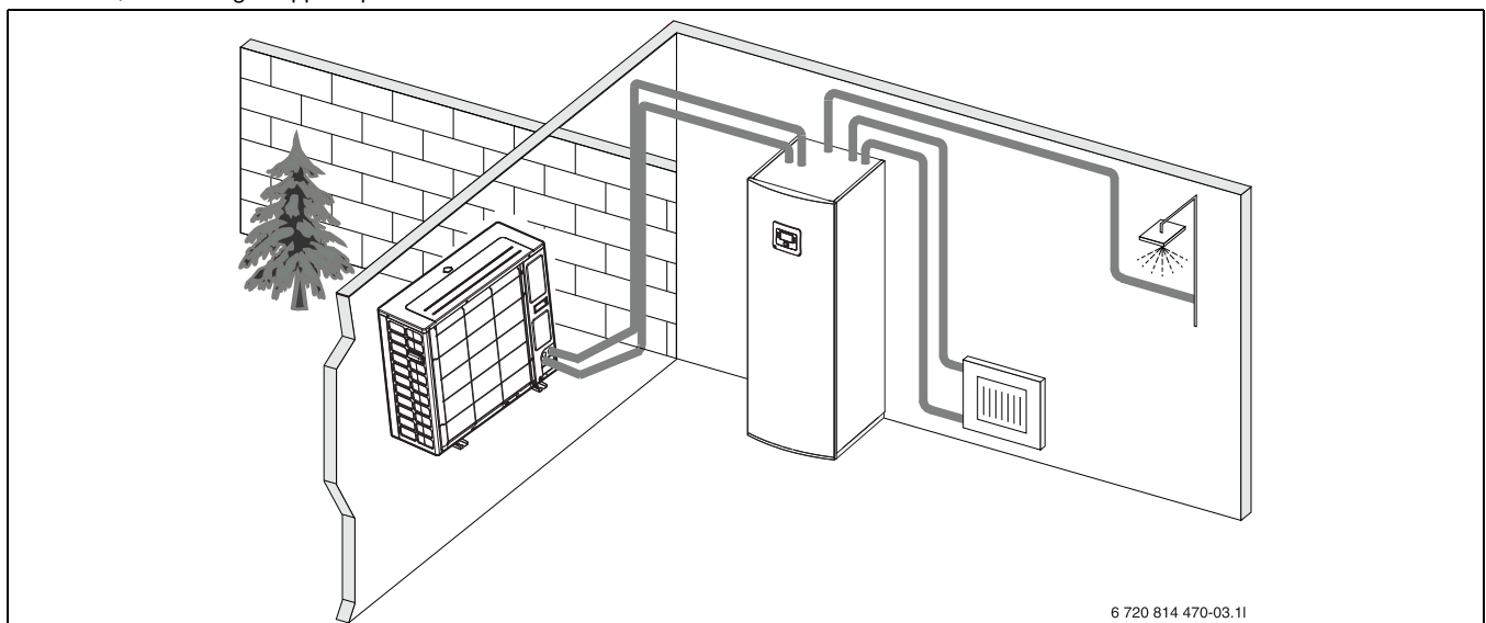
Fig. 2 Pompe à chaleur, unité extérieure, unité intérieure AWMS/AWMS avec ballon d'eau chaude sanitaire et chauffage d'appoint électrique intégrés
