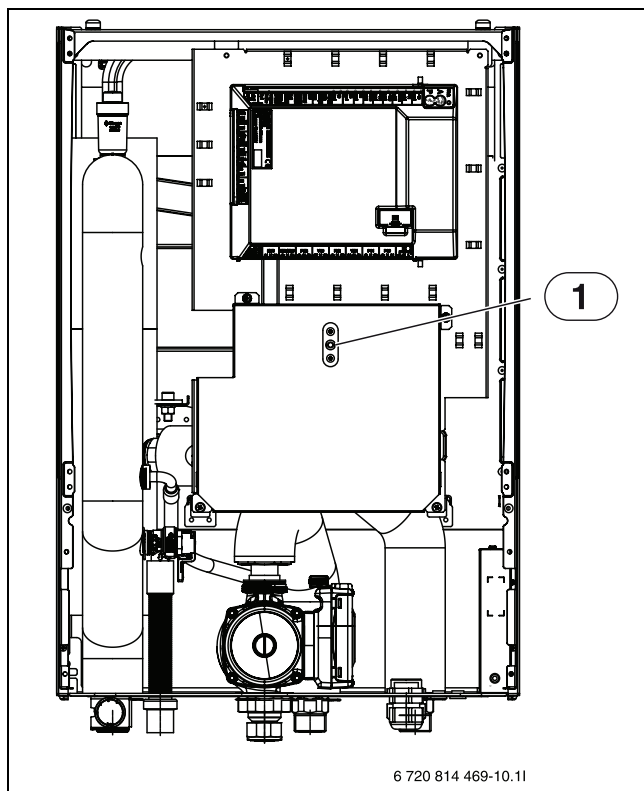
Bild 6 Inneneinheit ASE
