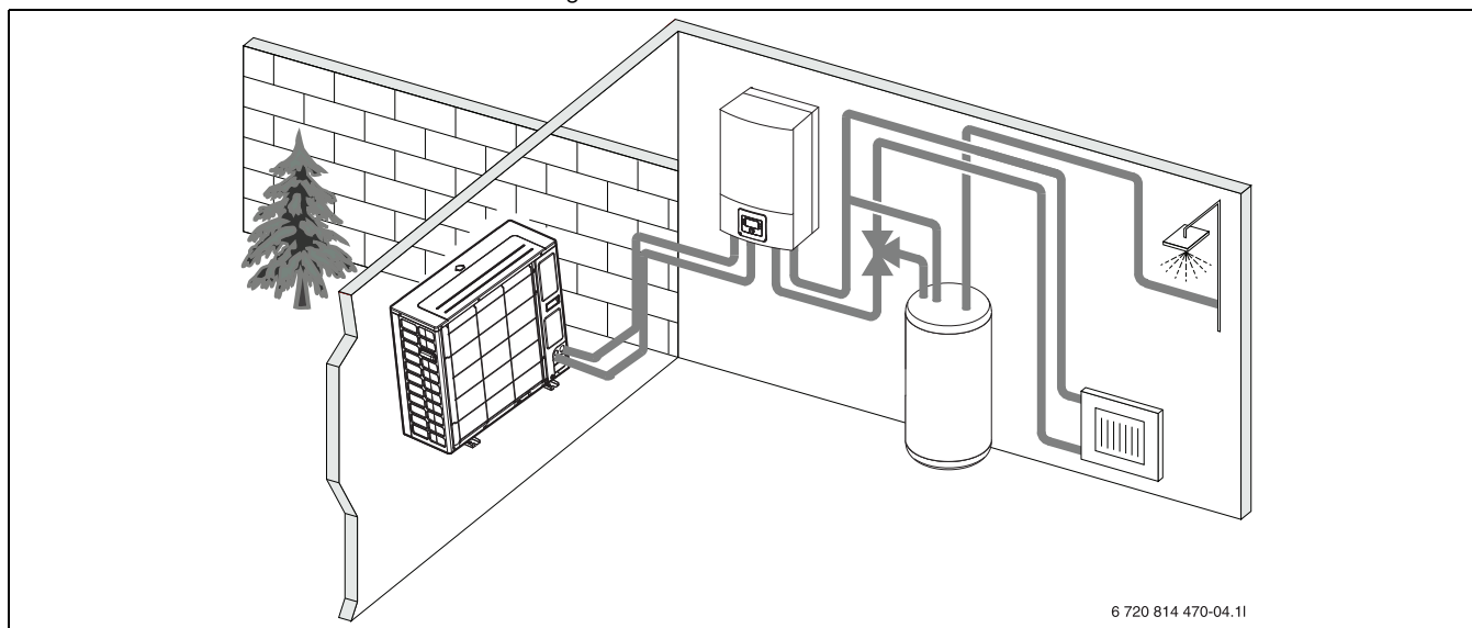
Bild 2 Wärmepumpe Außeneinheit, Inneneinheit ASE mit elektrischem Zuheizter, externer Warmwasserspeicher
