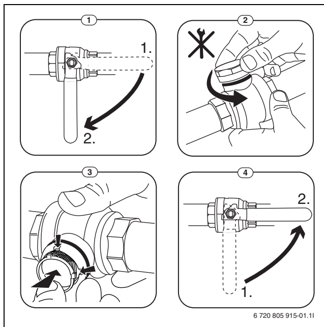
Bild 7 Siebreinigung
