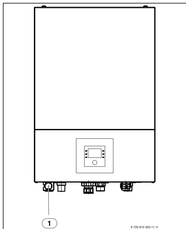
Afb. 5 Binneneenheid AWES
