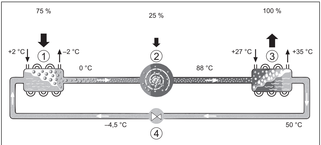
Fig. 1 Principe de fonctionnement du circuit du fluide frigorigère dans la pompe à chaleur
