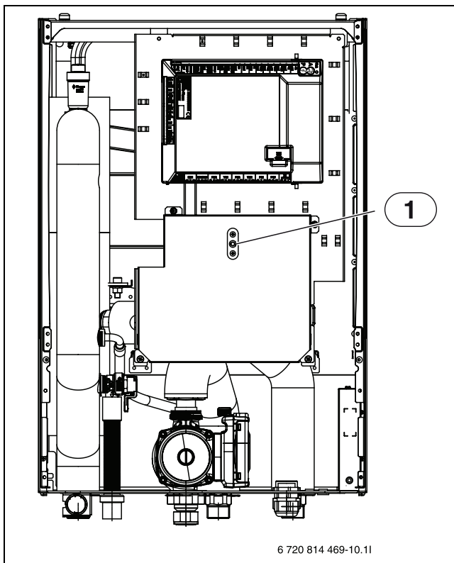
Fig. 6 Unité intérieure AWES
