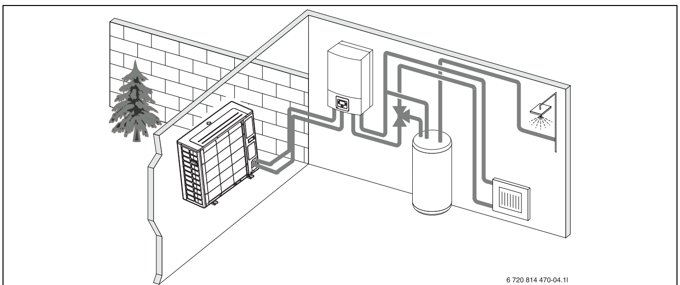
Fig. 2 Pompe à chaleur unité extérieure, unité intérieure AWES avec chauffage d'appoint électrique, ballon d'eau chaude sanitaire externe
